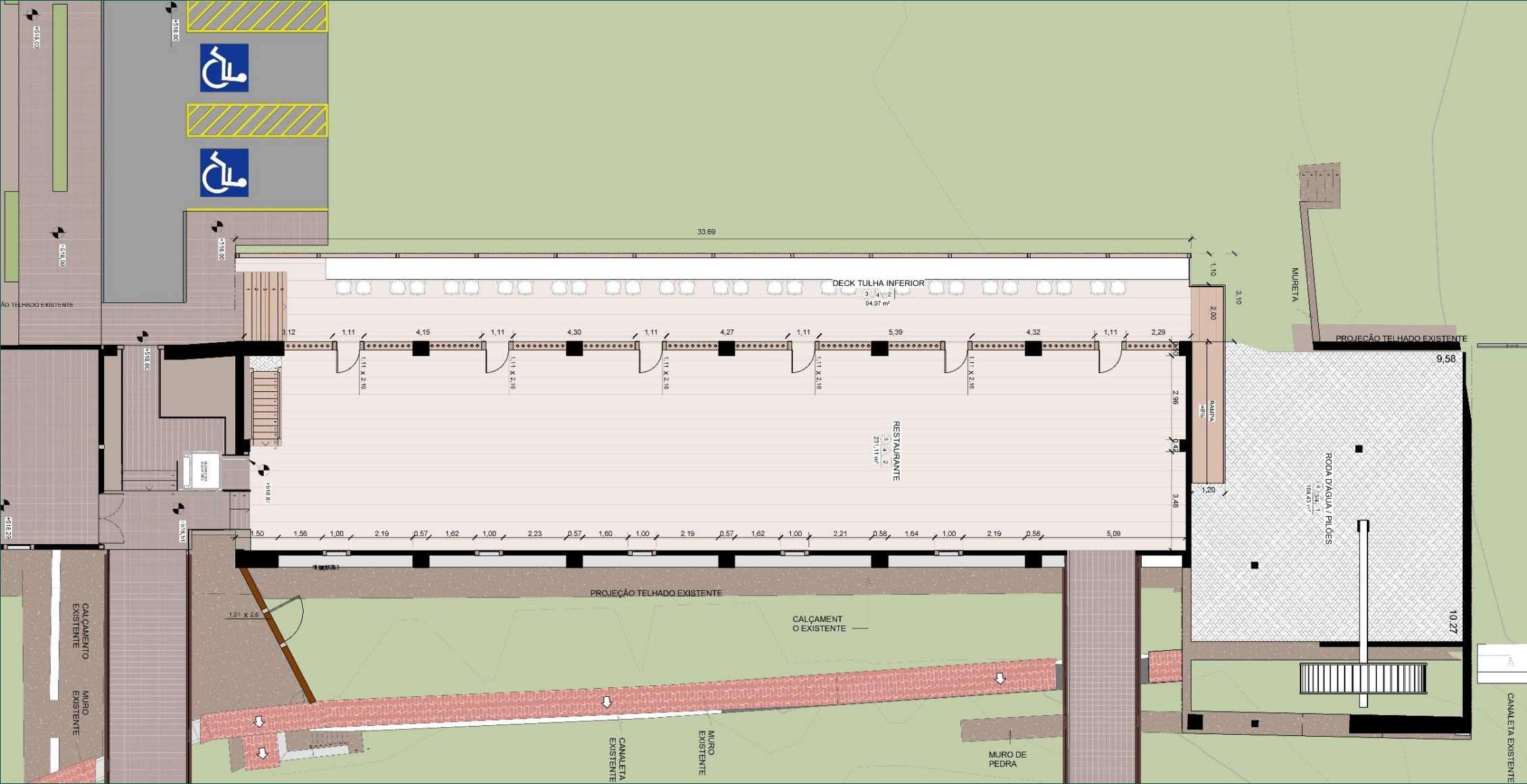
PLANTA – RODA D'ÁGUA / PILÕES / TULHA
