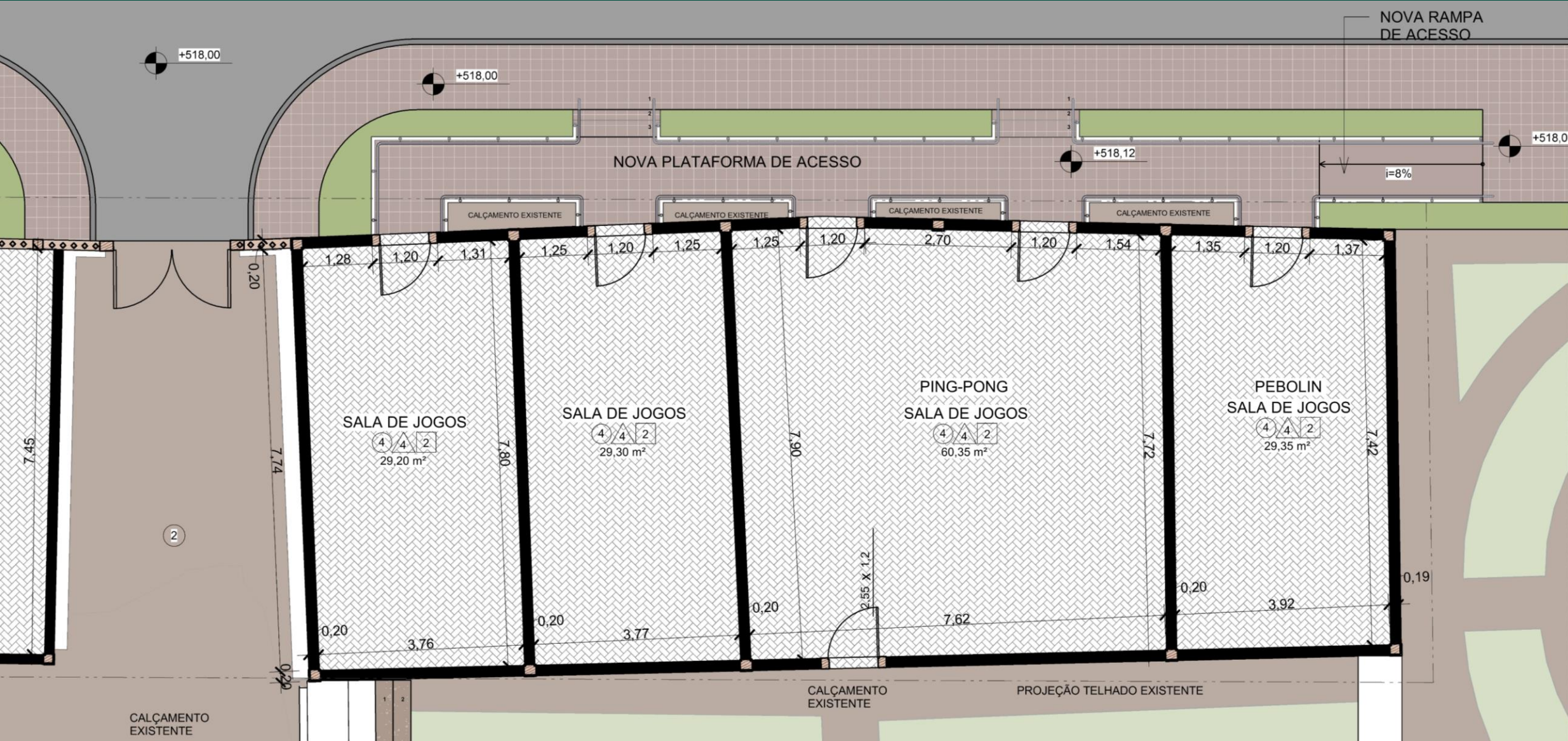
PLANTA – OFICINA N°1
