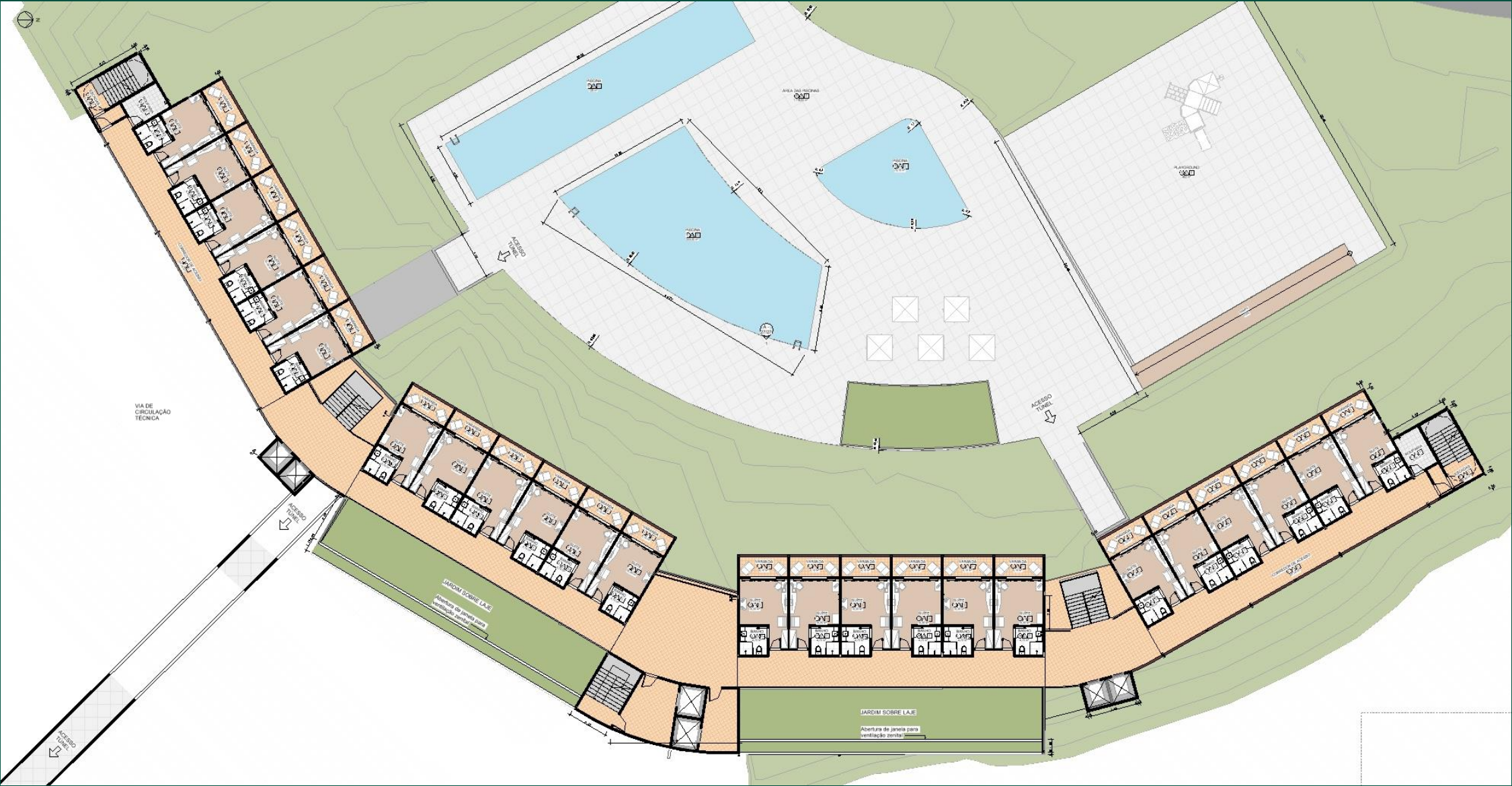
PLANTA – NÍVEL 507
