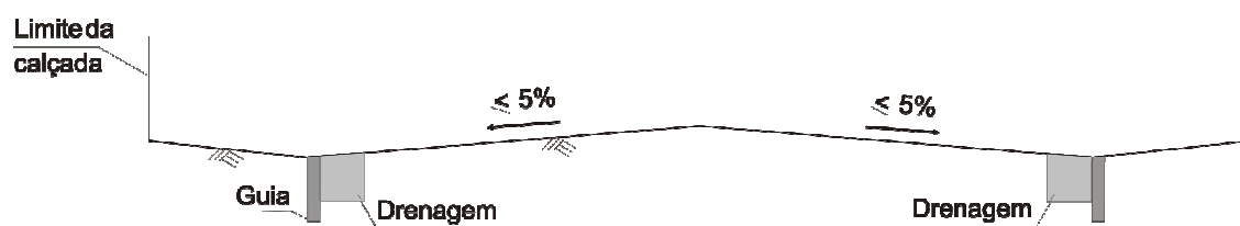
CORTE B-B
