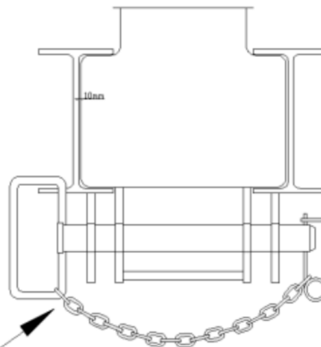
TRAVA LATERAL (DETALHES DA VIGA i)
