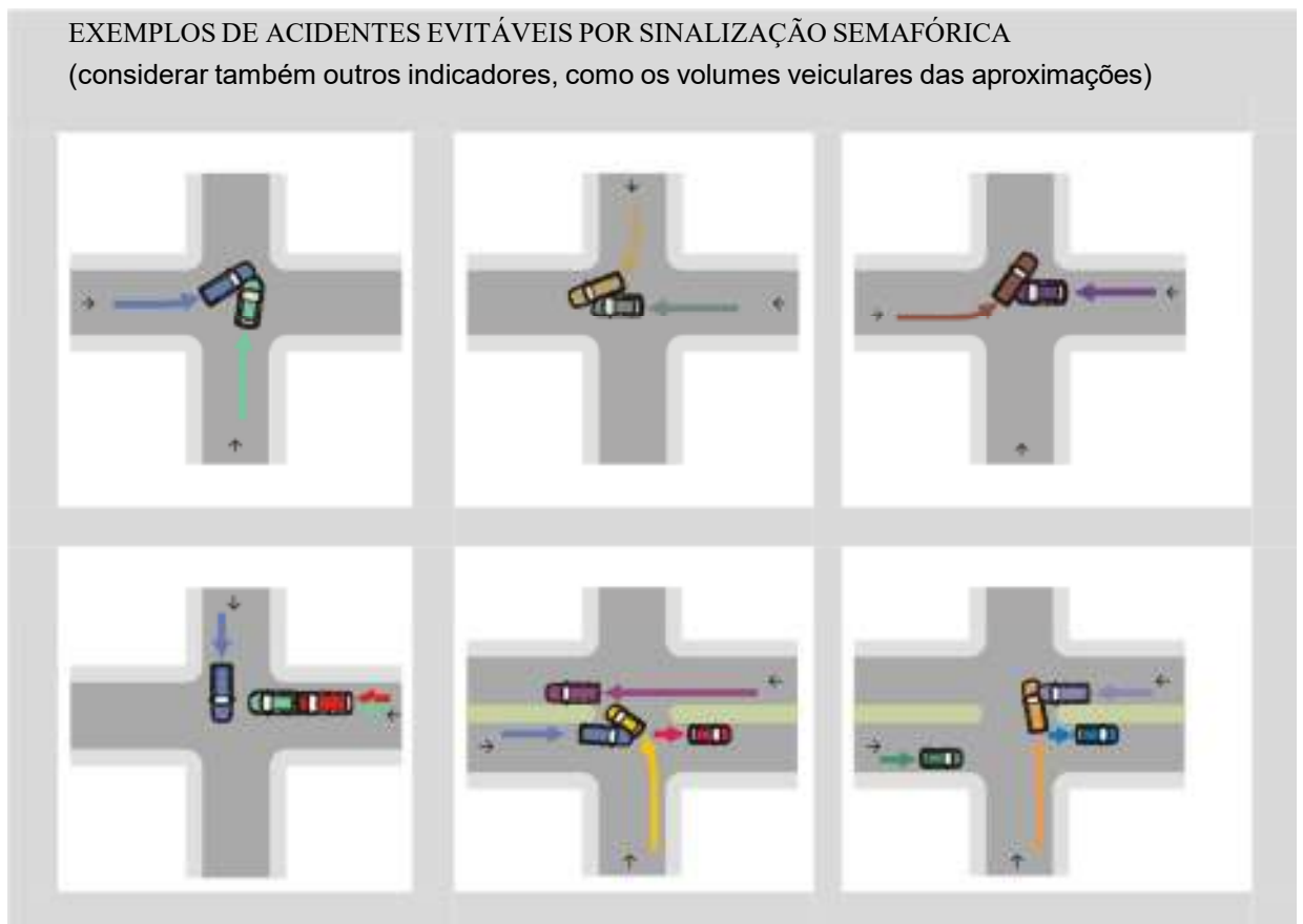
Figura 4.12: Exemplos de acidentes evitáveis por sinalização semafórica
