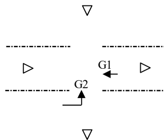
Figura 7.20: Distribuição dos grupos semafóricos
