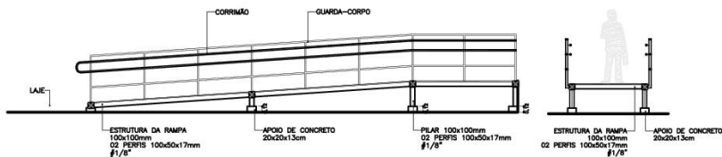
DETALHE D1
