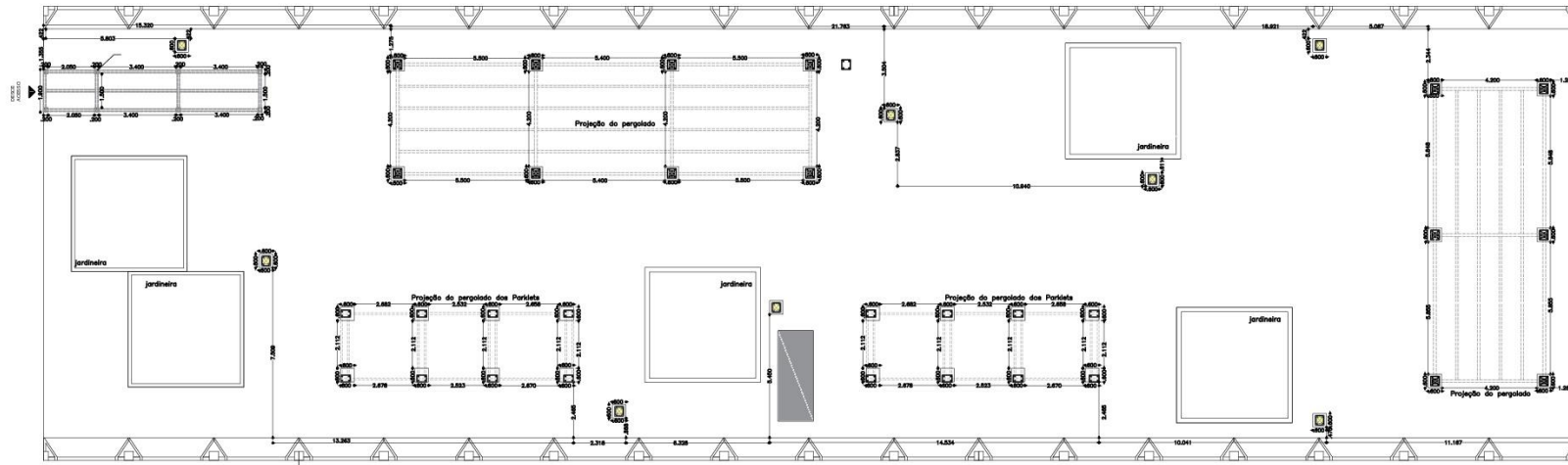
PLANTA DE LOCAÇÃO DE BASES DE CONCRETO
