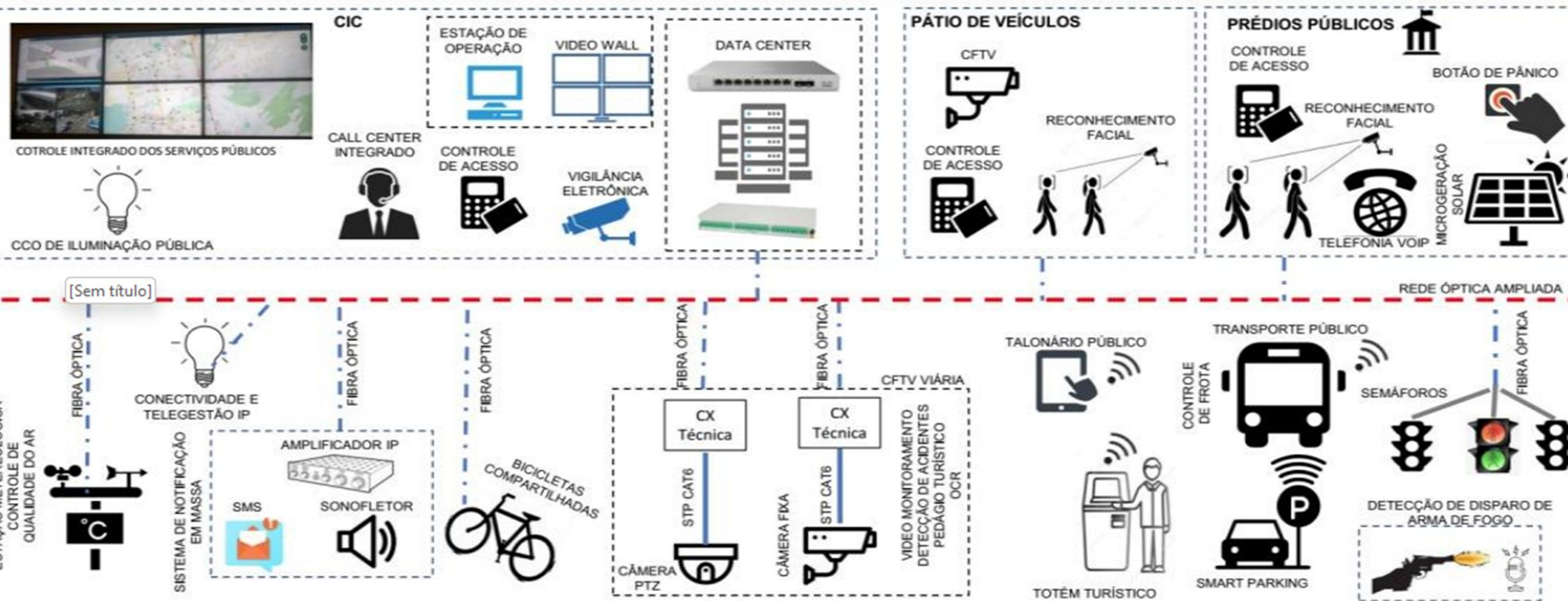
Figura 3 - Arquitetura Esquemática para os serviços digitais Urbanos. Fonte: Omatic (2024)
