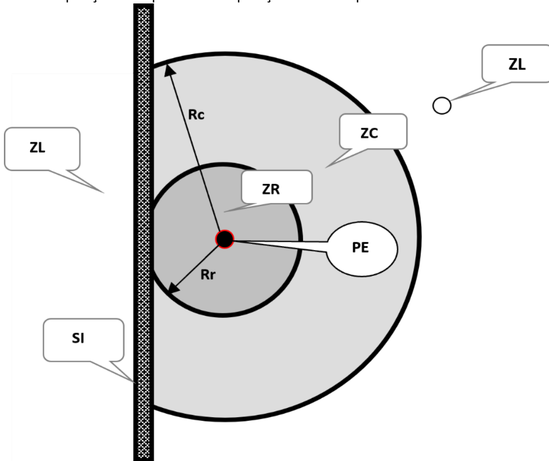
Figura 2 - Distâncias no ar que delimitam radialmente a zona de risco, a zona controlada e a zona livre, com interposição de superfície de separação física adequada.
