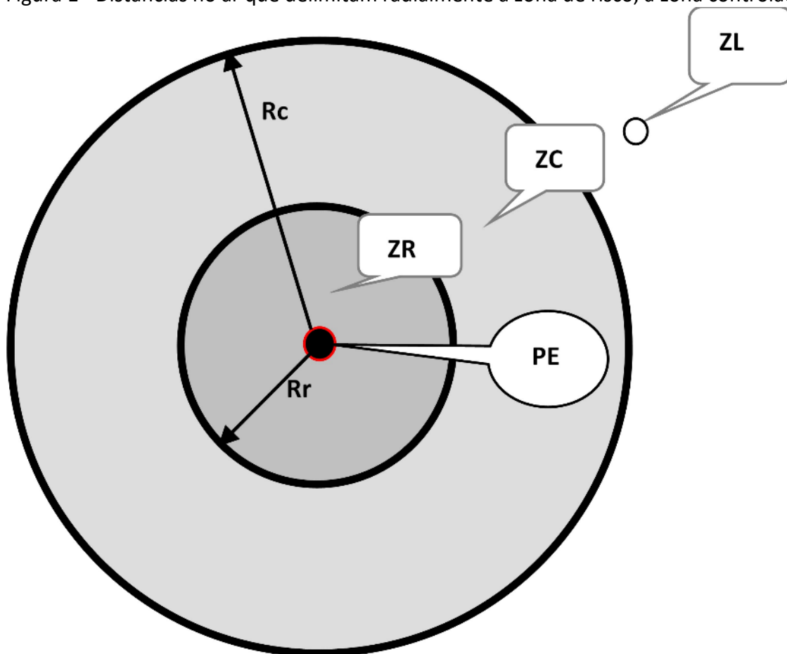
Figura 1 - Distâncias no ar que delimitam radialmente a zona de risco, a zona controlada e a zona livre
