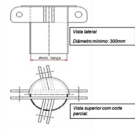
Imagem 1 - Croqui - reforço metálico em lança de madeira
