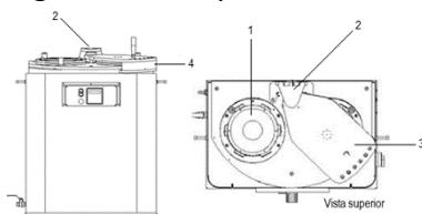
Figura 20: Máquina sorveteira
