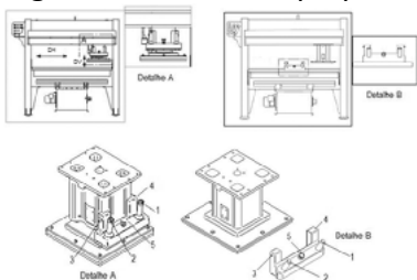
Figura 6: Balancim tipo ponte manual - Vista frontal
