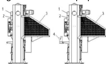
Figura 5: Balancim tipo ponte manual - Vista lateral
