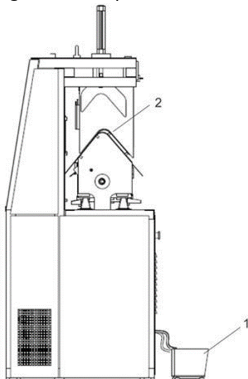
Figura 9: Máquina de cambrê facão - Vista lateral
