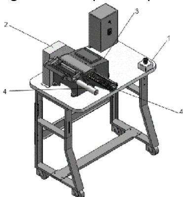
Figura 31: Máquina de passar cola
