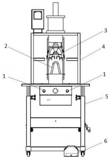
Figura 7: Máquina de cambrê com borrachão - Vista Frontal
