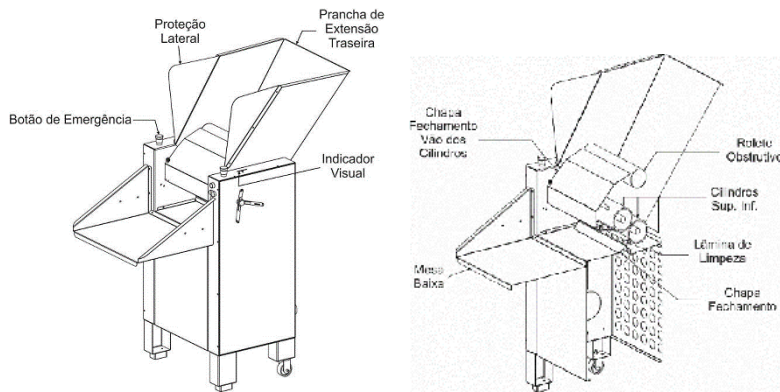
Figura 1: Representação esquemática do cilindro soador.
