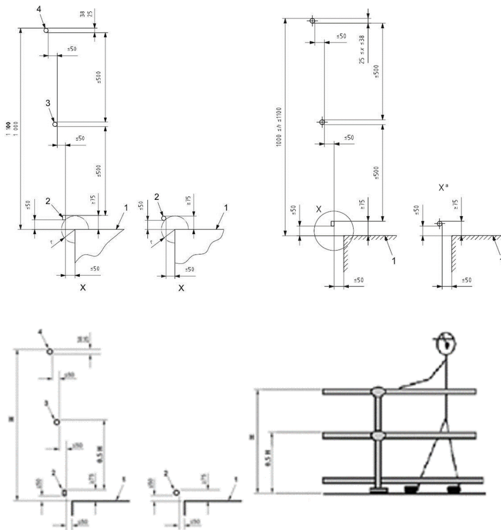
Figura 3: Sistema de proteção contra quedas em plataforma. (dimensões em milímetros)
