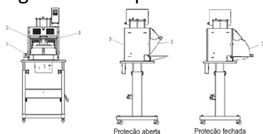
Figura 27: Máquina de dublar ou unir componentes de calçados - Vista frontal e lateral
