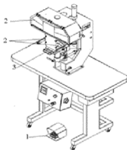
Figura 30: Máquina de carimbar solas e palmilhas
