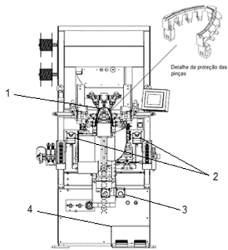
Figura 17: Máquina de montar bicos
