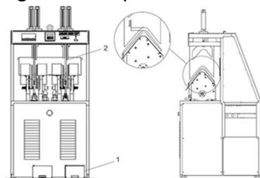
Figura 8: Máquina de cambrê facão - Vista frontal
