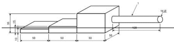
Figura 3 – Gabarito de teste
