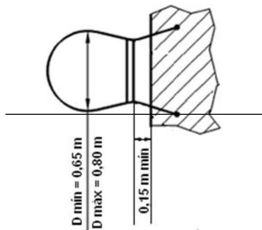
Figura 4: Exemplo de detalhe da gaiola da escada fixa do tipo marinheiro.
