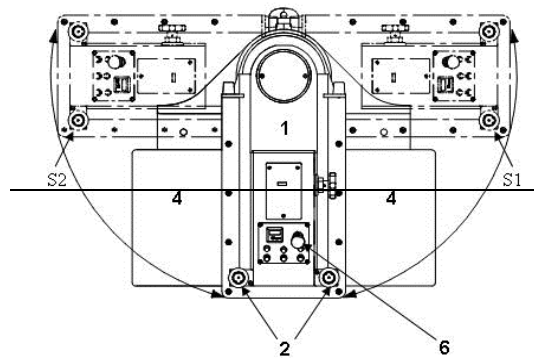
Figura 2 – Balancim de braço móvel manual ou balancim jacaré. Vista de topo – Posição de giro do braço 180° (cento e oitenta graus)
