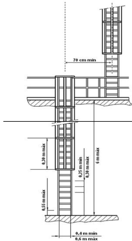
Figura 3: Exemplo de escada fixa do tipo marinheiro.
