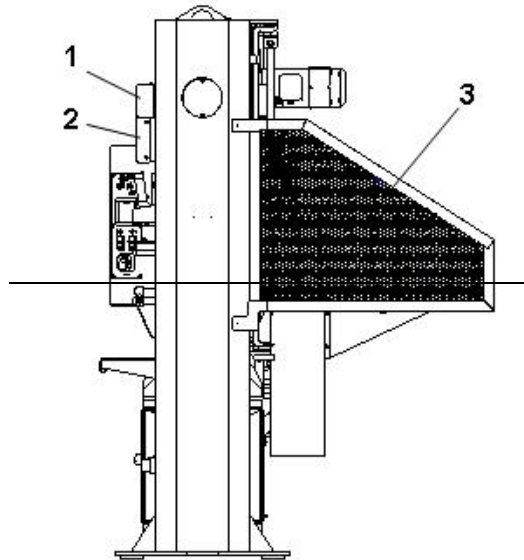
Figura 3 — Balancim do tipo ponte manual. Vista lateral
