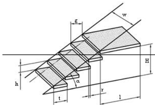
Figura 2: Exemplo de escada sem espelho.
