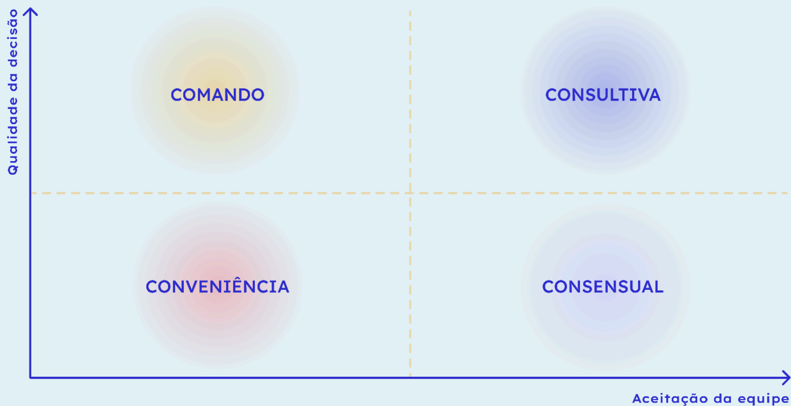
Matriz 4 estilos de tomada de decisão
