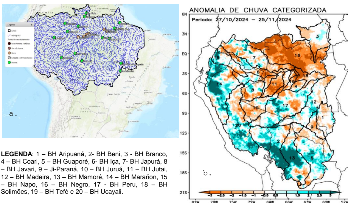
Figura 3. Monitoramento da bacia do rio Amazonas (a.) e anomalia de chuva no período de 27/10 a 25/11 de 2024.
