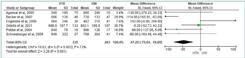
Figura 12 - Gráfico de floresta das soluções de preservação HTK vs. UW no tempo de isquemia do enxerto pancreático
