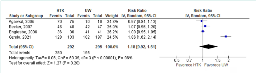
Figura 10 - Gráfico de floresta das soluções de preservação HTK vs. UW na sobrevida do paciente no transplante pancreático
