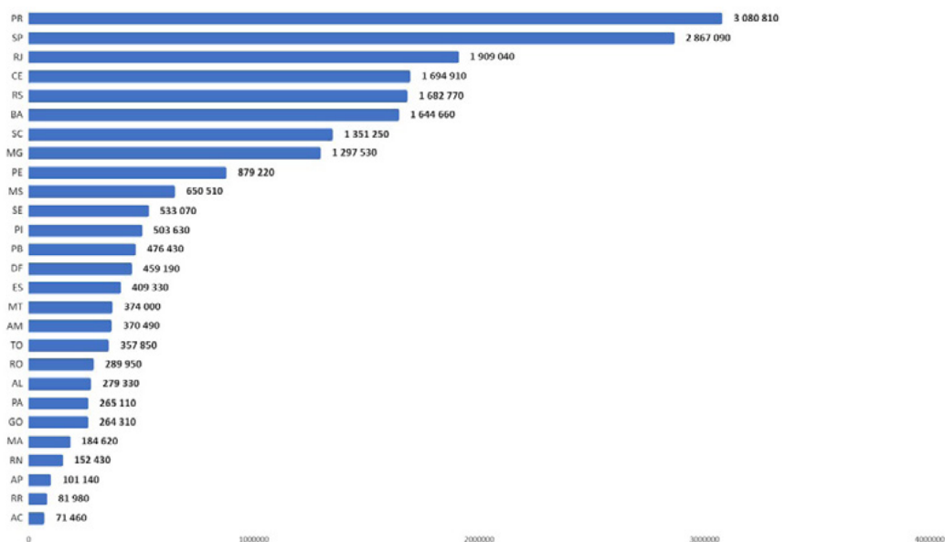
FIGURA 5 Total de tubos de coleta de amostras suspeitas de covid-19 distribuídos por UF, Brasil, 5 de março de 2020 até 12 de novembro de 2022
