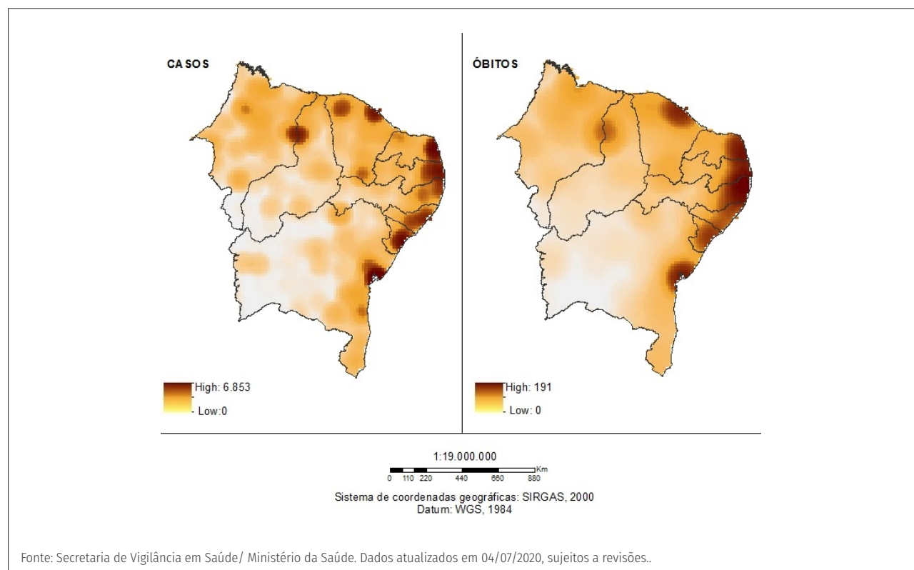
FIGURA 25 Ocorrência de novos registros de casos e óbitos de COVID-19 na Região Nordeste do Brasil na Semana Epidemiológica 27, observando-se a densidade por método Kernel
