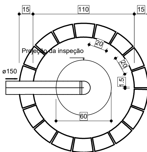
Sumidouro - Pavimento Planta baixa - ESC. 1:100
