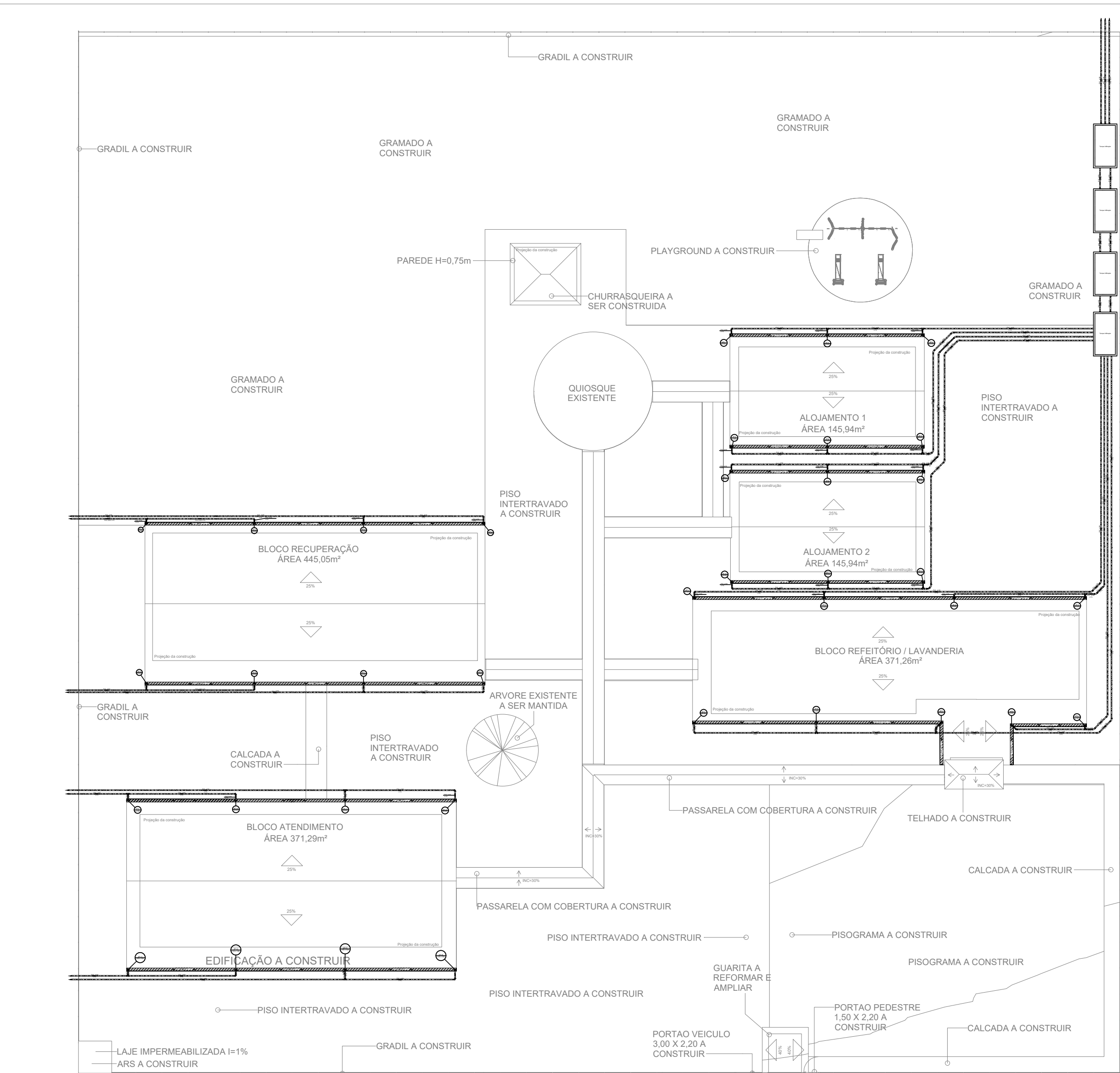
DETALHAMENTO ESGOTAMENTO PLUVIAL - CASA CANARANA ESC - 1/350
