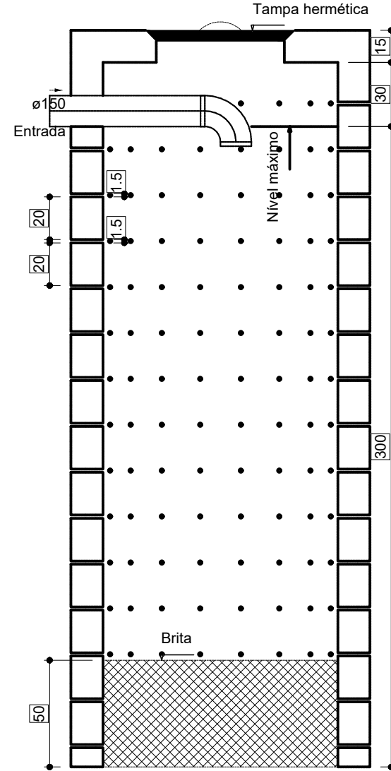
Sumidouro - Pavimento Corte 1 - ESC. 1:100
