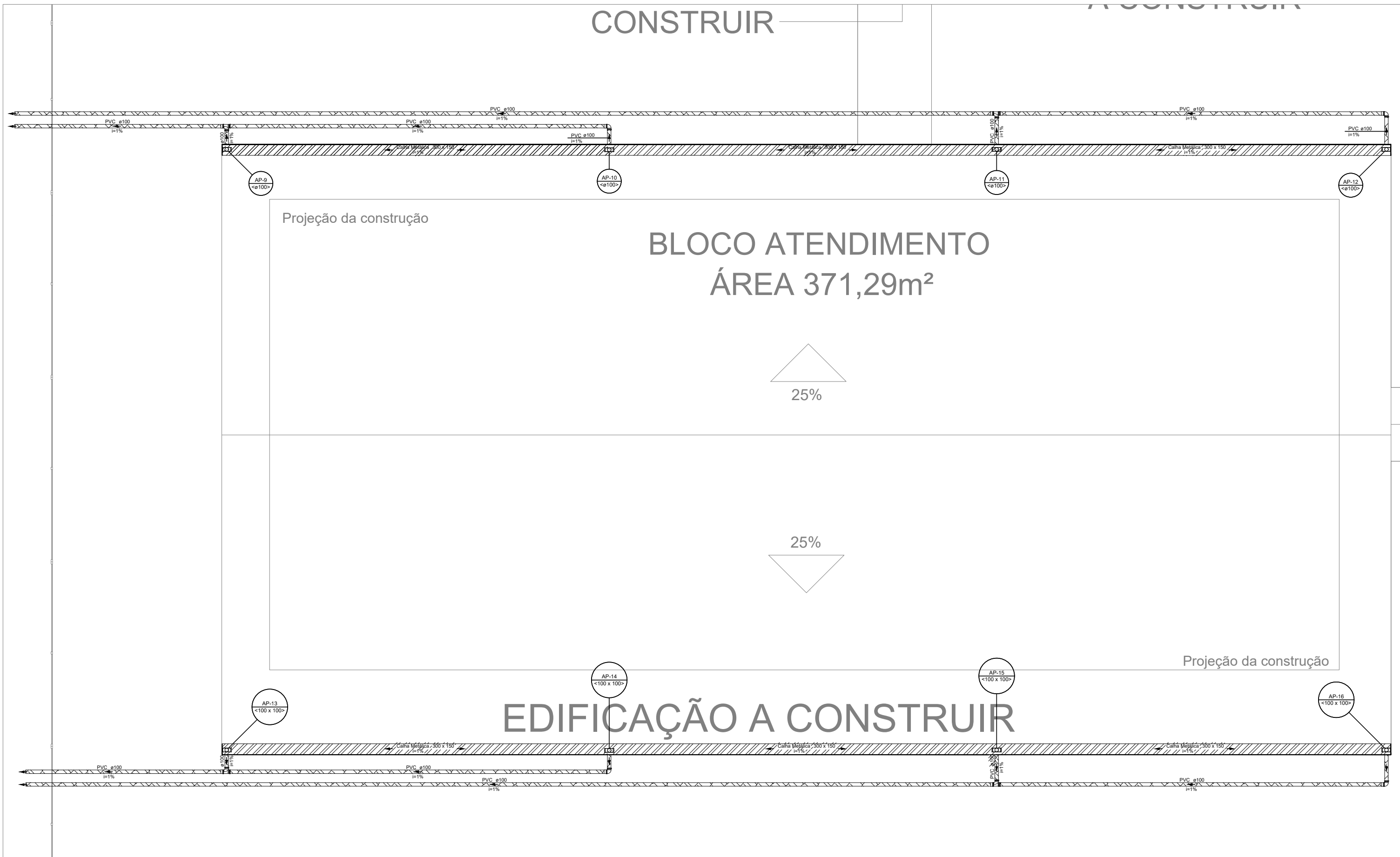
DETALHAMENTO ESGOTAMENTO PLUVIAL - BLOCO DE ATENDIMENTO ESC - 1/100
