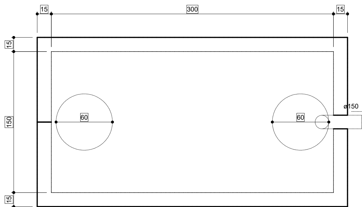
Tanque séptico - Pavimento Planta baixa - ESC. 1:100
