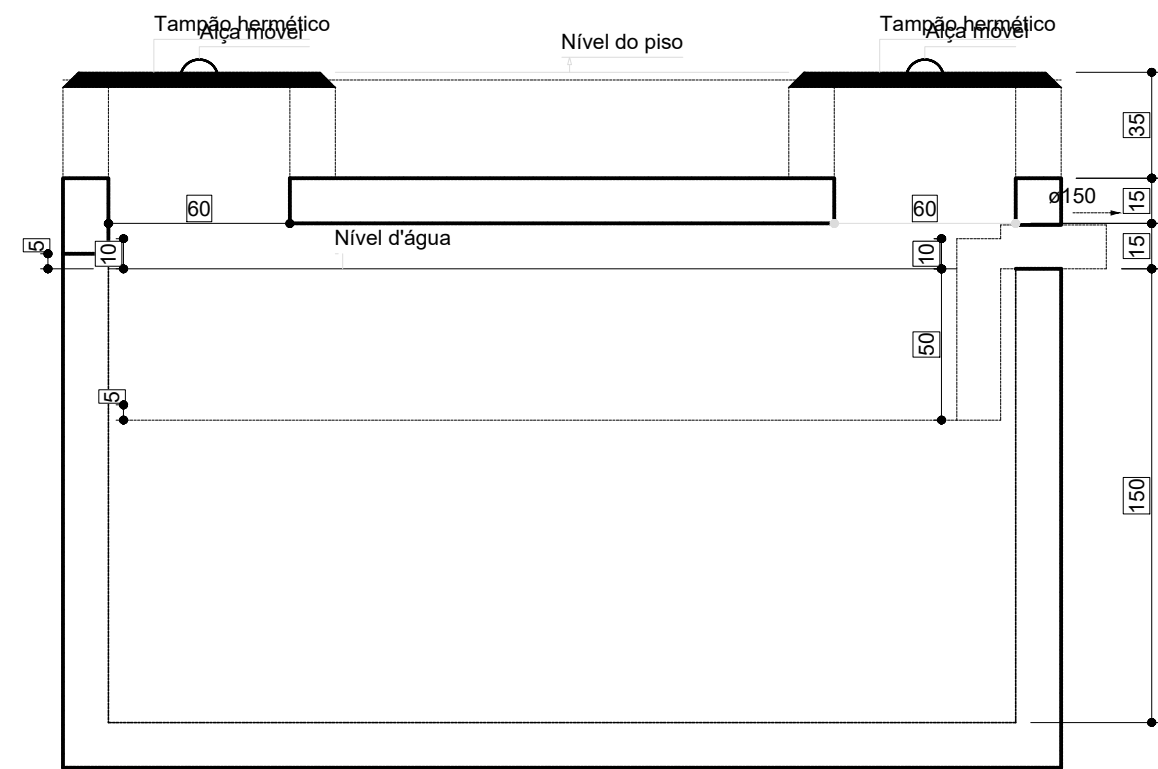
Tanque séptico - Pavimento Corte 1 - ESC. 1:100
