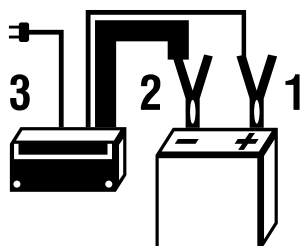
Fig. 3 – Secuencia para conectar el cargador
