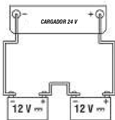
Fig. 6 – Carga en serie
