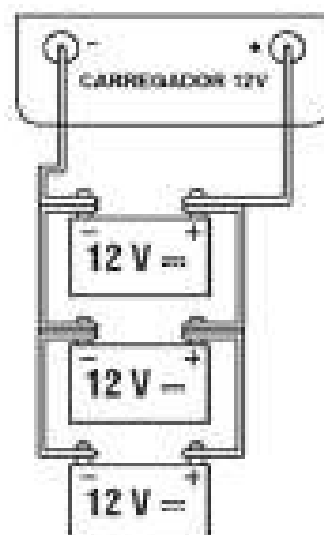
Fig. 5 – Carregamento em paralelo
