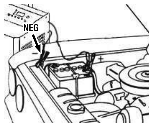
Fig. 4 – Carregamento com a bateria no veículo
