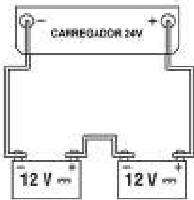
Fig. 6 – Carregamento em série
