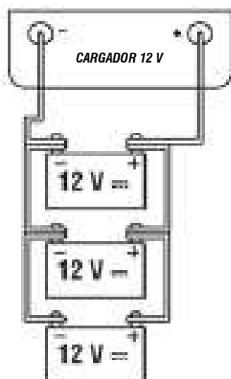
Fig. 5 – Carga paralelo
