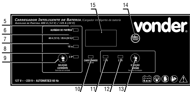
Fig. 2 – Painel de controle
