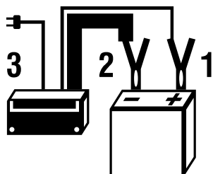
Fig. 3 – Sequência para ligar o carregador
