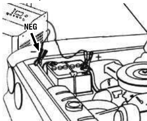
Fig. 4 – Carga con la batería en el vehículo
