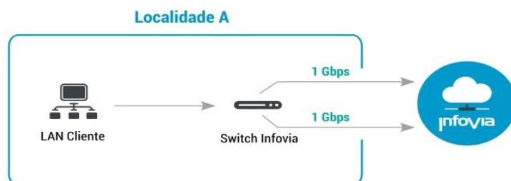
Figura 1: Infovia - Topologia Conexão Tipo 1 – 1 Gbps.
