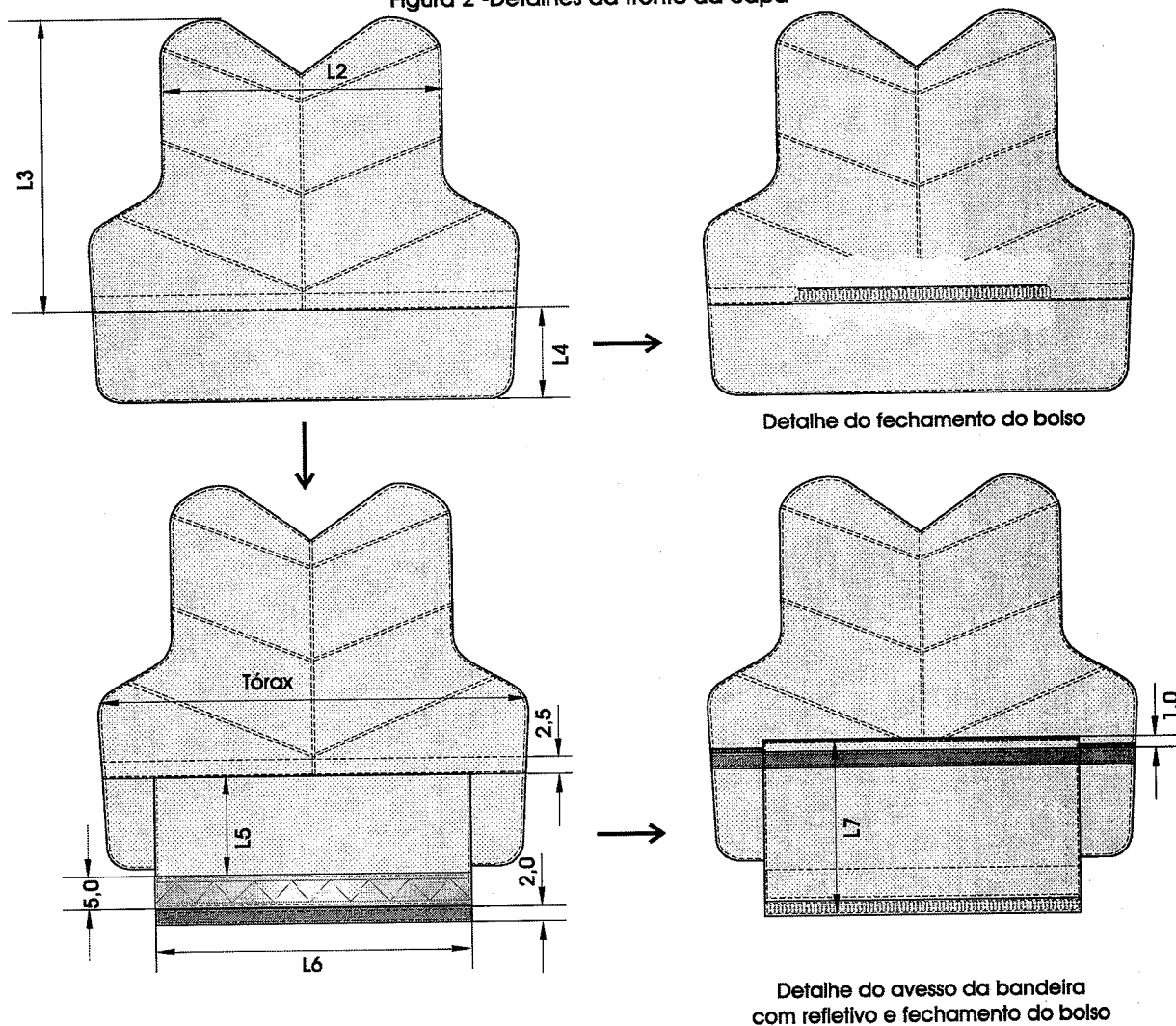
Figura 3 -Detalhes da face interna da frente da capa e do bolso para inserção da placa anti-impacto
