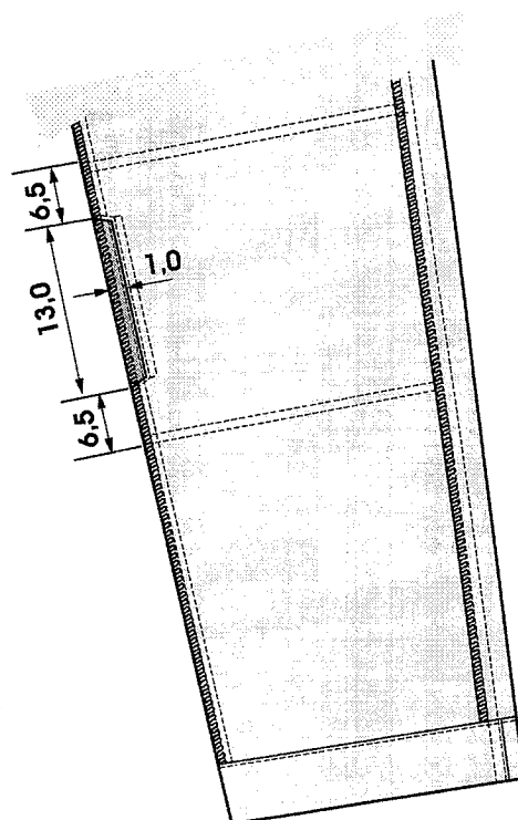
Figura 14- Detalhes do bolso localizado na face interna do reforço do joelho
