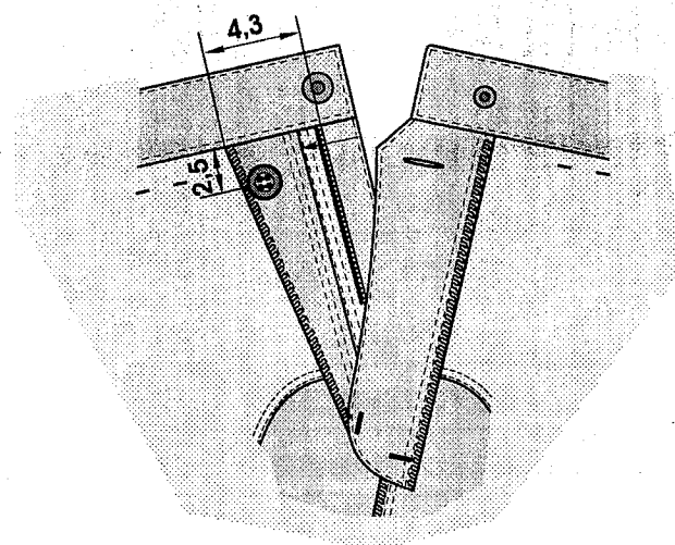
Figura 18- Detalhes da face interna da braguilha
