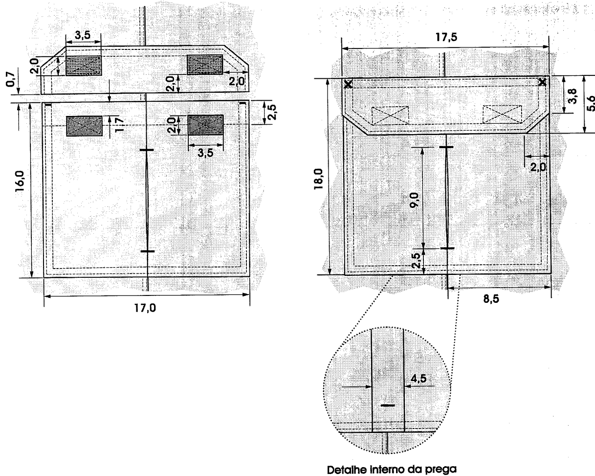
Figura 13 - Detalhes do bolso cargo
