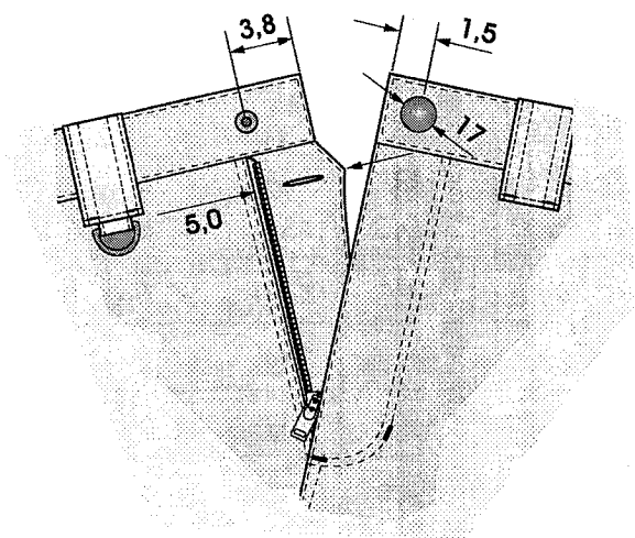
Figura 17- Detalhes da braguilha
