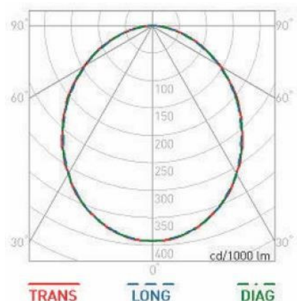
Curva de distribuição Fotométrica Ilustrativa - Ref. Itaim- Minotauro MS Premium
