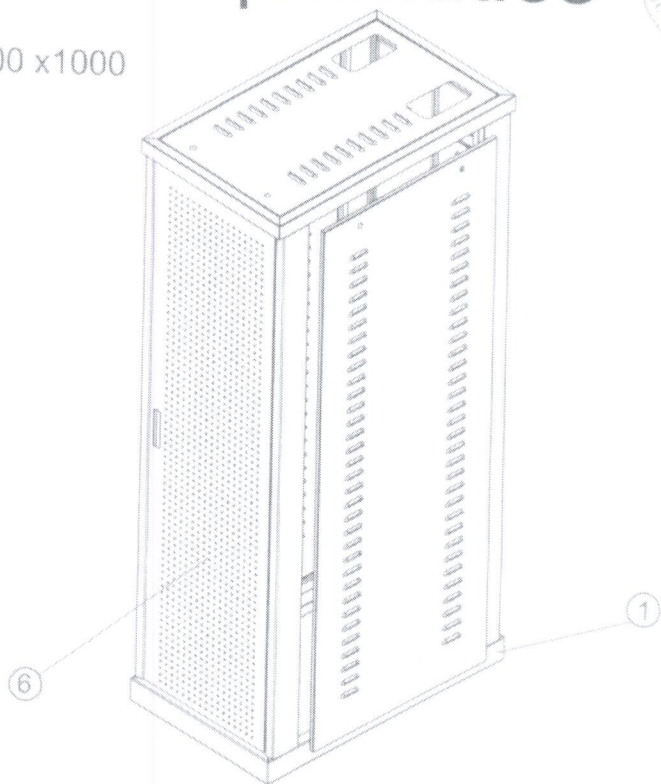
isometrica
