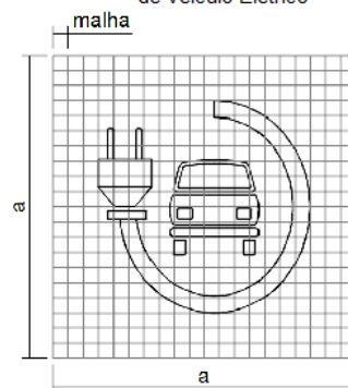
SAU - 30 Estação de Recarga de Veículo Elétrico
