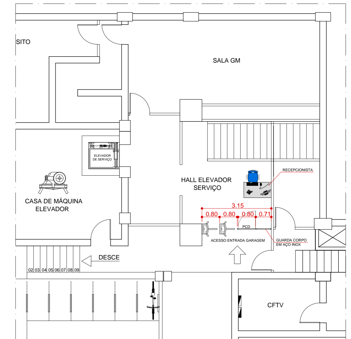
PROPOSTA ACESSO GARAGEM Escala 1:100
