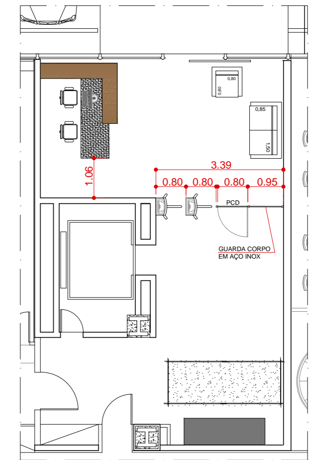
PROPOSTA ACESSO PRIVATIVO Escala 1:100
