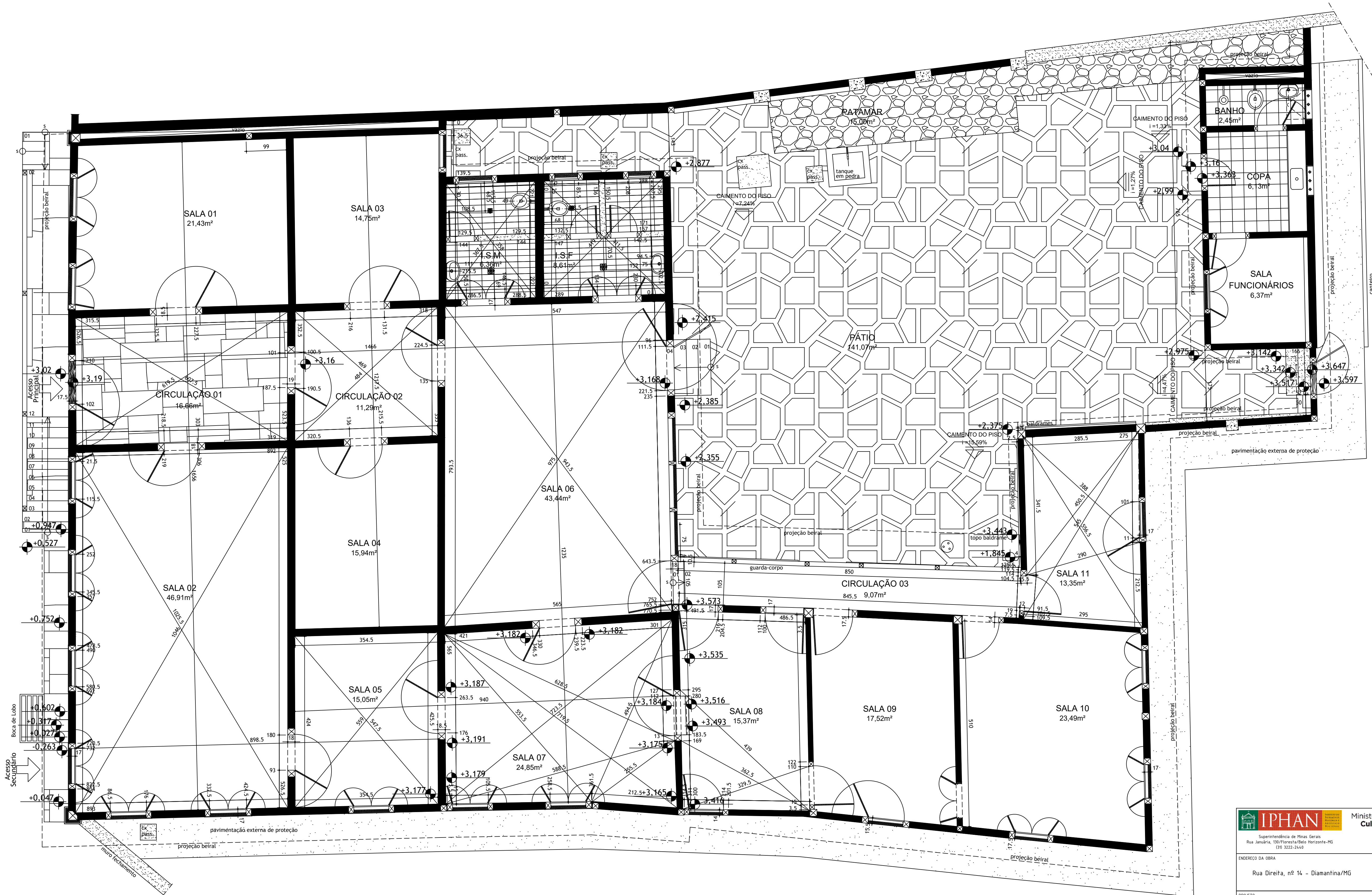
Planta 1º PAVIMENTO Levantamento Revisado por amostragem ESC 1/50 ÁREA DA EDIFICAÇÃO PRINCIPAL = 337,68m² ÁREA DA EDÍCULA = 19,46m²
