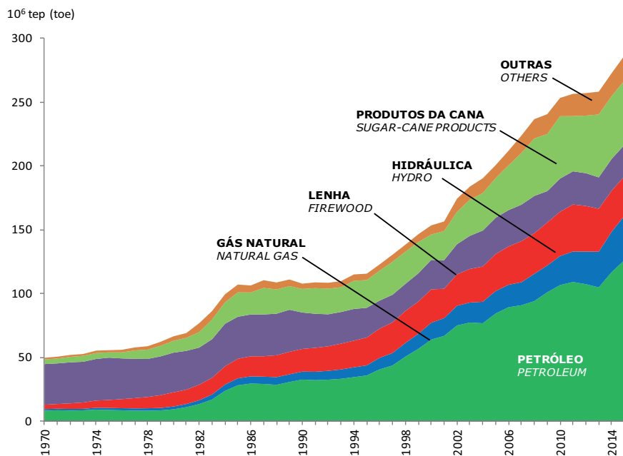
Gráfico 1.2.a – Produção de Energia Primária
