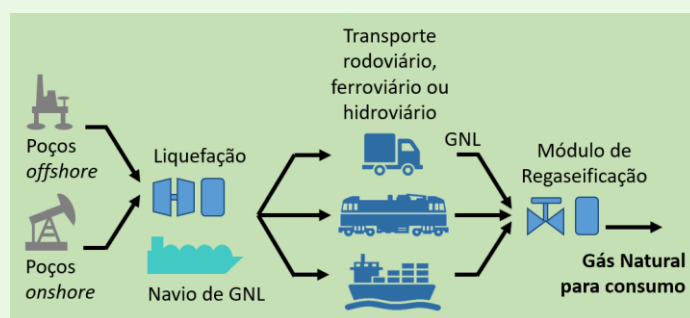
Figura 7-3 – Etapas do GNL em pequena escala a partir de poços produtores ou cargas de GNL de navios
