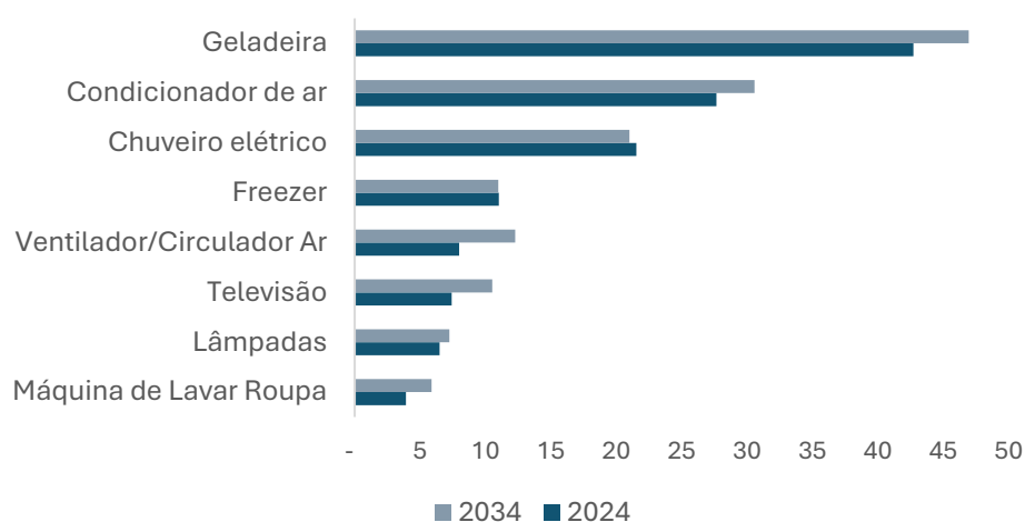
Figura 2-10 – Consumo de energia elétrica por equipamento residencial (TWh)
