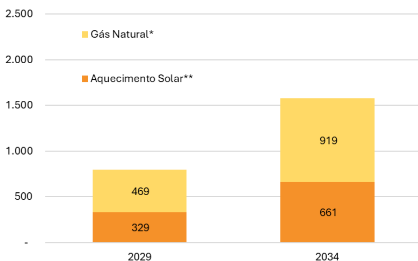
Figura 9-33 – Consumo evitado de eletricidade residencial para aquecimento de água utilizando outras fontes energéticas (GWh)
