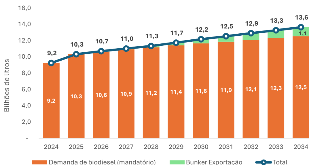
Figura 8-14 - Projeção do consumo total de biodiesel
