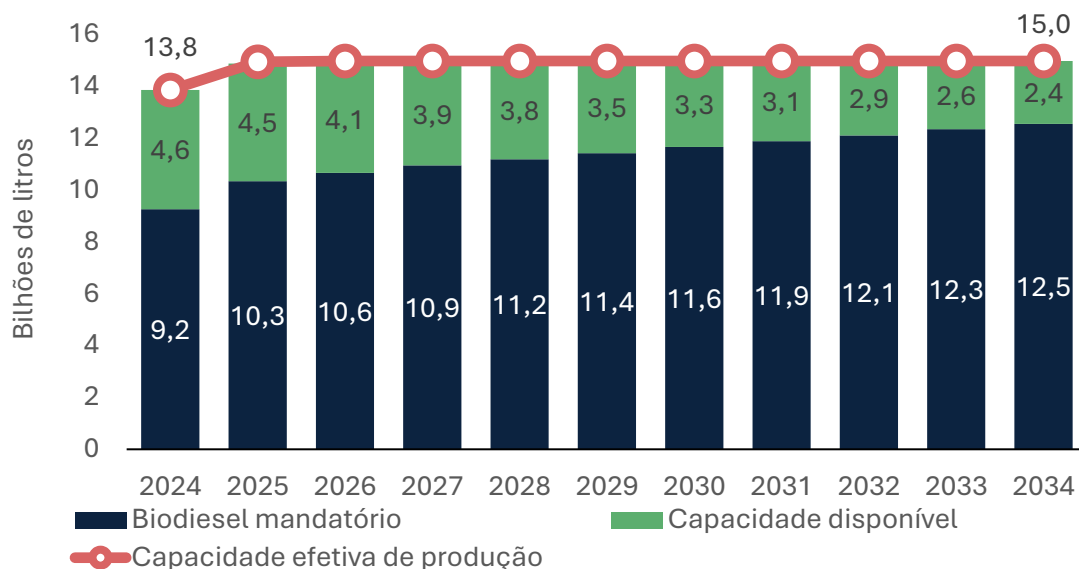
Figura 8-26 – Projeção da demanda de biodiesel para uso aquaviário
