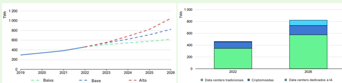
Figura 2-22 – Perspectivas para a demanda global de eletricidade relativa a data centers, IA e criptomoedas e cenários (2026)
