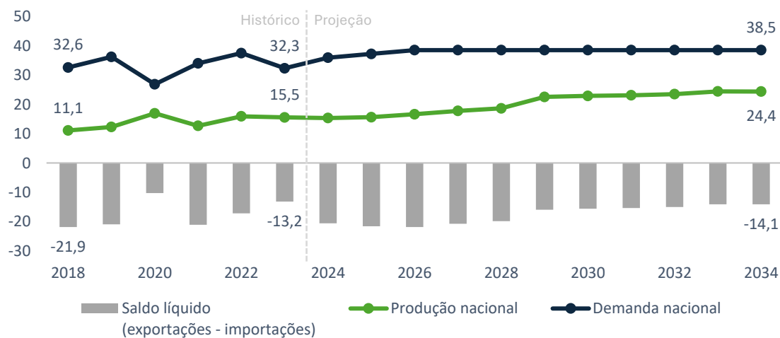
Figura 6-7 – Balanço nacional de nafta (mil m 3 /d)
