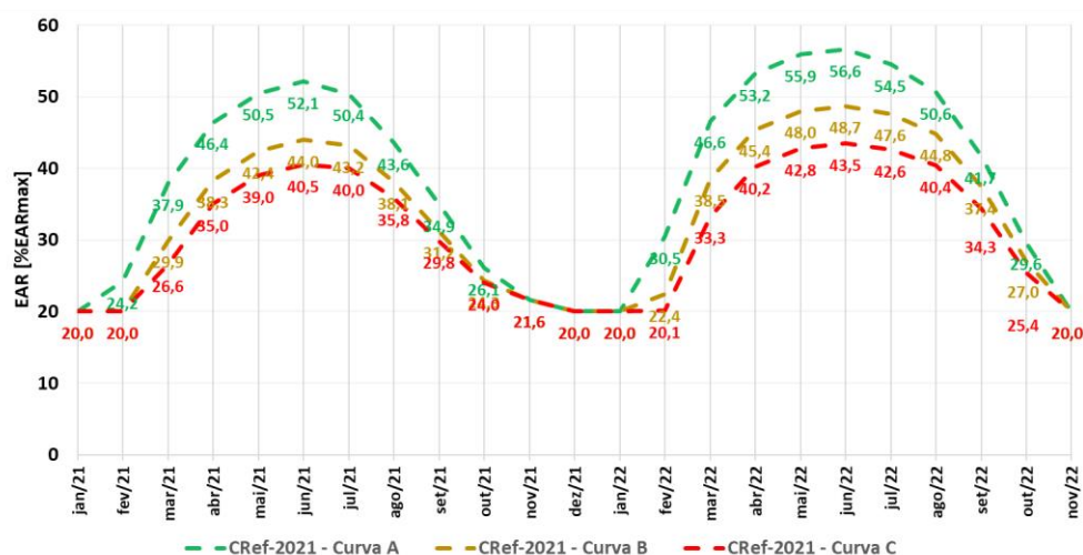
Figura 6-1: Curvas Originais
