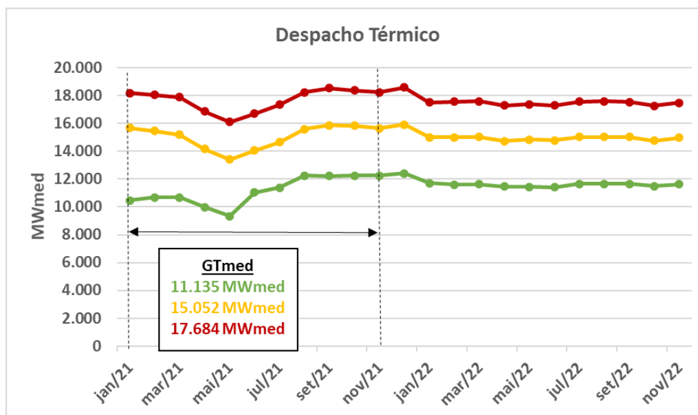
Figura 3-3: Despacho Térmico
