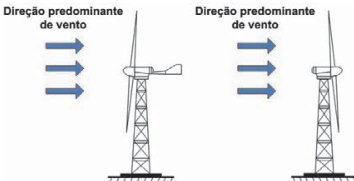
Figura 3.24 – Tipos de rotores com relação à sua orientação, da esquerda para a direita: upwind e downwind
