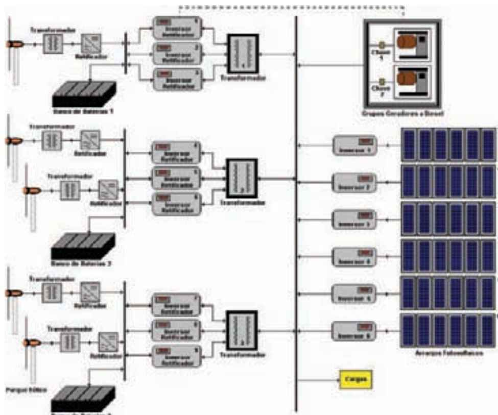
Figura 13.14 – Diagrama de blocos do sistema Sucuriçu
