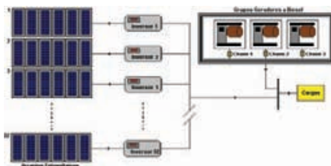
Figura 13.10 – Diagrama de blocos do sistema de Araras
