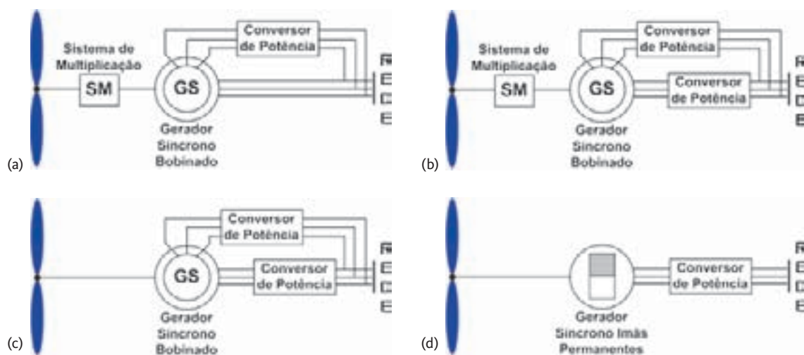
Figura 3.32 – Configurações de sistemas eólicos com geradores síncronos
