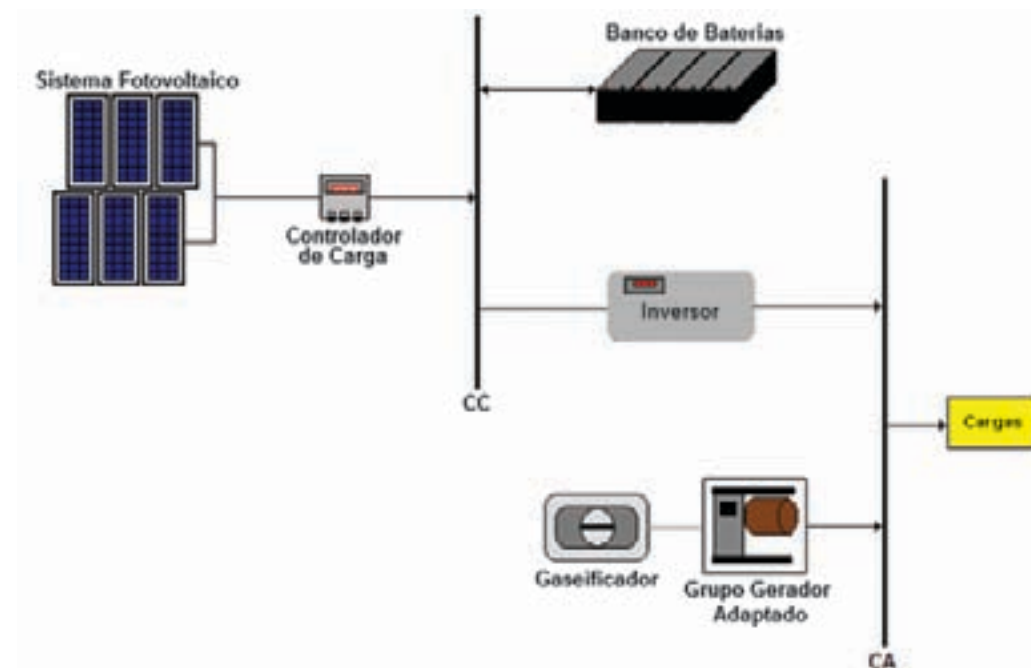
Figura 7.21 – Diagrama de blocos de um sistema híbrido fotovoltaico-biomassa-gasificação
