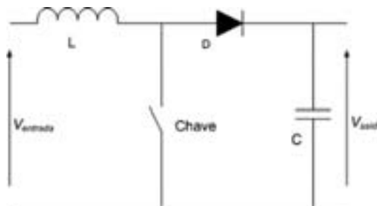
Figura 6.17 – Circuito de um conversor buck
