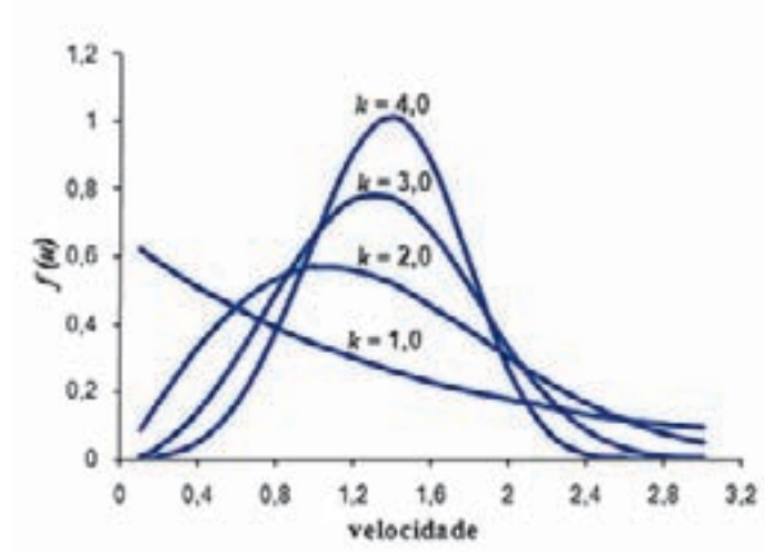
Figura 3.19 – Funções de Weibull para C = 2 m/s e diferentes valores de k
