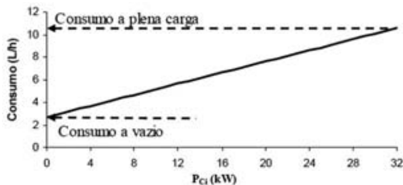
Figura 4.26 – Curva de consumo de um grupo gerador [BLASQUES, 2005].
