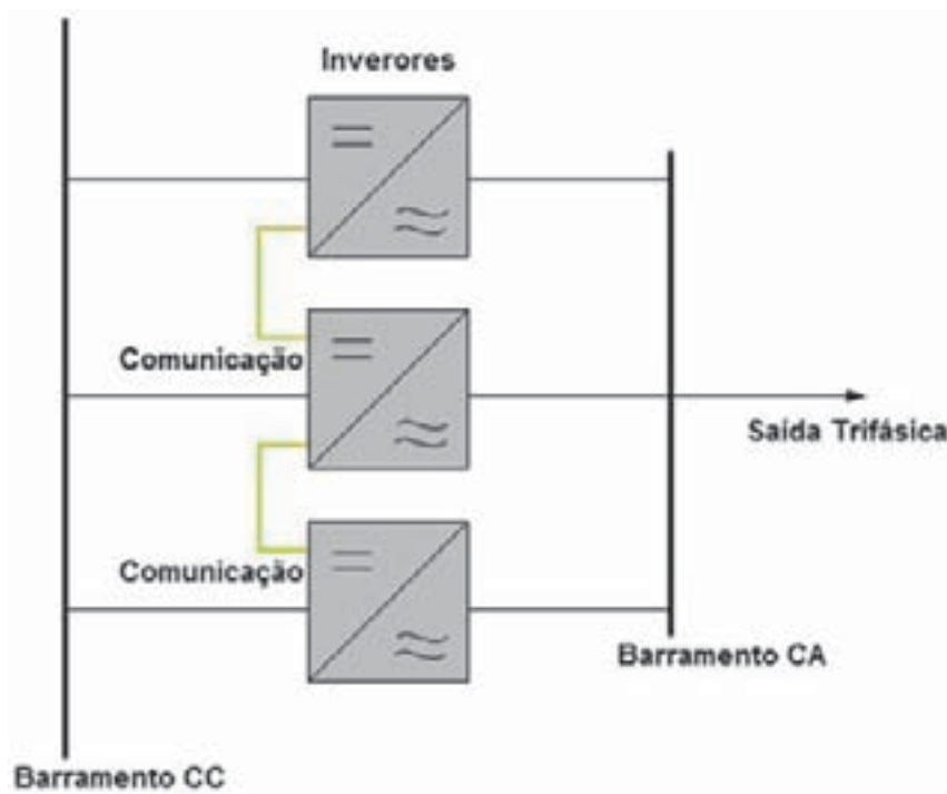
(a) Inversores monofásicos associados
