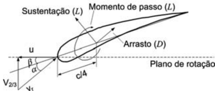
Figura 3.27 – Conceitos referentes à teoria do aerofólio
