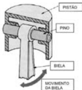
Figura 4.9 – Conjunto pistão, pino e biela [SODRÉ, 2008]
