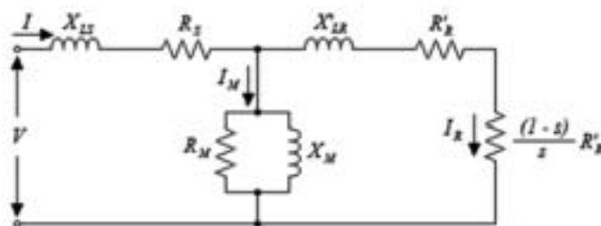
Figura 3.33 – Circuito equivalente de uma máquina de indução
