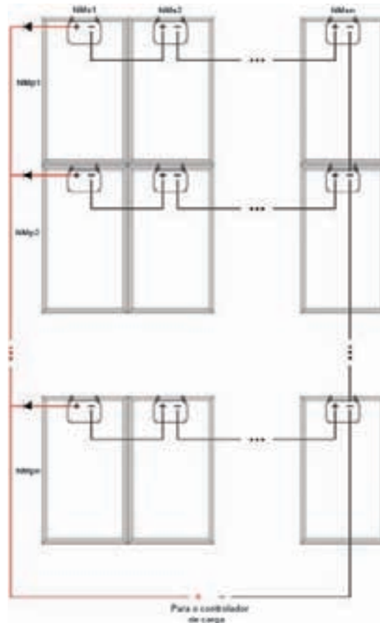
Figura 9.6 – Exemplo geral de associação mista de módulos
