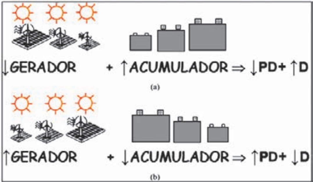
Figura 5.12 – Inf uência do dimensionamento do gerador e da bateria nos parâmetros PD e e D: (a) diminuindo o tamanho do gerador e aumentando o acumulador; (b) aumentando o tamanho do gerador e diminuindo o tamanho do acumulador
