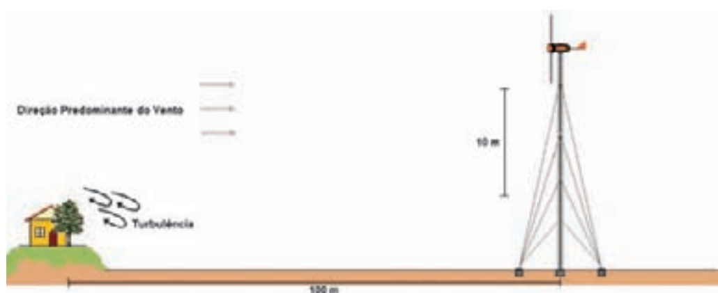
Figura 9.17 – Outra técnica de instalação de aerogerador
