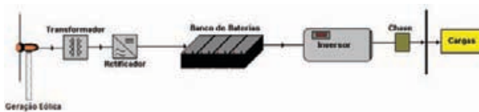
Figura 3.43 – Configuração típica de um sistema eólico isolado
