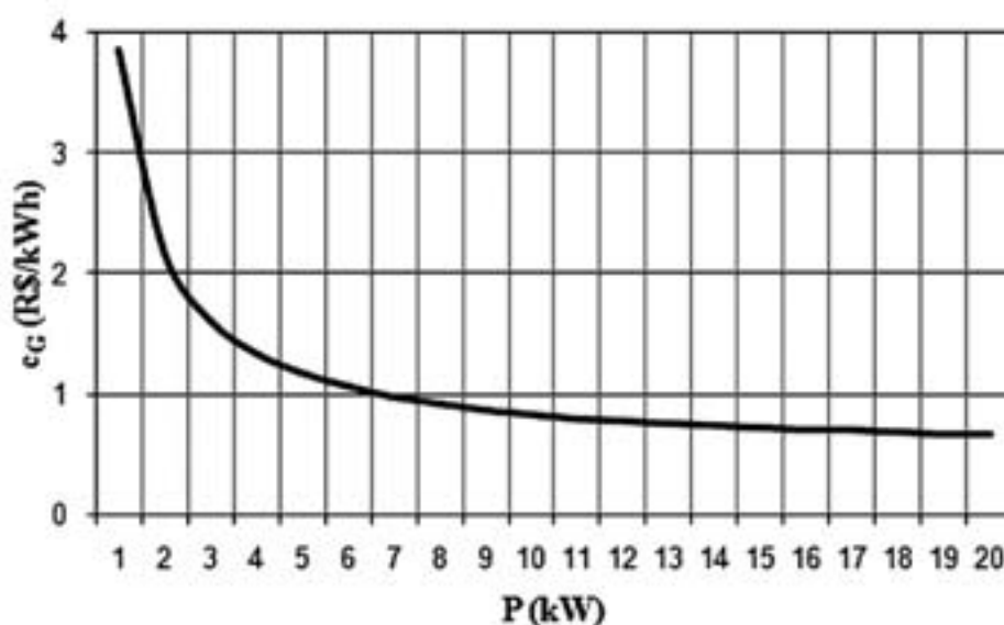
Figura 12.4 – Custo da energia gerada por um grupo gerador a diesel de 20 kW
