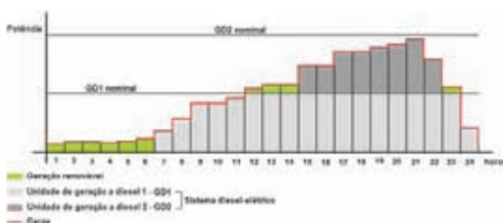
Figura 7.13 – Representação do comportamento de um sistema híbrido baseado no recurso não renovável
