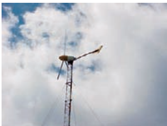
Aerogerador com o leme dobrado (retirada da direção predominante do vento)
