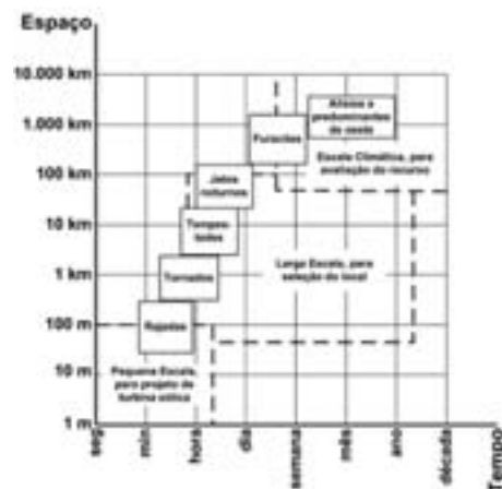
Figura 3.3 – Escalas espacial e temporal de movimento dos ventos Fonte: SPERA, 1994
