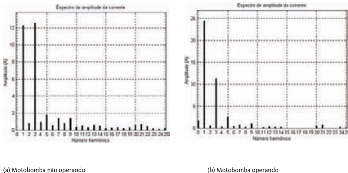
Figura 13.20 – Espectro harmônico de amplitude da corrente no neutro (São Tomé)
