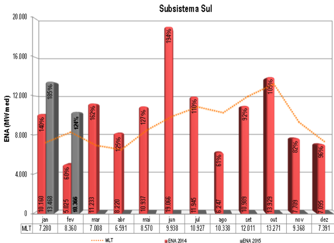
Figura 5: Energia Natural Afluyente/MLT (Subsistema Sul)
