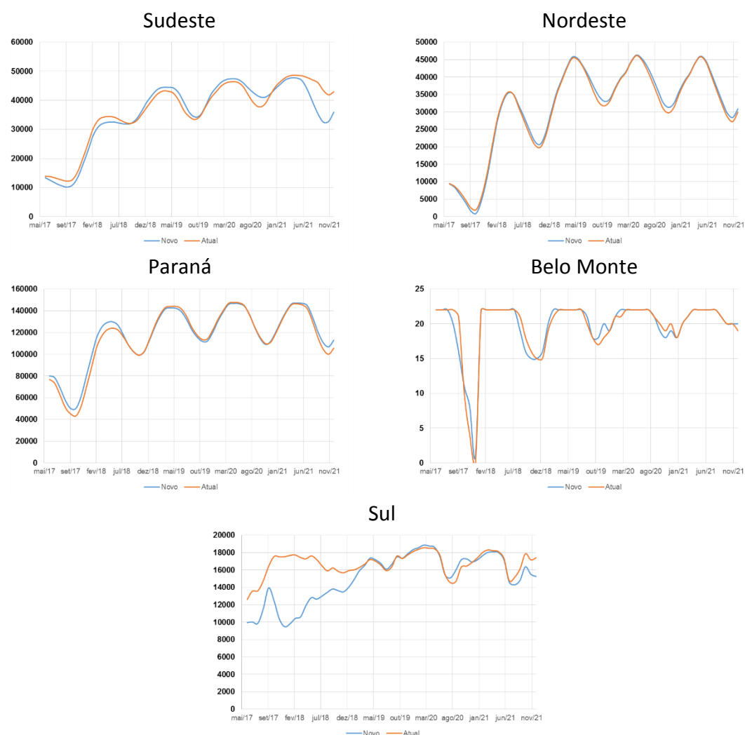
Figura 56- Evolução temporal da energia armazenada final dos REE's selecionados – PLD junho/2017
