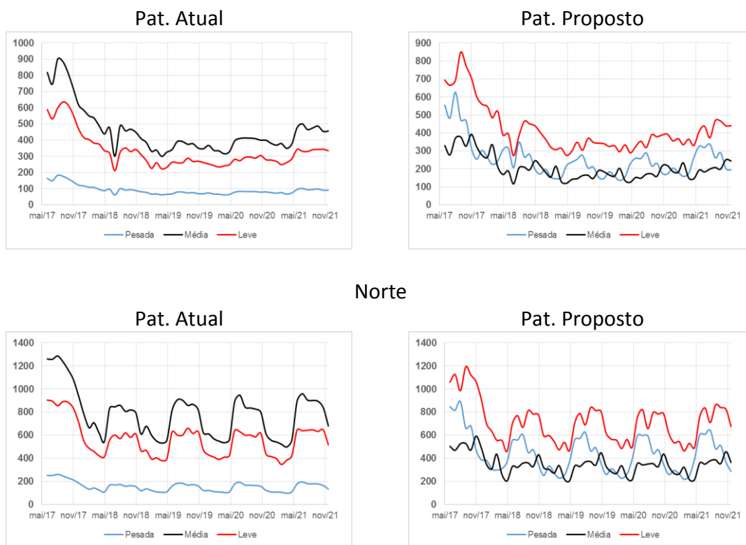
Figura 58- Evolução temporal da geração térmica total final dos REE's selecionados – PLD junho/2017
