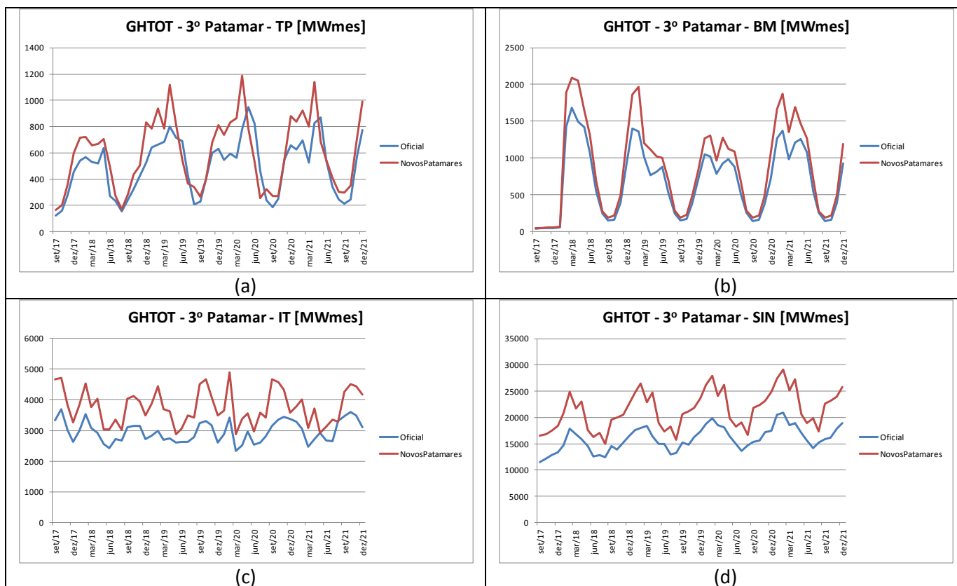
Figura 85 – Evolução temporal da geração hidráulica total dos REEs e do SIN para o patamar de carga leve: (a) Teles Pires; (b) Belo Monte; (c) Itaipu; e (d) SIN – PMO Set/2017
