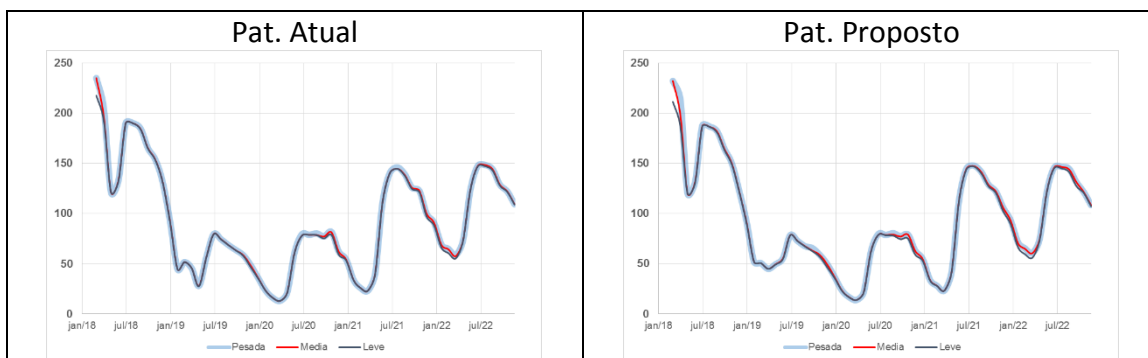
Figura 43 - Evolução temporal do CMO do Nordeste – PLD março/2018
