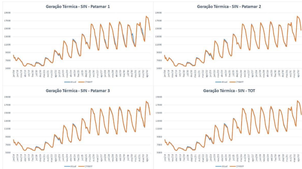
Figura 34 – Geração térmica total por patamar
