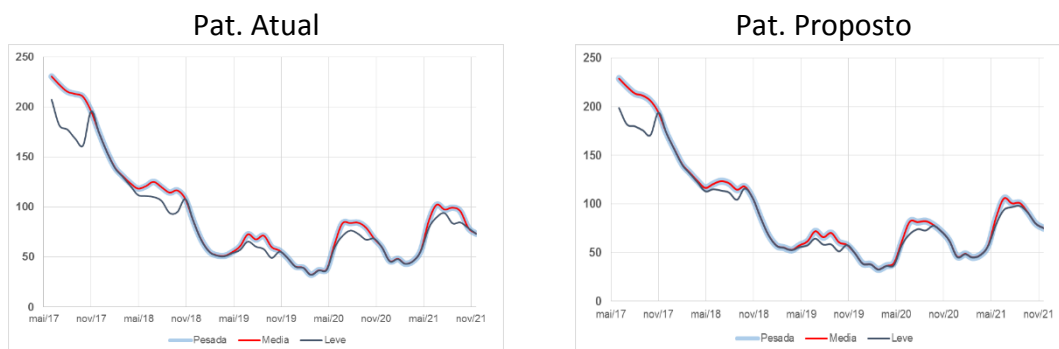
Figura 54- Evolução temporal do CMO do Sul – PLD junho/2017
