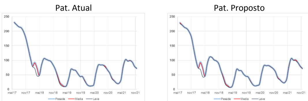
Figura 55- Evolução temporal do CMO do Sul – PLD junho/2017
