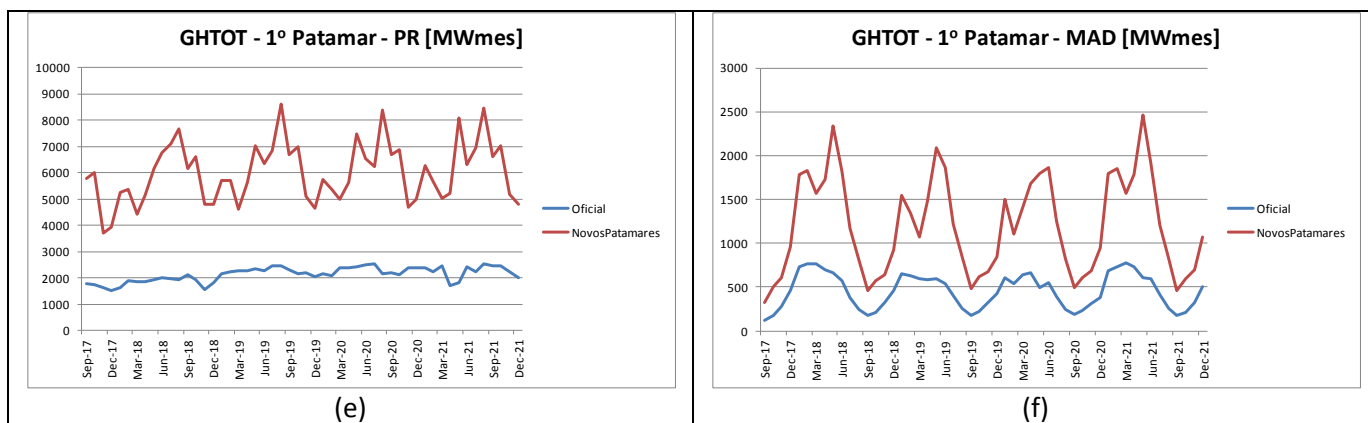
Figura 80 – Evolução temporal da geração hidráulica total dos REEs para o patamar de carga pesada: (a) Sudeste; (b) Sul; (c) Nordeste; (d) Norte; (e) Paraná; e (f) Madeira – PMO Set/2017
