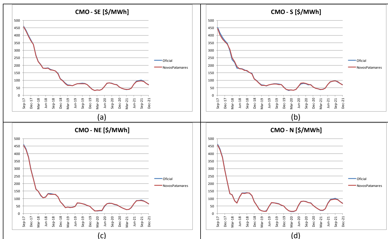
Figura 63 – Evolução temporal do CMO dos submercados: (a) Sudeste; (b) Sul; (c) Nordeste; e (d) Norte – PMO Set/2017
