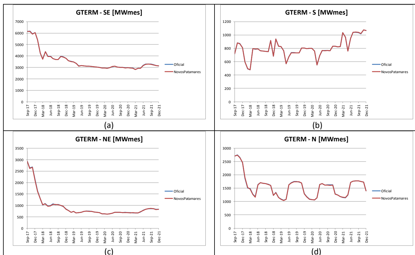
Figura 71 – Evolução temporal da geração térmica dos submercados: (a) Sudeste; (b) Sul; (c) Nordeste; e (d) Norte – PMO Set/2017
