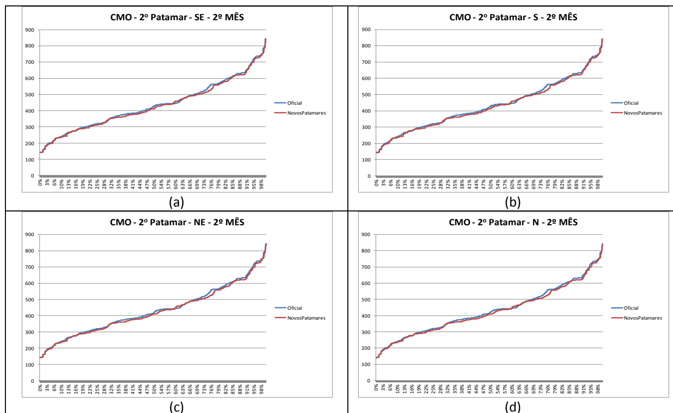
Figura 69 – Curva de permanência do CMO do patamar de carga média dos submercados: (a) Sudeste; (b) Sul; (c) Nordeste; e (d) Norte – PMO Set/2017
