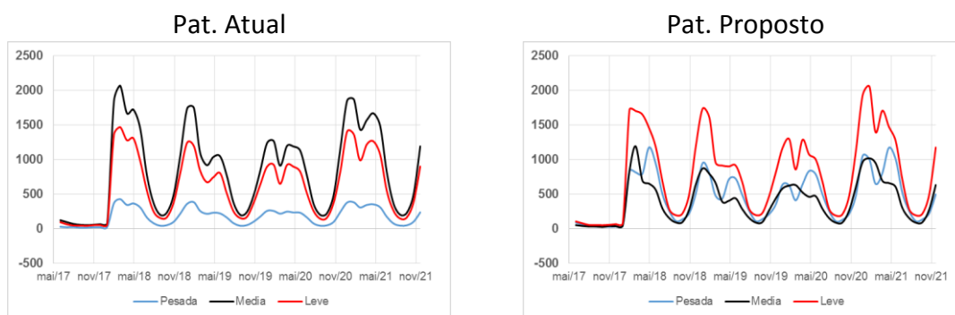
Figura 57- Evolução temporal da geração hidráulica total final dos REE's selecionados – PLD junho/2017
