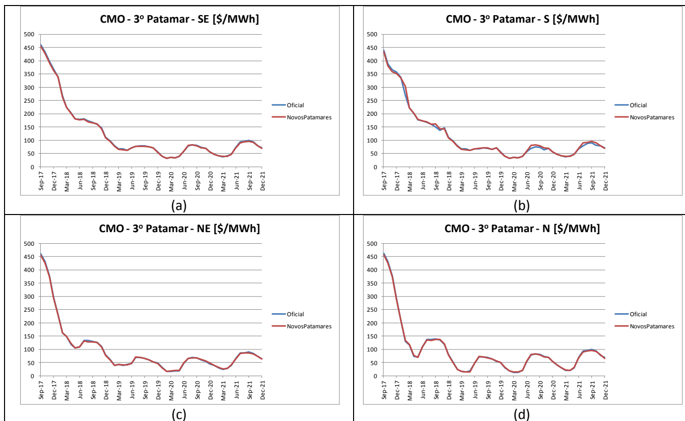
Figura 66 – Evolução temporal do CMO do patamar de carga leve dos submercados: (a) Sudeste; (b) Sul; (c) Nordeste; e (d) Norte – PMO Set/2017
