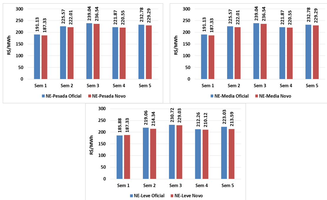
Figura 49 - PLD Mar/2018 RV0 – Nordeste
