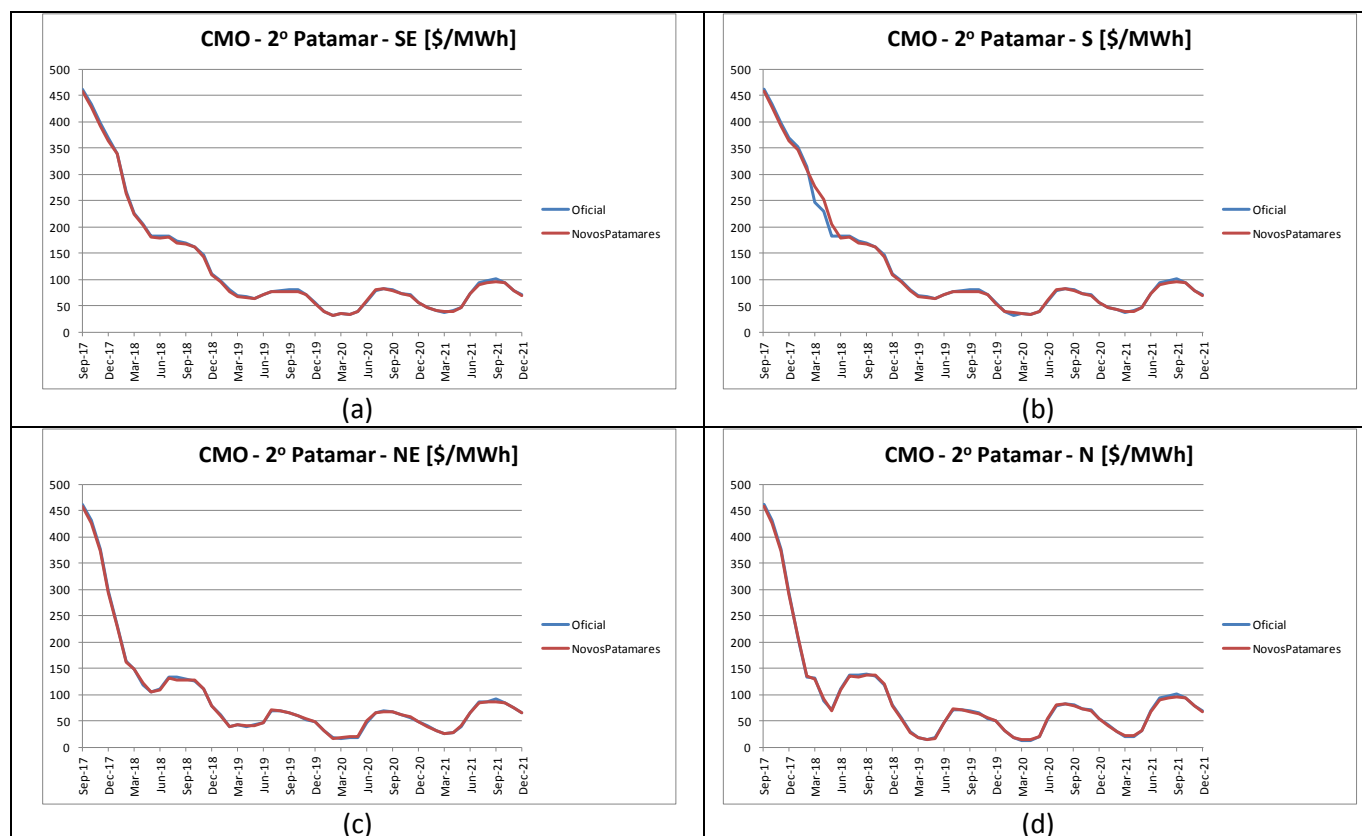
Figura 65 – Evolução temporal do CMO do patamar de carga média dos submercados: (a) Sudeste; (b) Sul; (c) Nordeste; e (d) Norte – PMO Set/2017
