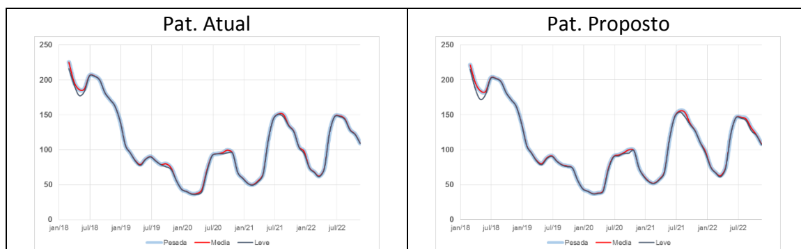
Figura 41- Evolução temporal do CMO do Sudeste – PLD março/2018
