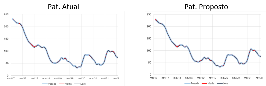
Figura 52 - Evolução temporal do CMO do Sudeste – PLD junho/2017
