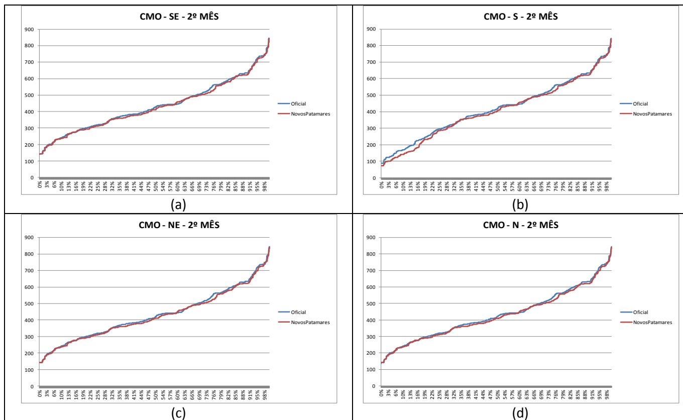
Figura 67 – Curva de permanência do CMO dos submercados: (a) Sudeste; (b) Sul; (c) Nordeste; e (d) Norte – PMO Set/2017
