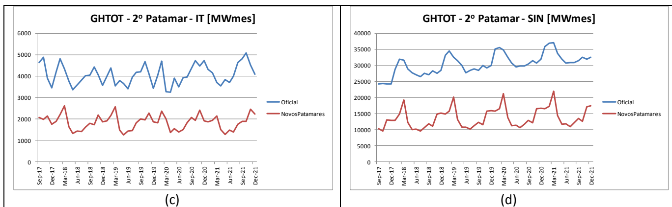
Figura 83 – Evolução temporal da geração hidráulica total dos REEs e do SIN para o patamar de carga média: (a) Teles Pires; (b) Belo Monte; (c) Itaçu; e (d) SIN – PMO Set/2017
