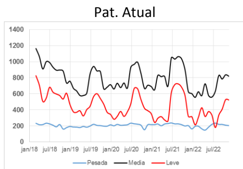
Figura 46 - Evolução temporal da geração hidráulica total final dos REE's selecionados – PLD março/2018
