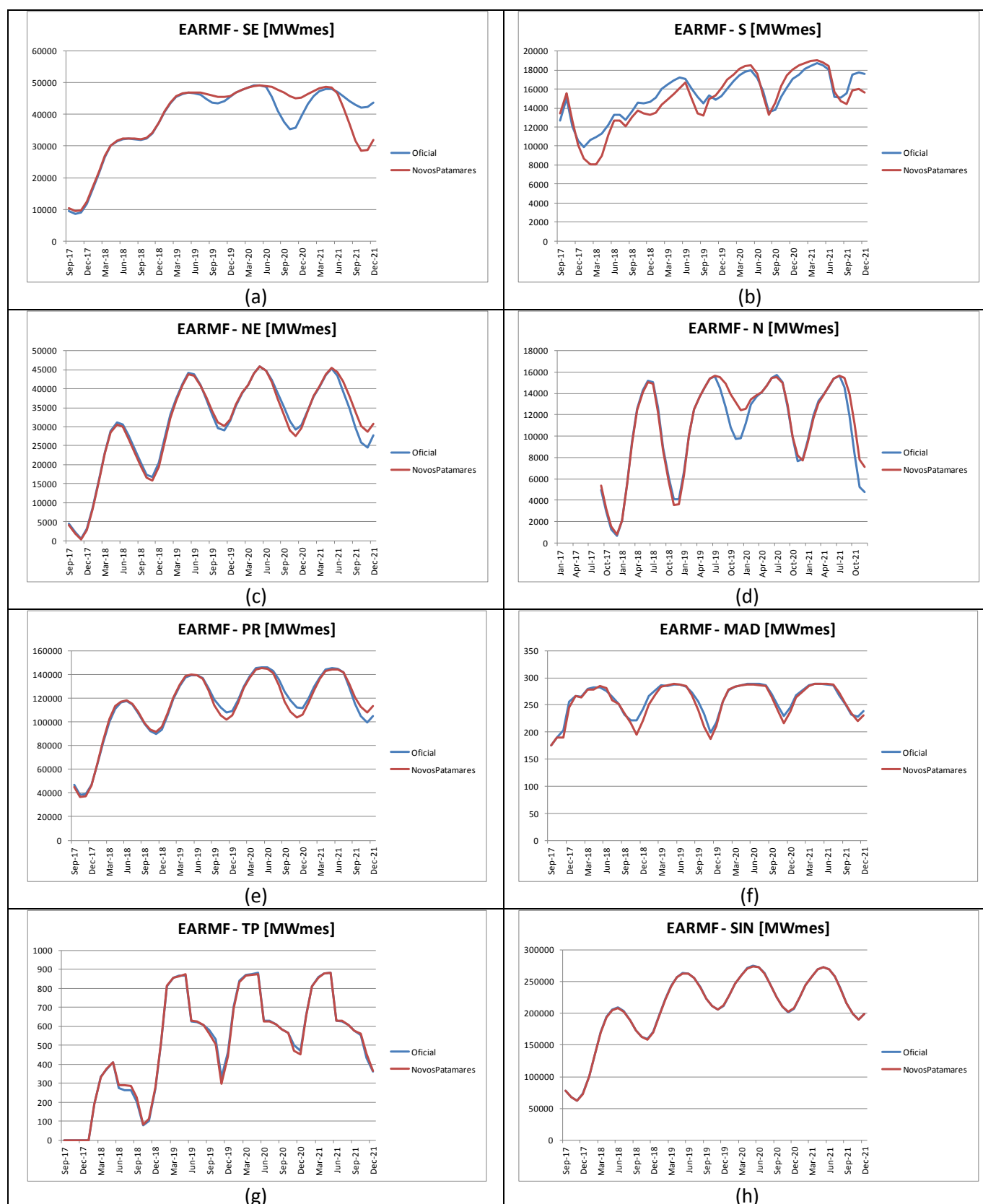
Figura 76 – Evolução temporal da energia armazenada final dos REEs do SIN: (a) Sudeste; (b) Sul; (c) Nordeste; (d) Norte; (e) Paraná; (f) Madeira; (g) Teles Pires; e (h) SIN – PMO Set/2017
