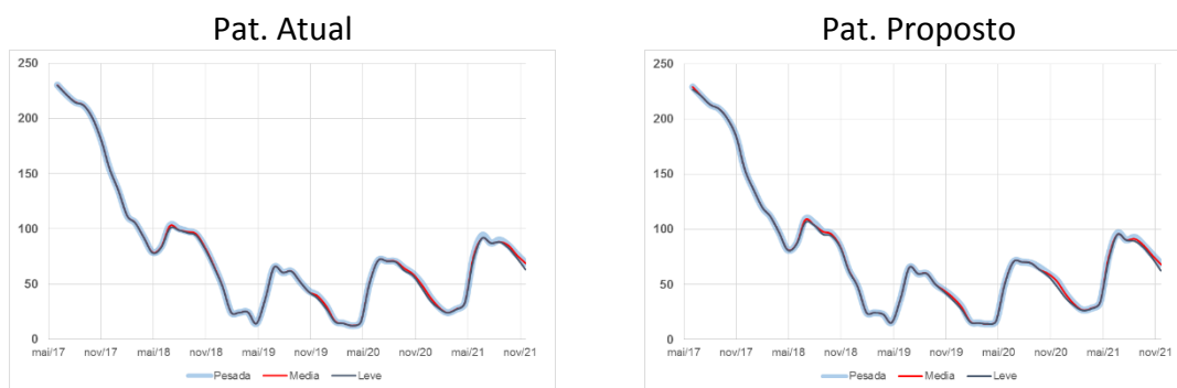
Figura 53- Evolução temporal do CMO do Nordeste – PLD junho/2017
