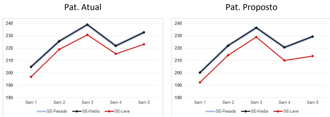
Figura 50 - Comparação PLD Sudeste – março/2018
