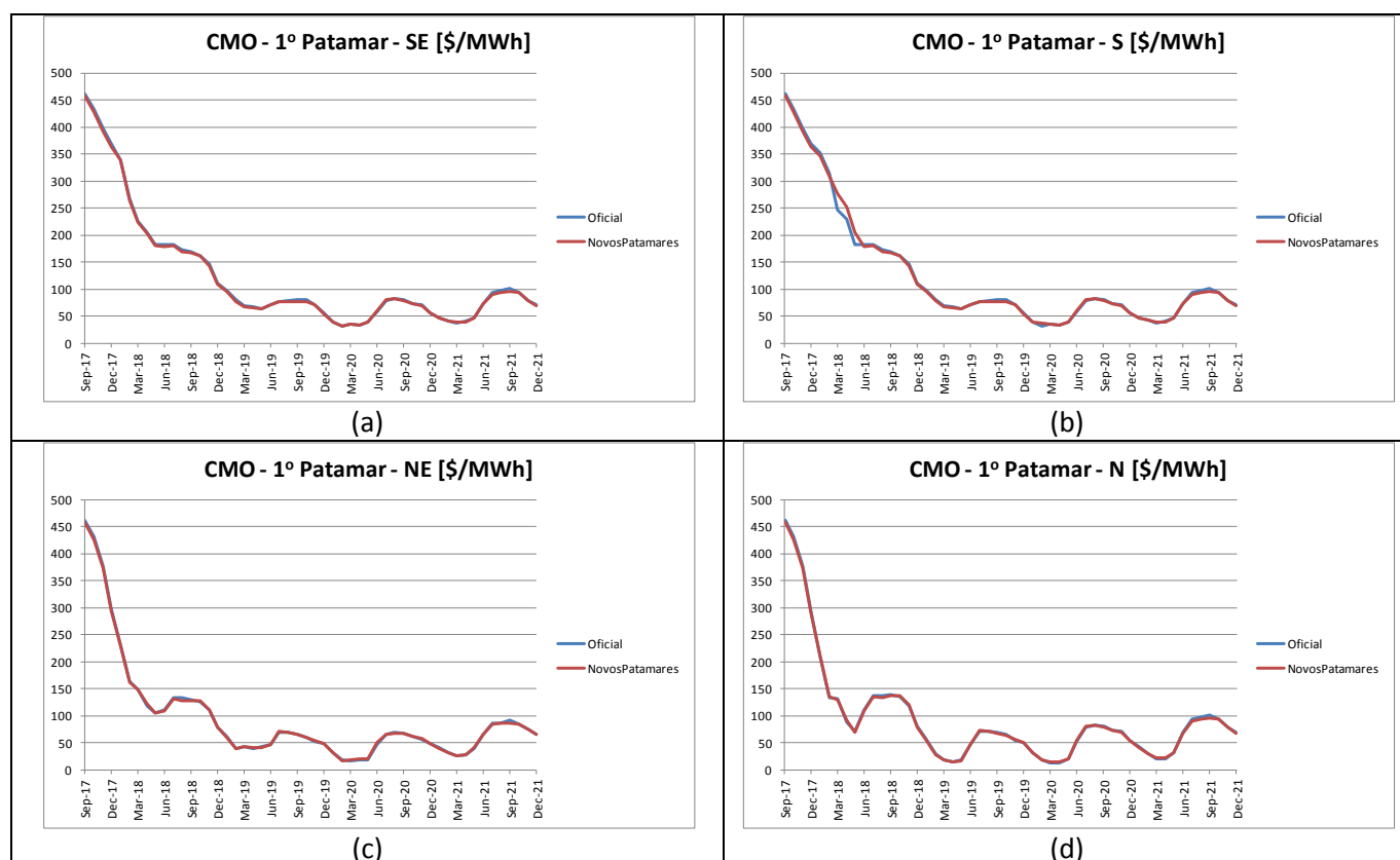
Figura 64– Evolução temporal do CMO do patamar de carga pesada dos submercados: (a) Sudeste; (b) Sul; (c) Nordeste; e (d) Norte – PMO Set/2017
