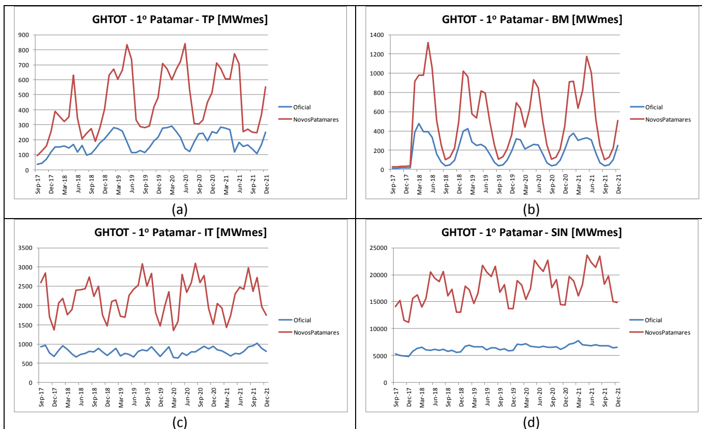
Figura 81 – Evolução temporal da geração hidráulica total dos REEs e do SIN para o patamar de carga pesada: (a) Teles Pires; (b) Belo Monte; (c) Itaipu; e (d) SIN – PMO Set/2017
