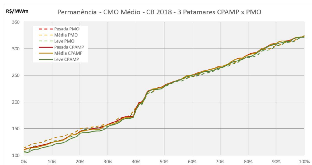
Figura 38 – Permanência do CMO – Valor Médio - Caso Base LEN A-4 2018
