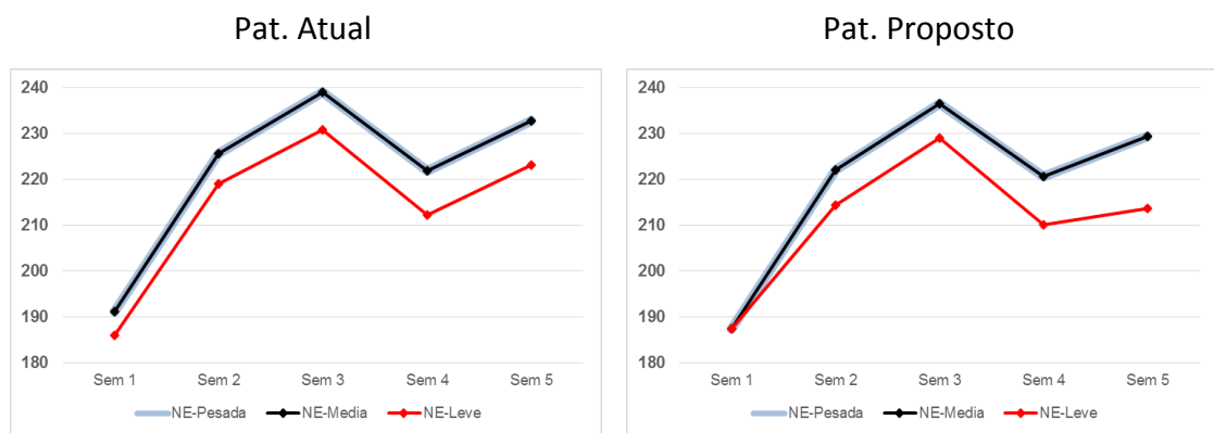
Figura 51 - Comparação PLD Nordeste – março/2018
