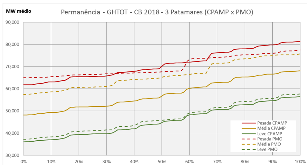
Figura 39 – Geração Hidráulica - Caso Base LEN A-4 2018
