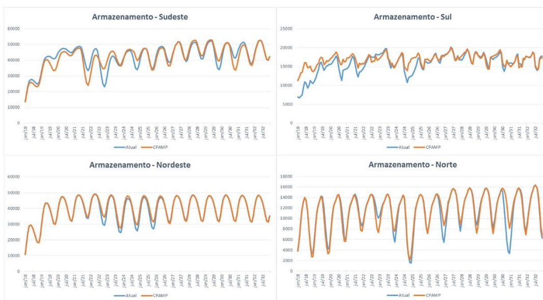
Figura 36 – Armazenamento final por subsistema
