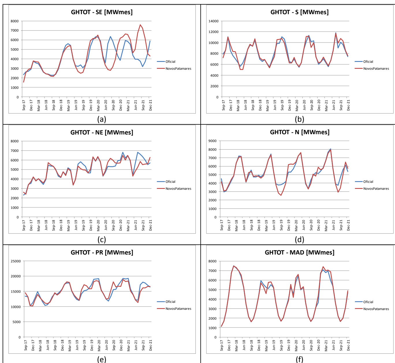
Figura 78 – Evolução temporal da geração hidráulica total dos REEs: (a) Sudeste; (b) Sul; (c) Nordeste; (d) Norte; (e) Paraná; e (f) Madeira – PMO Set/2017
