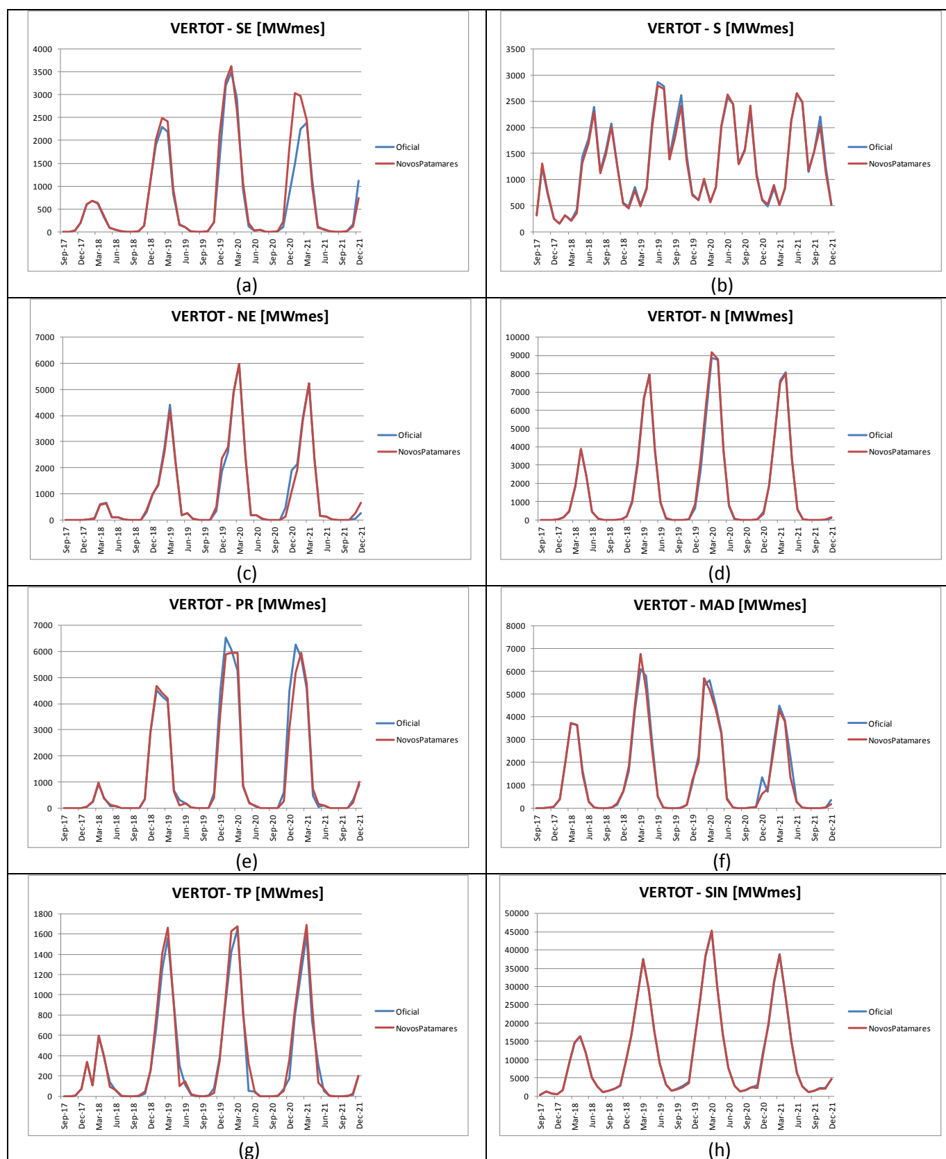
Figura 86 – Evolução temporal da energia vertida dos REEs do SIN: (a) Sudeste; (b) Sul; (c) Nordeste; (d) Norte; (e) Paraná; (f) Madeira; (g) Teles Pires; e (h) SIN – PMO Set/2017
