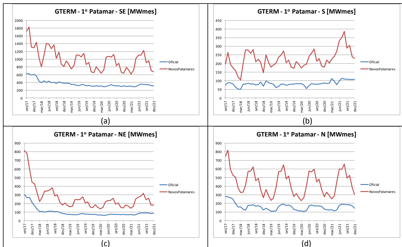
Figura 72 – Evolução temporal da geração térmica para o patamar de carga pesada dos submercados: (a) Sudeste; (b) Sul; (c) Nordeste; e (d) Norte – PMO Set/2017
