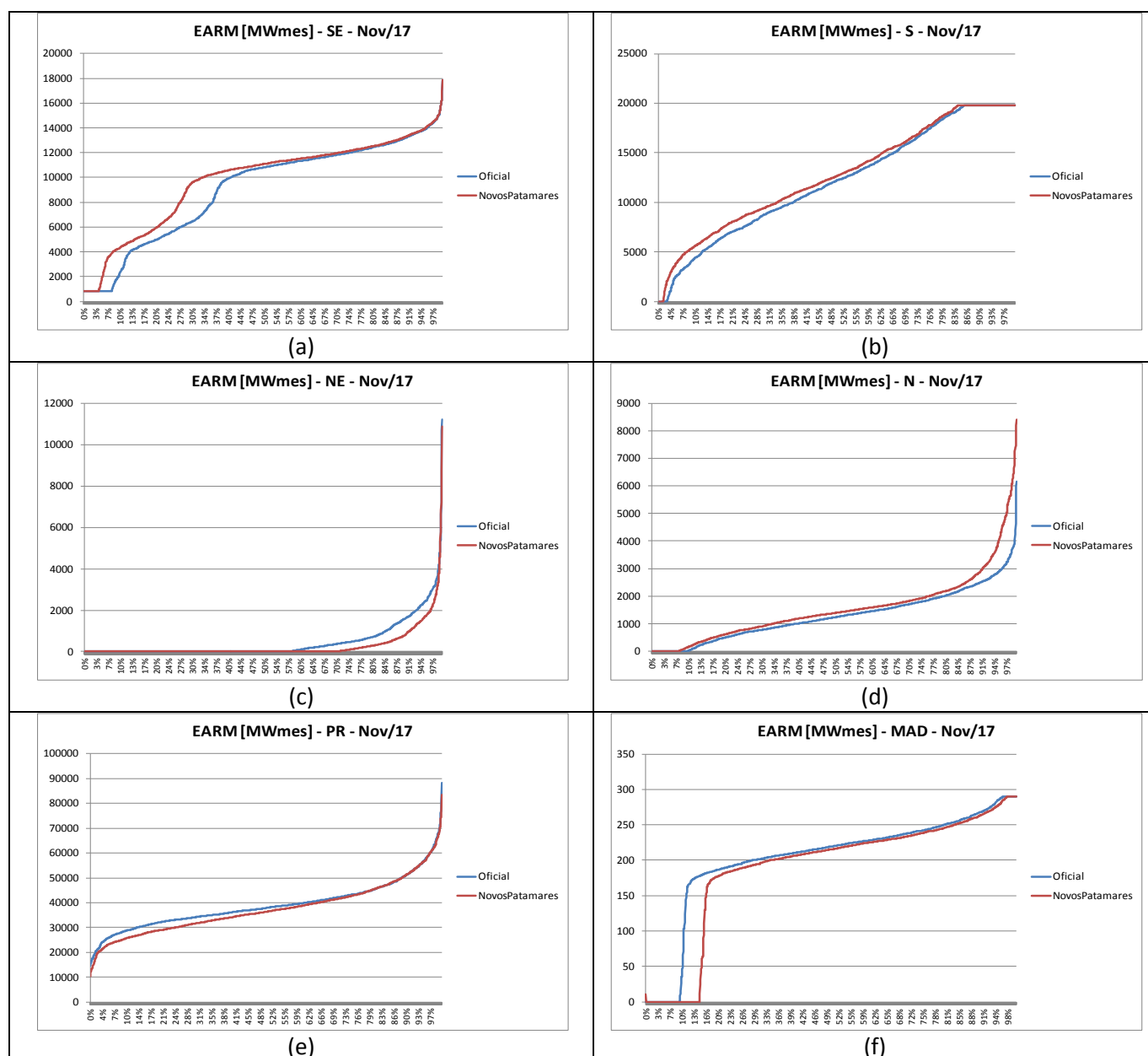
Figura 77 – Curva de permanência da energia armazenada final dos REEs em Novembro/2017: (a) Sudeste; (b) Sul; (c) Nordeste; (d) Norte; (e) Paraná; e (f) Madeira – PMO Set/2017
