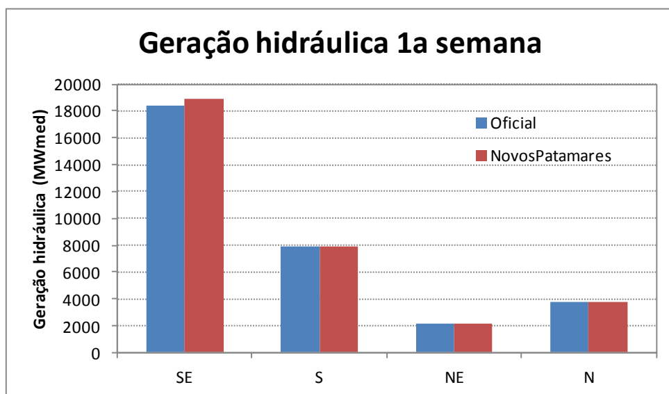
Figura 90 – Geração hidráulica da 1ª semana por submercados – PMO Set/2017
