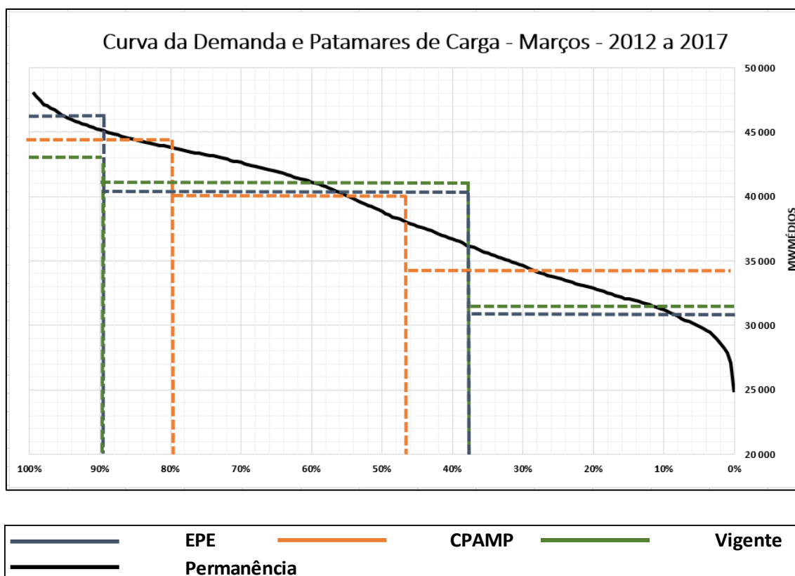
Figura 29 – Curva de demanda e patamares de carga
