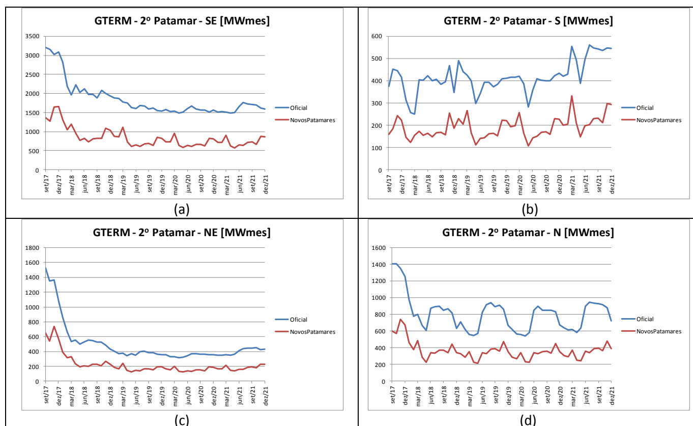
Figura 73 – Evolução temporal da geração térmica para o patamar de carga média dos submercados: (a) Sudeste; (b) Sul; (c) Nordeste; e (d) Norte – PMO Set/2017
