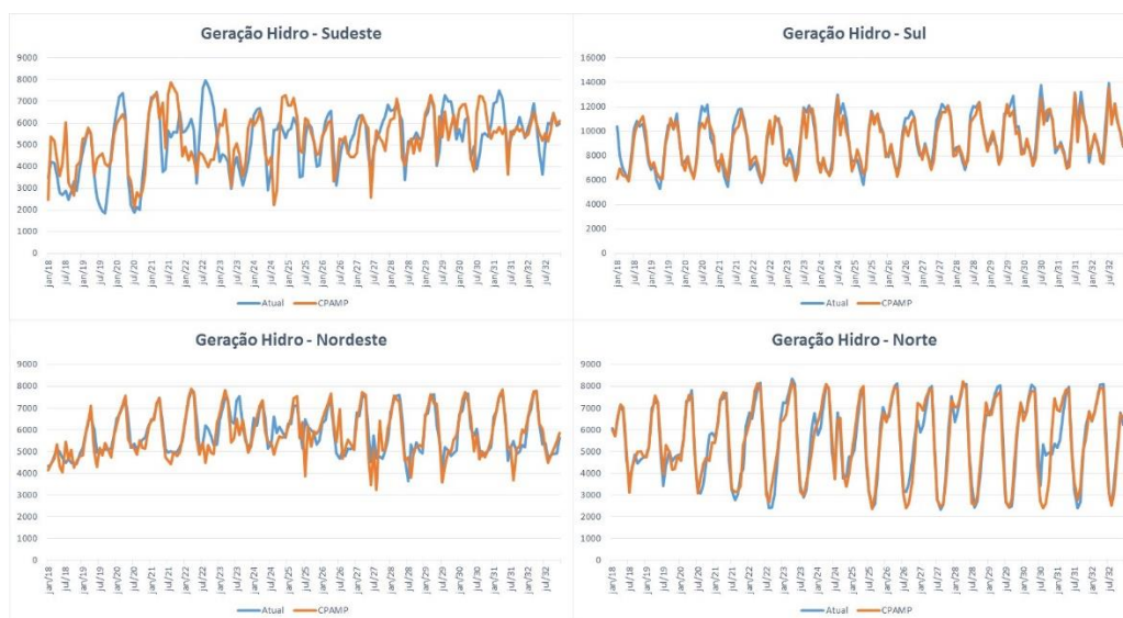
Figura 32 – Geração Hidrelétrica – Patamar 2
