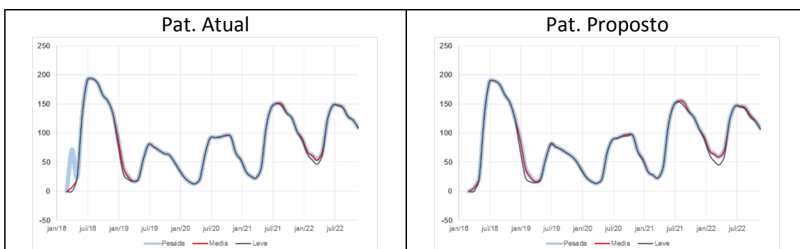
Figura 44 - Evolução temporal do CMO do Norte – PLD março/2018
