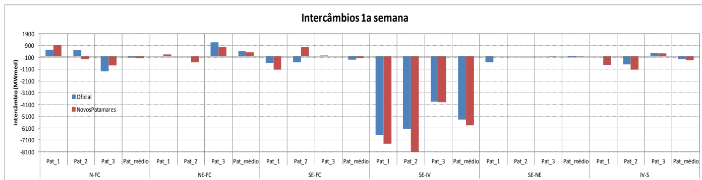
Figura 91 – Intercâmbio da 1ª semana por patamar de carga – PMO Set/2017
