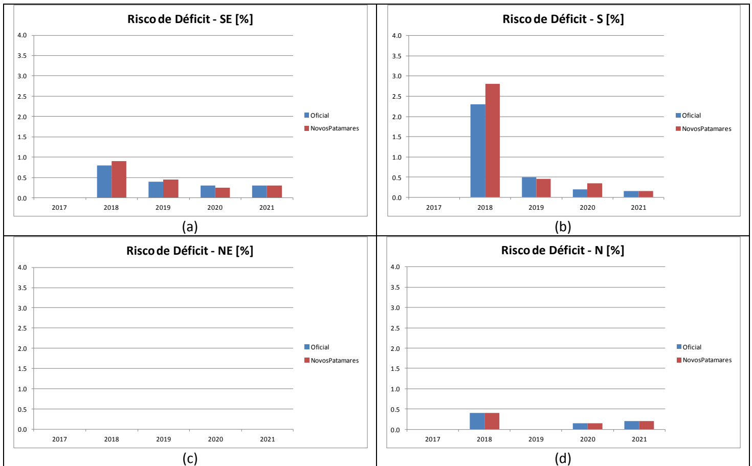
Figura 87 – Risco de déficit de energia dos submercados: (a) Sudeste; (b) Sul; (c) Nordeste; e (d) Norte – PMO Set/2017
