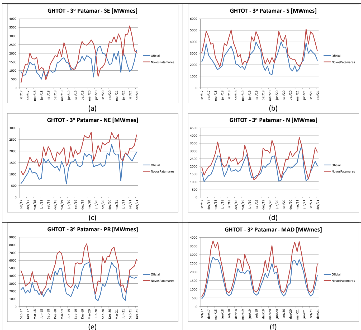
Figura 84 – Evolução temporal da geração hidráulica total dos REEs para o patamar de carga leve: (a) Sudeste; (b) Sul; (c) Nordeste; (d) Norte; (e) Paraná; e (f) Madeira – PMO Set/2017
