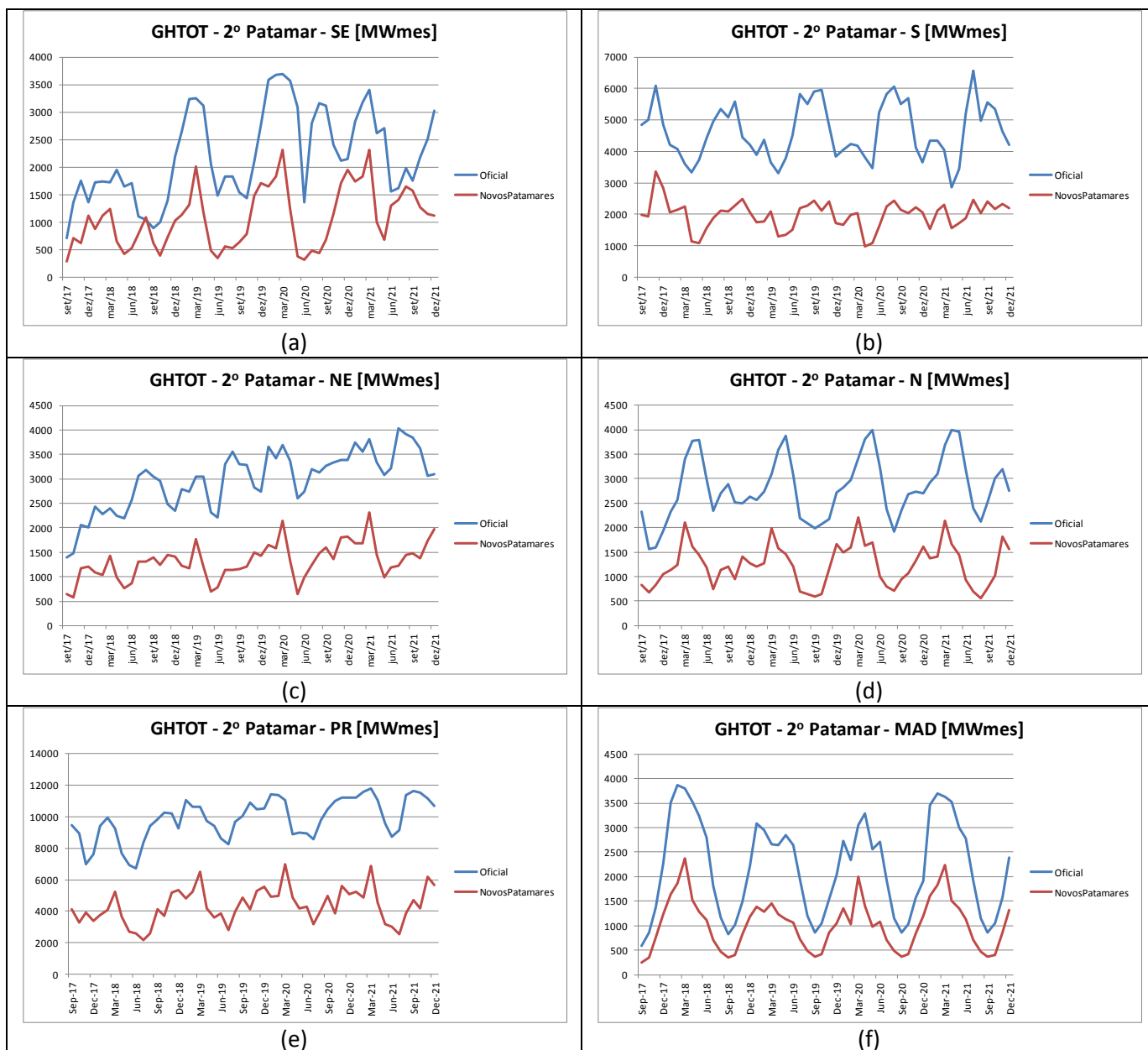
Figura 82 – Evolução temporal da geração hidráulica total dos REEs para o patamar de carga média: (a) Sudeste; (b) Sul; (c) Nordeste; (d) Norte; (e) Paraná; e (f) Madeira – PMO Set/2017
