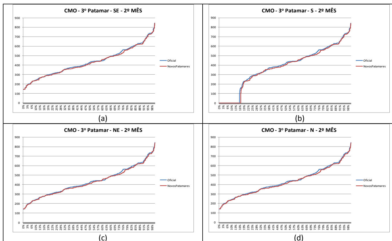
Figura 70 – Curva de permanência do CMO do patamar de carga leve dos submercados: (a) Sudeste; (b) Sul; (c) Nordeste; e (d) Norte – PMO Set/2017
