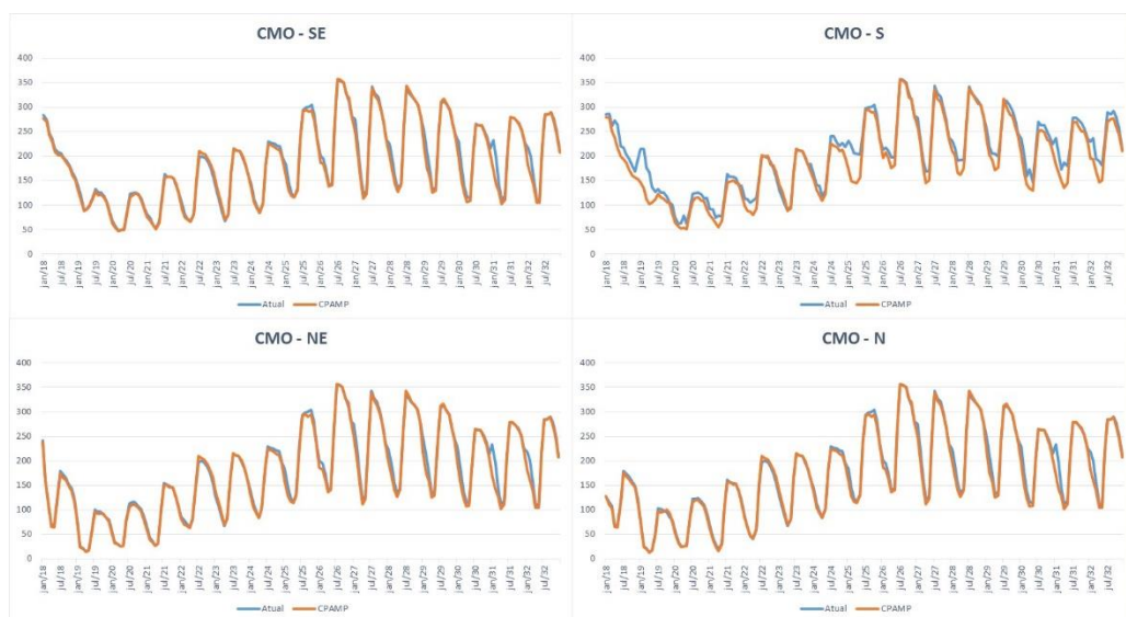
Figura 35 – Custo Marginal de Operação (CMO) por subsistema
