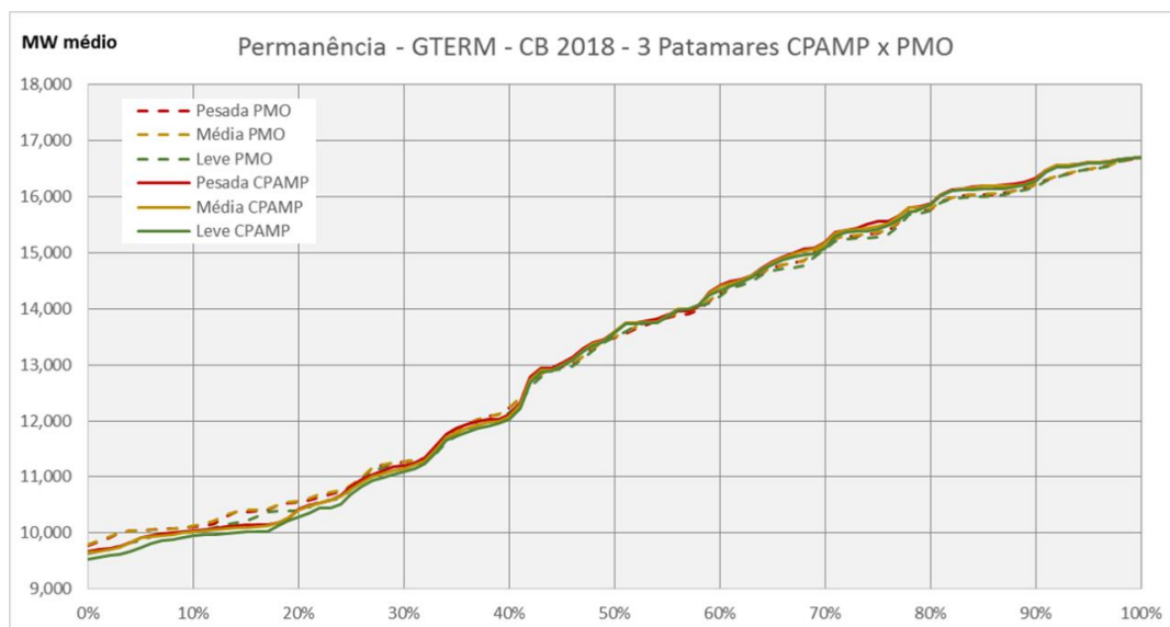
Figura 40 – Geração Térmica - Caso Base LEN A-4 2018
