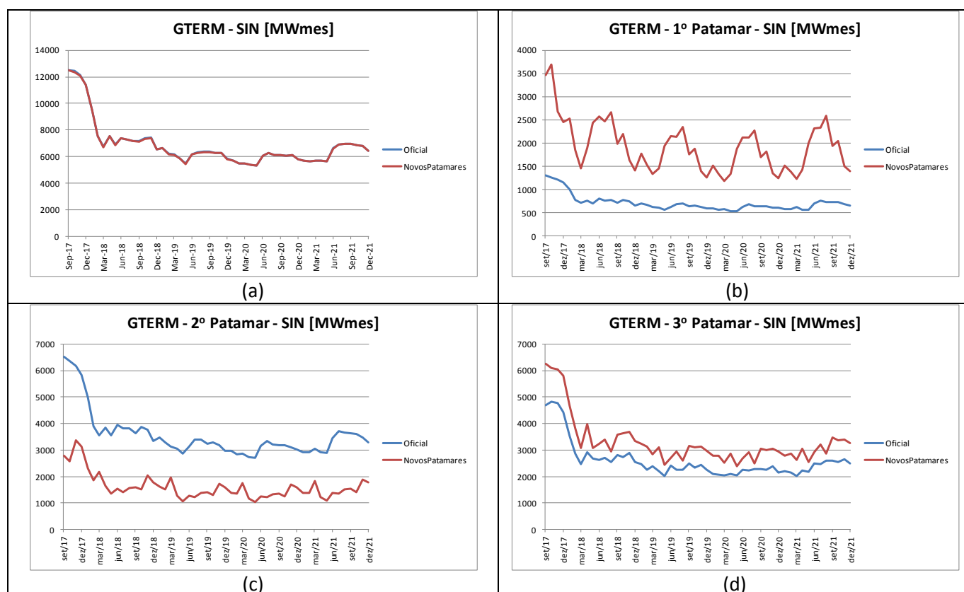
Figura 75 – Evolução temporal da geração térmica do SIN: (a) média; (b) patamar de carga pesada; (c) patamar de carga média; e (d) patamar de carga leve – PMO Set/2017
