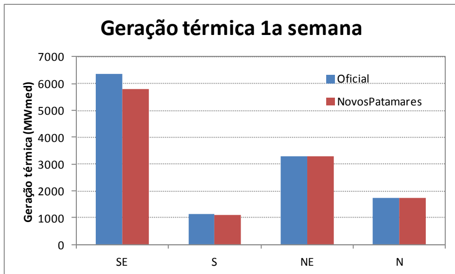
Figura 89 – Geração térmica da 1ª semana por submercados – PMO Set/2017
