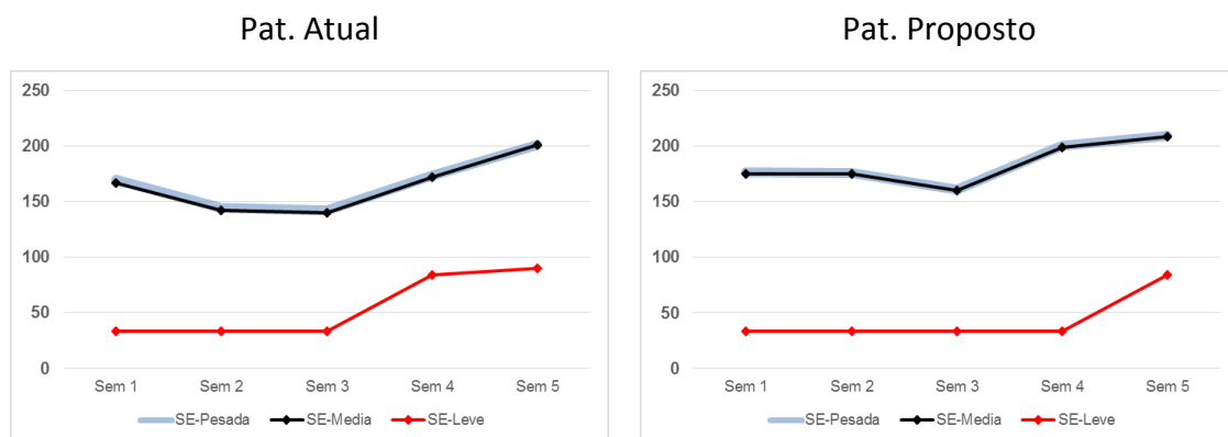
Figura 61 - Comparação PLD Sudeste – junho/2017
