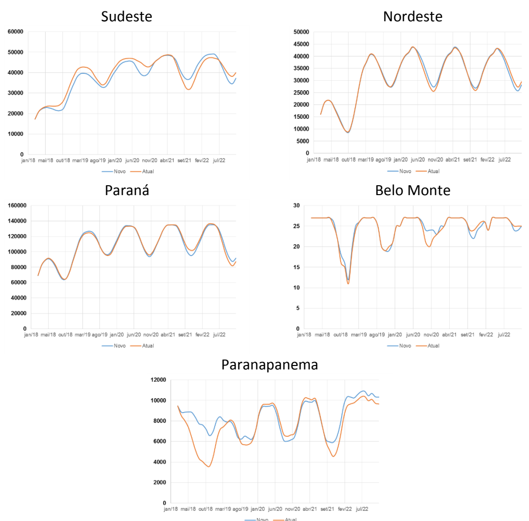
Figura 45 - Evolução temporal da energia armazenada final dos REE's selecionados – PLD março/2018
