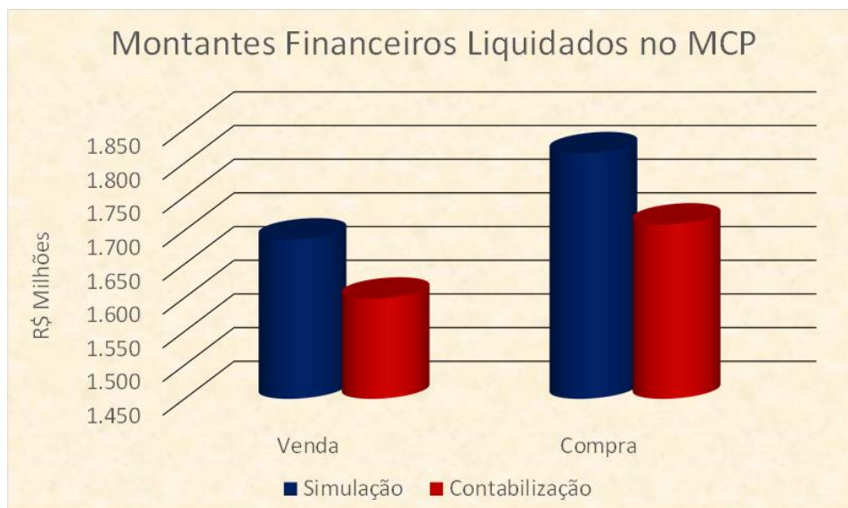
Figura 96 – Montantes liquidados no MCP
