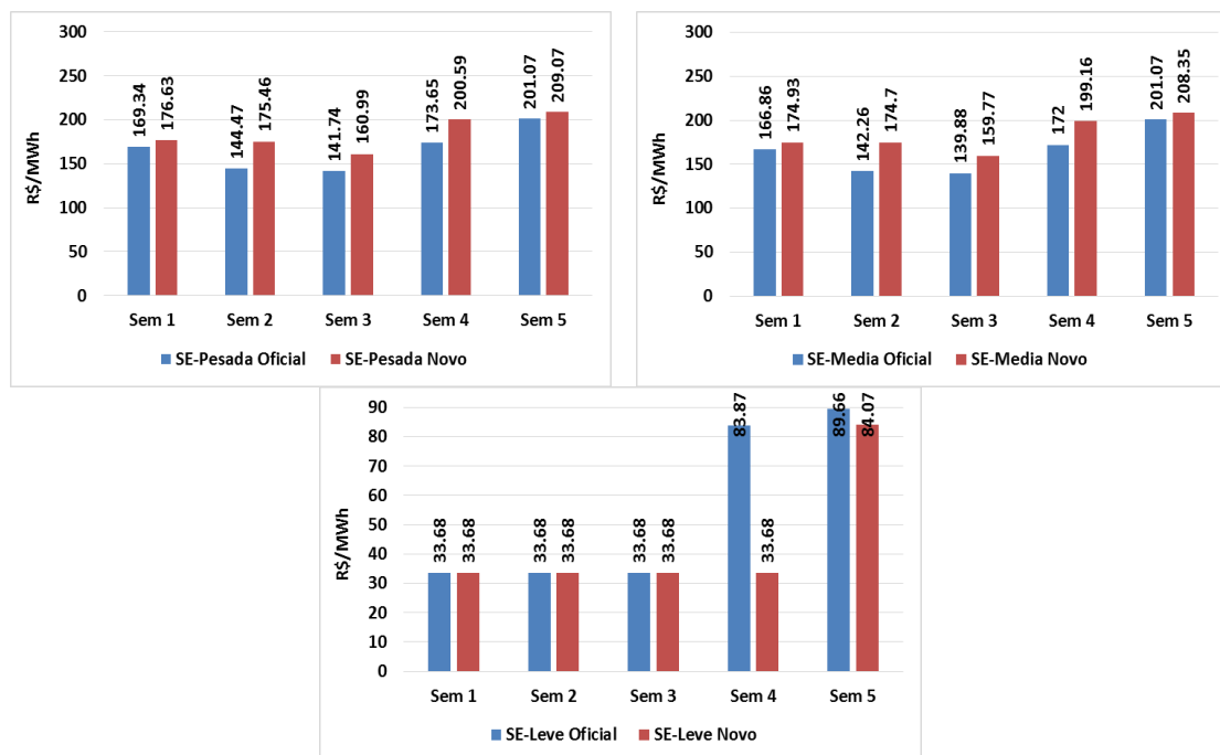
Figura 59- PLD Jun/2017 RV0 – Sudeste
