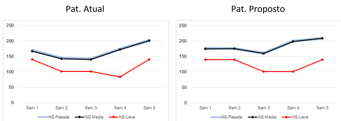
Figura 62 - Comparação PLD Nordeste – junho/2017
