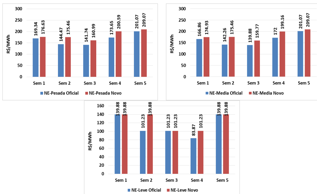
Figura 60- PLD Jun/2017 RV0 – Nordeste
