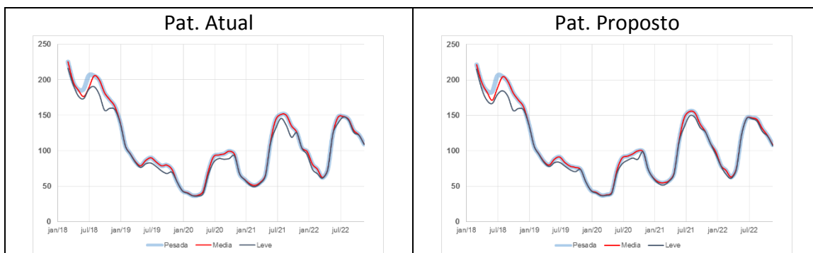
Figura 42- Evolução temporal do CMO do Sul – PLD março/2018
