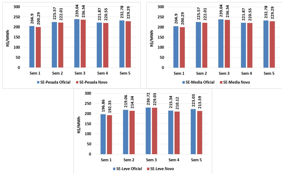
Figura 48 – PLD Mar/2018 RV0 – Sudeste
