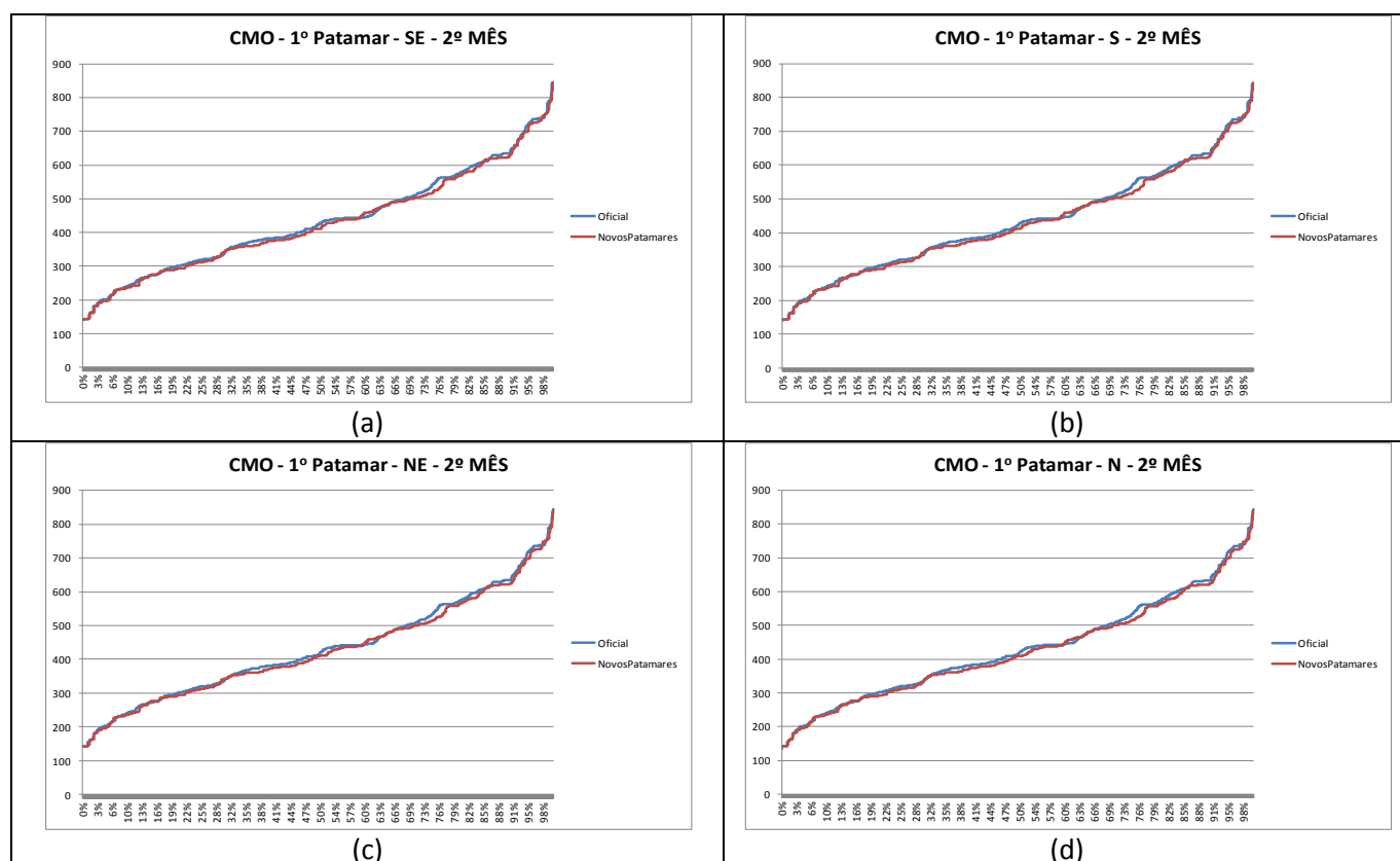
Figura 68 – Curva de permanência do CMO do patamar de carga pesada dos submercados: (a) Sudeste; (b) Sul; (c) Nordeste; e (d) Norte – PMO Set/2017
