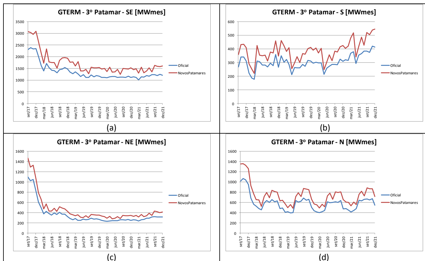
Figura 74 – Evolução temporal da geração térmica para o patamar de carga leve dos submercados: (a) Sudeste; (b) Sul; (c) Nordeste; e (d) Norte – PMO Set/2017
