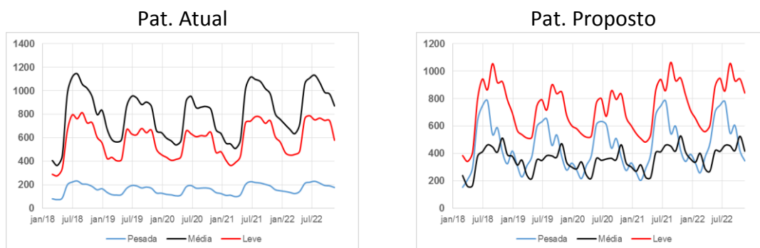
Figura 47- Evolução temporal da geração térmica total final dos REE's selecionados – PLD março/2018
