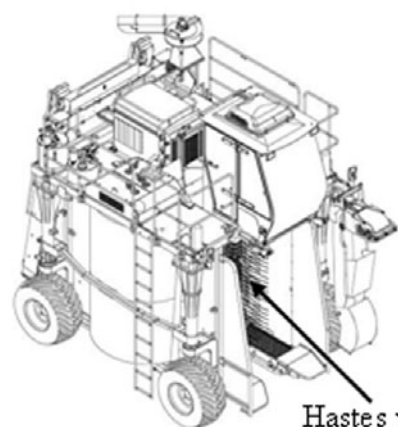
Colhedora de cana-de-açúcar: equipamento que permite a colheita de cana de modo uniforme, por possuir sistema de corte de base capaz de cortar a cana-de-açúcar acompanhando o perfil do solo. Possui um sistema de elevador que desloca a cana cortada até a unidade de transbordo.
