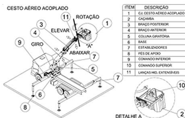
FIGURA 1: EXEMPLO DE ARRANJO COM CESTO ACOPLADO
