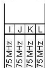
Figura 3. Ilustração da segmentação da faixa de 31,00 GHz a 31,30 GHz em blocos de 75 MHz. (Frequências em GHz)
