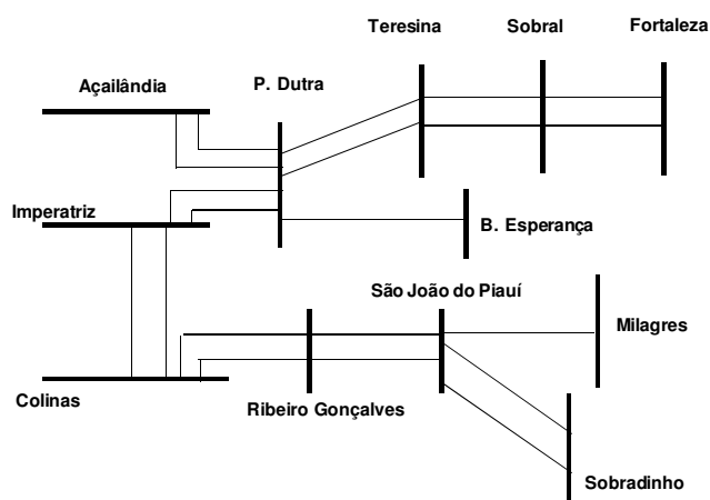
Figura 12 – Diagrama esquemático da interligação Norte – Nordeste – 2010
