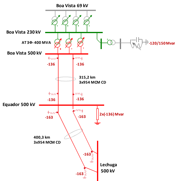
Figura 18 – Interligação Boa Vista - Manaus – Unifilar
