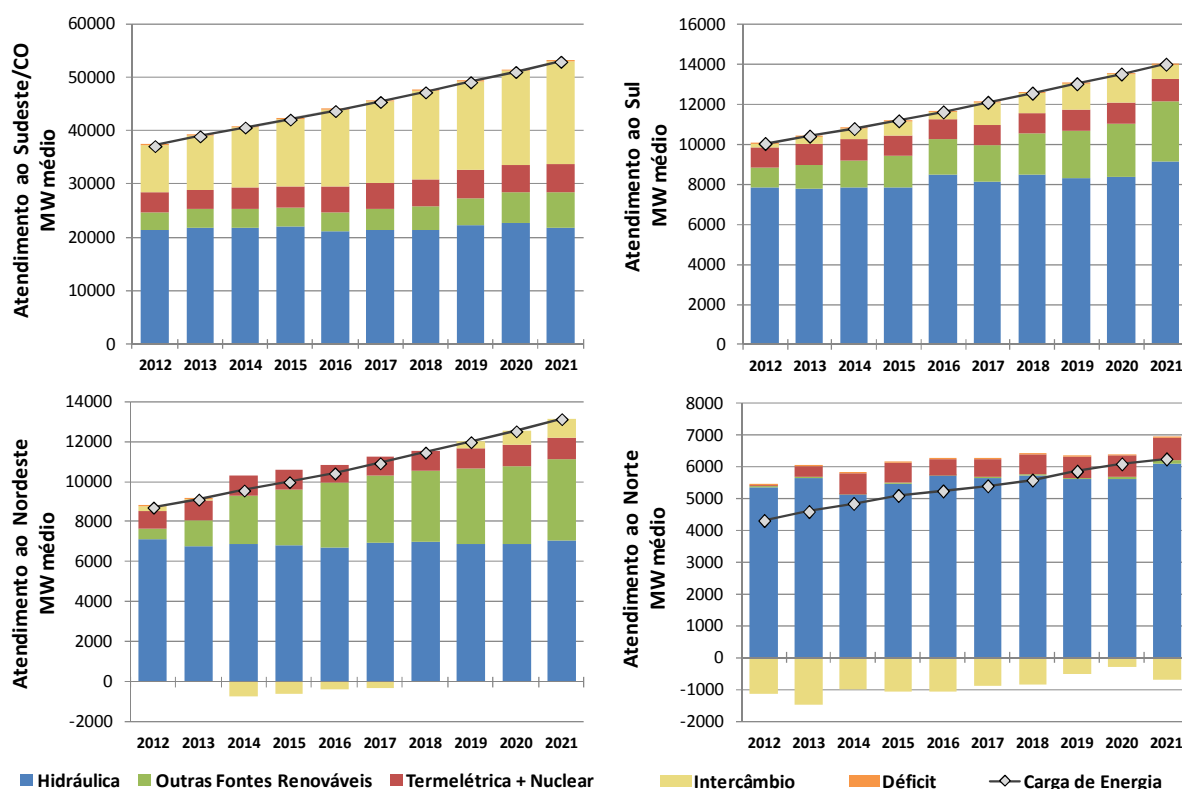
Gráfico 43 – Geração hidrotérmica por subsistema - média dos 2.000 cenários hidrológicos (MWmed)
