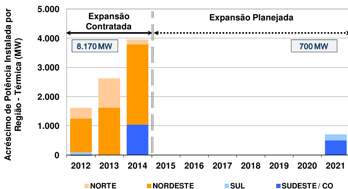
Gráfico 24 – Acréscimo de capacidade instalada termelétrica (MW)
