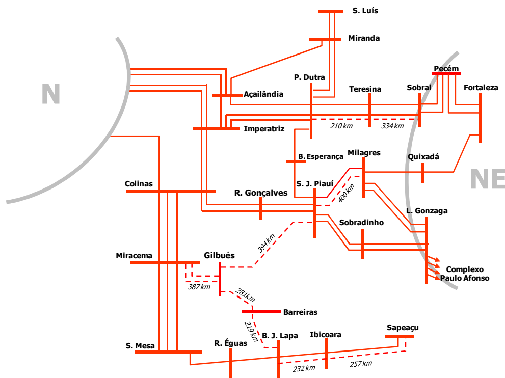
Figura 13 – Reforços indicados para aumentar a capacidade de exportação da região Nordeste para a região Sudeste
