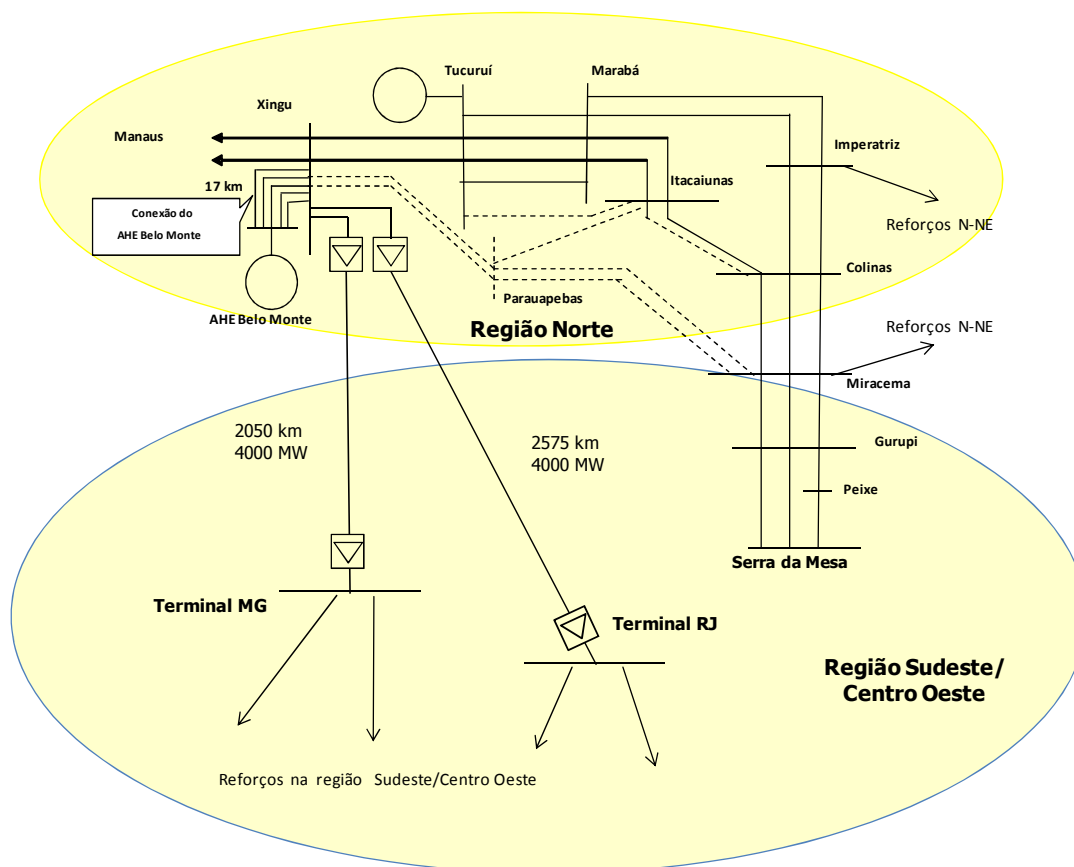
Figura 11 – Reforços na interligação Norte-Sudeste
