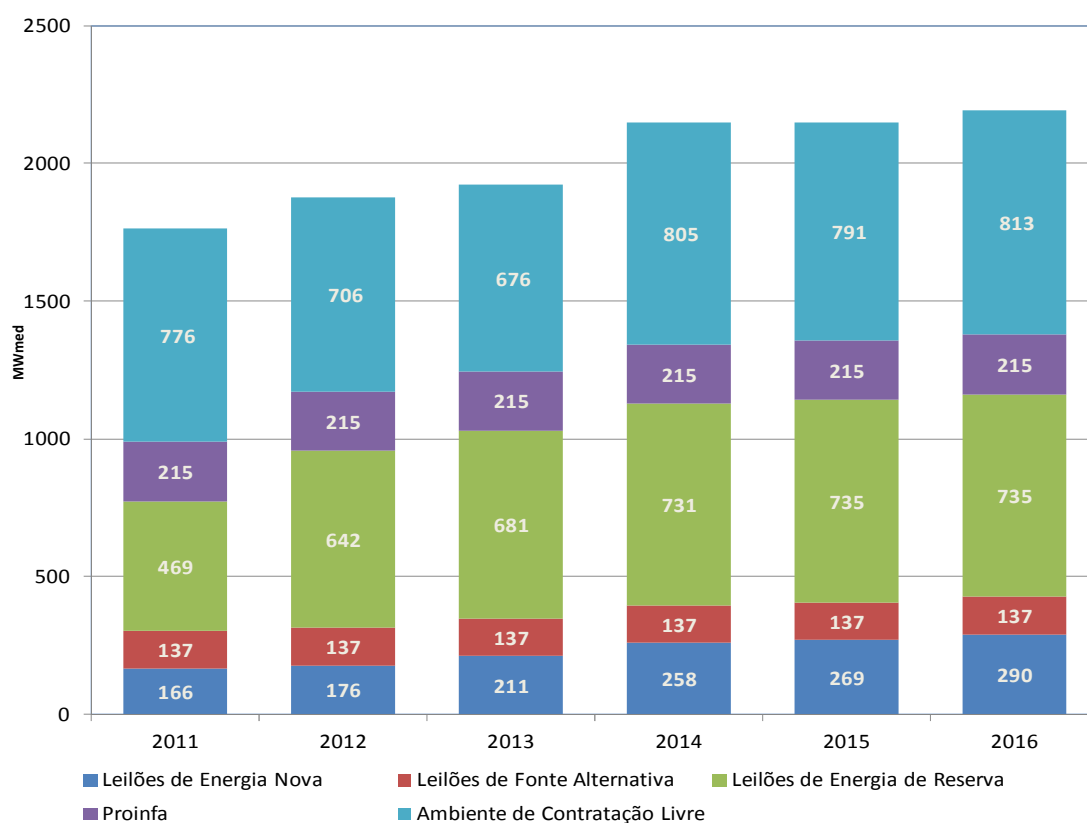
Gráfico 129 – Energia contratada e comercializável - usinas sucroenergéticas vencedoras dos leilões
