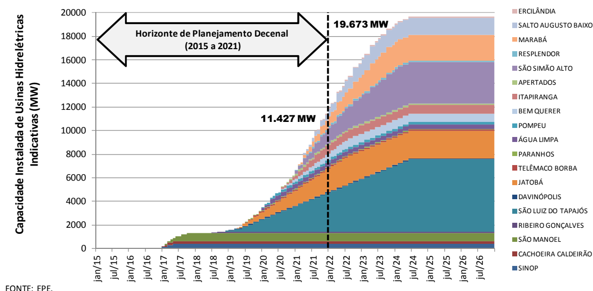
Gráfico 20 – Evolução da capacidade instalada de hidrelétrica indicativas (MW)
