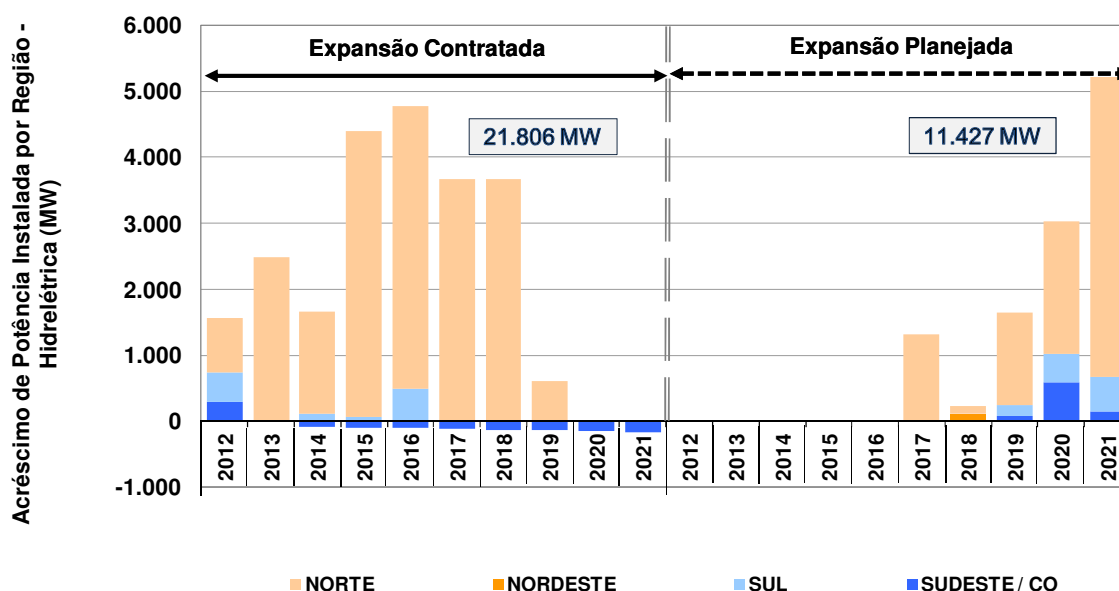
Gráfico 21 – Acréscimo da capacidade instalada hidrelétrica (MW)
