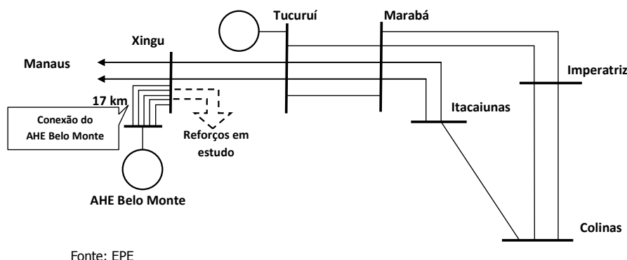
Figura 8 – Conexão do AHE Belo Monte na SE Xingu 67
