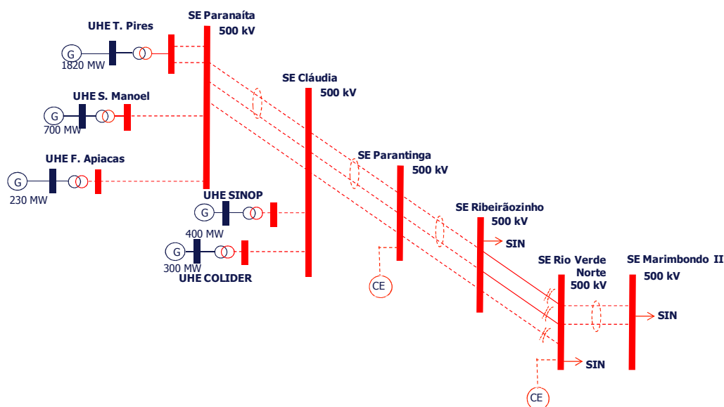
Figura 9 – Diagrama unifilar simplificado do sistema de transmissão para escoamento das usinas do Rio Teles Pires
