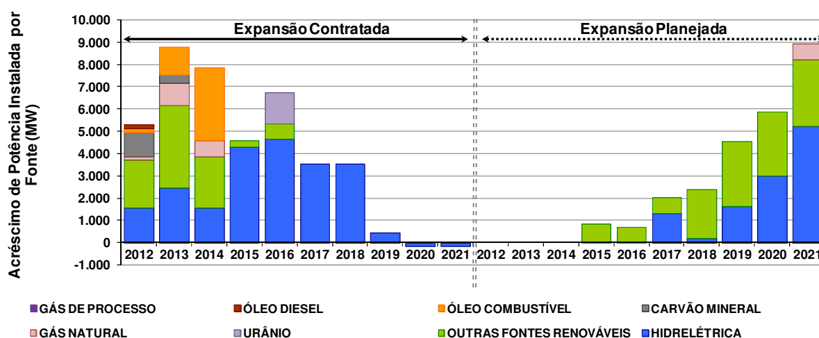
Gráfico 31 – Acréscimo de capacidade instalada anual por fonte (MW)
