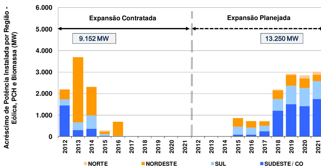
Gráfico 27 – Acréscimo de capacidade instalada de outras fontes renováveis (MW)
