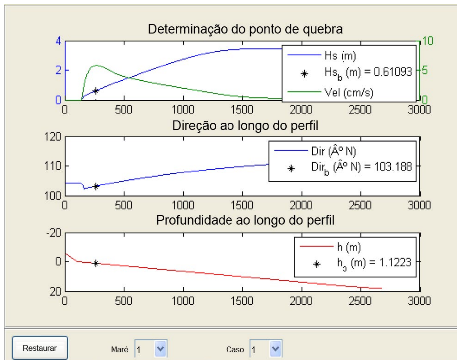
Figura 44: Evolução dentro da área de arrebentação em um perfil definido (o asterisco indica o ponto de velocidade máxima e, portanto, o de quebra).
