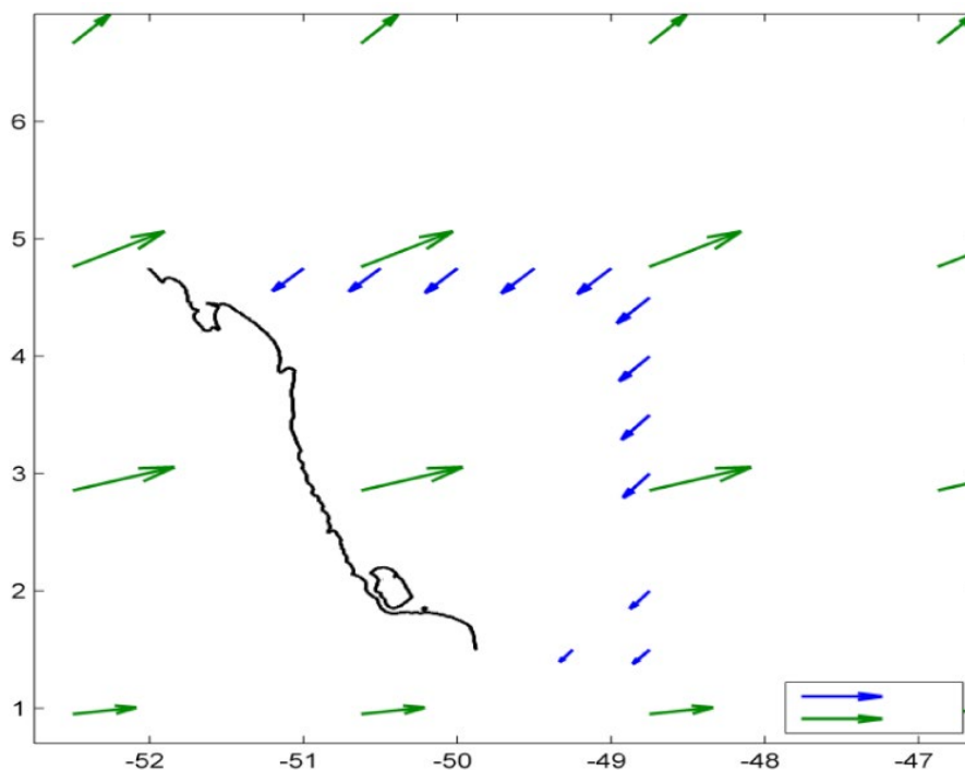
Figura 13: Condições de ondas e vento na malha de propagação 1. Em azul a magnitude e direção da altura significativa de onda ( H_s ) e em verde a magnitude e direção do vento. Escala: H_s (em m) e vento (em m/s) .
