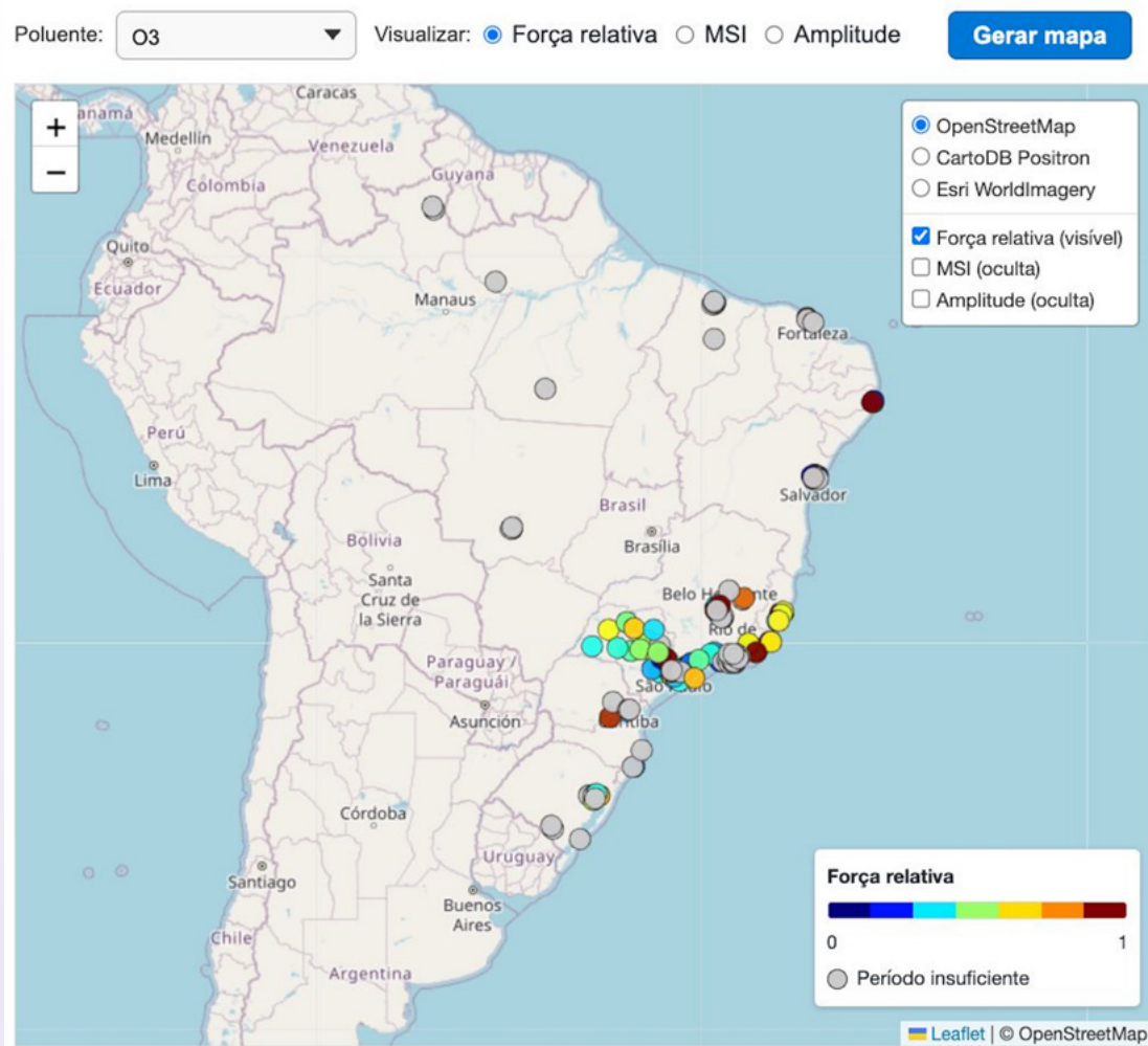
Figura 35 - Mapa interativo da sazonalidade de CO, NO 2 , SO 2 , MP 2,5 , MP 10 e O 3 no Brasil.
