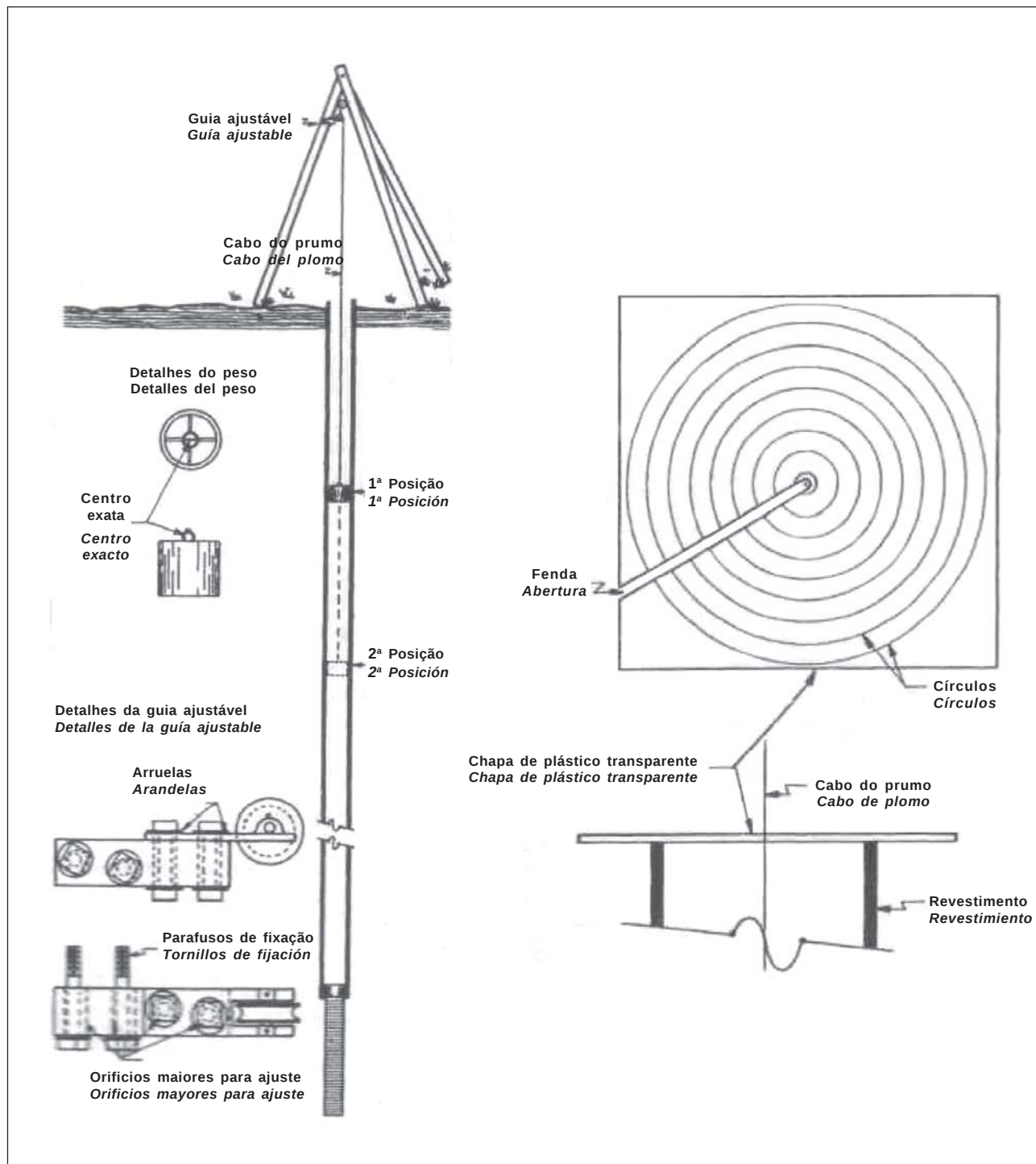
Figura 25.- Esquerda, Disposição típica para a verificação da verticalidade e alinhamento de um poço; Direita, A chapa de plástico com círculos concêntricos colocada sobre o revestimento auxilia a medida do afastamento. Fonte: Água Subterrânea e Poços Tubulares – Johnson Screens – 3ª edição. – Cetesb – SP
