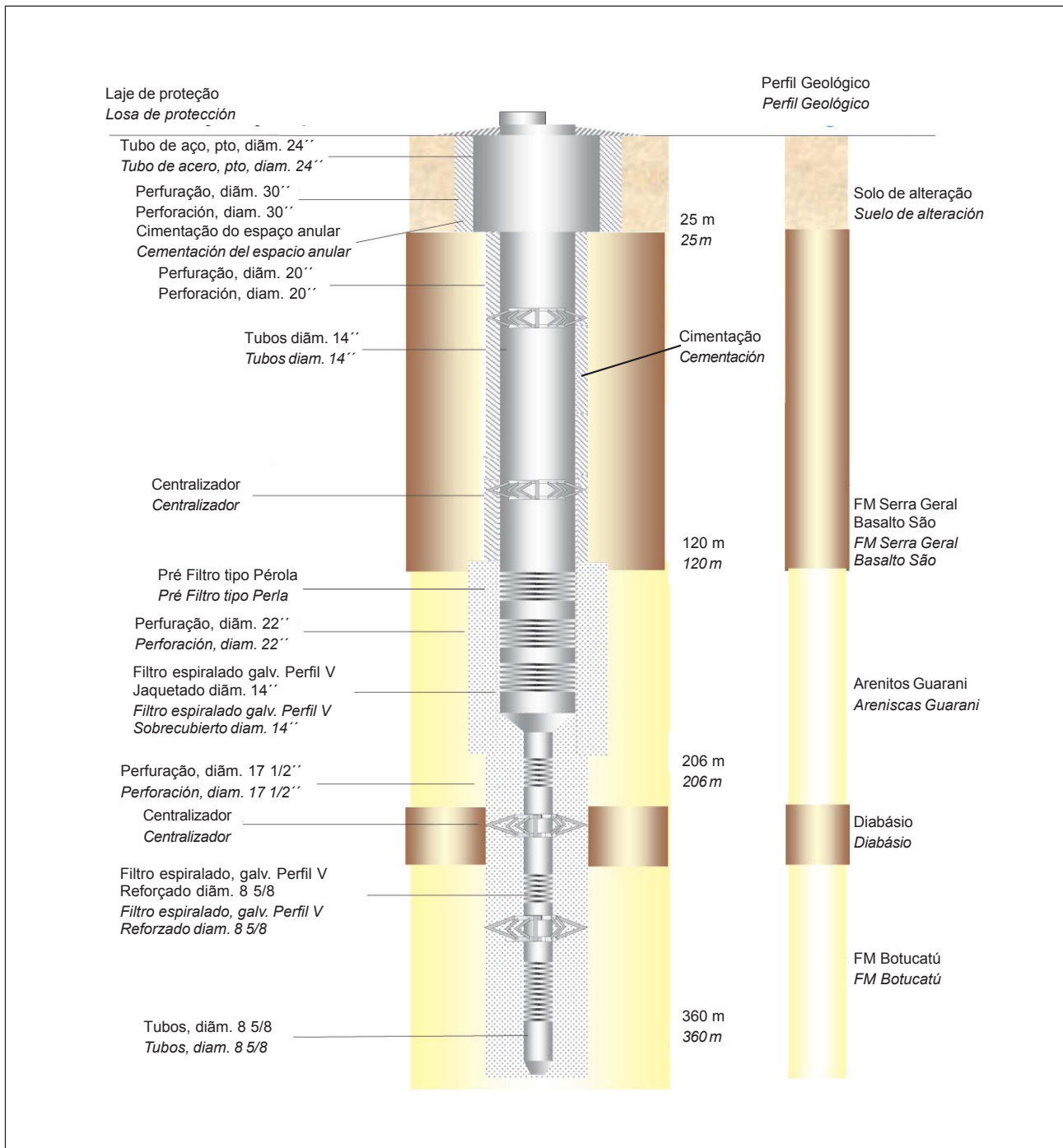
Figura 18.- Projeto Tipo Guaraní – mostrando relação de diâmetros de perfuração e coluna de revestimentos e também filtros espiralados. Coluna dotada de centralizadores com isolamento do basalto.
