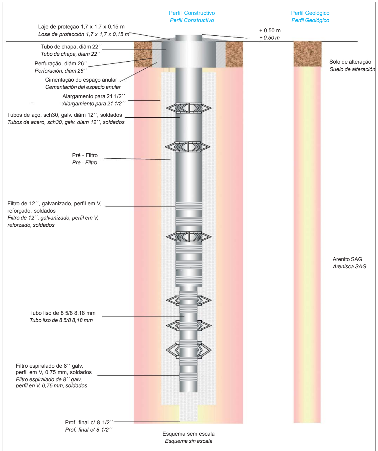
Figura 3.- Projeto esquemático de um poço tubular profundo em área de afloramento do SAG
