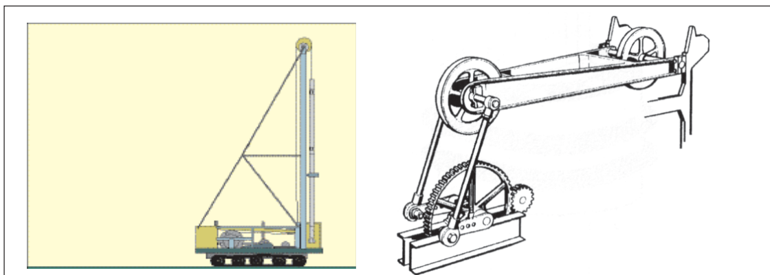
Figura 21.- Esquema de sonda percussora com balancim
