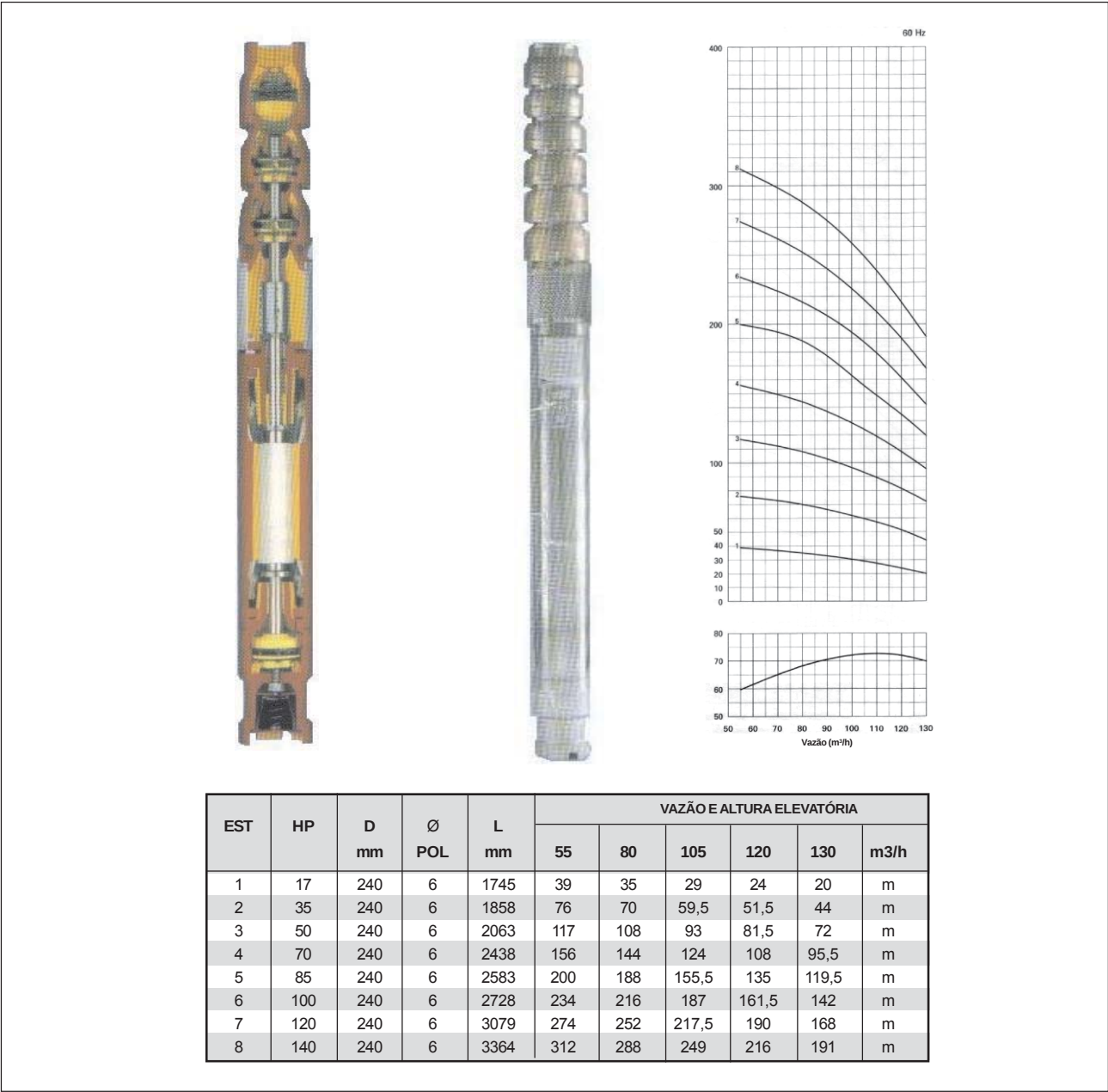
Figura 22.- Grupo Moto Bomba Submersa – modelo de curva de rendimento de um equipamento e tabela analítica produção e altura manométrica total
