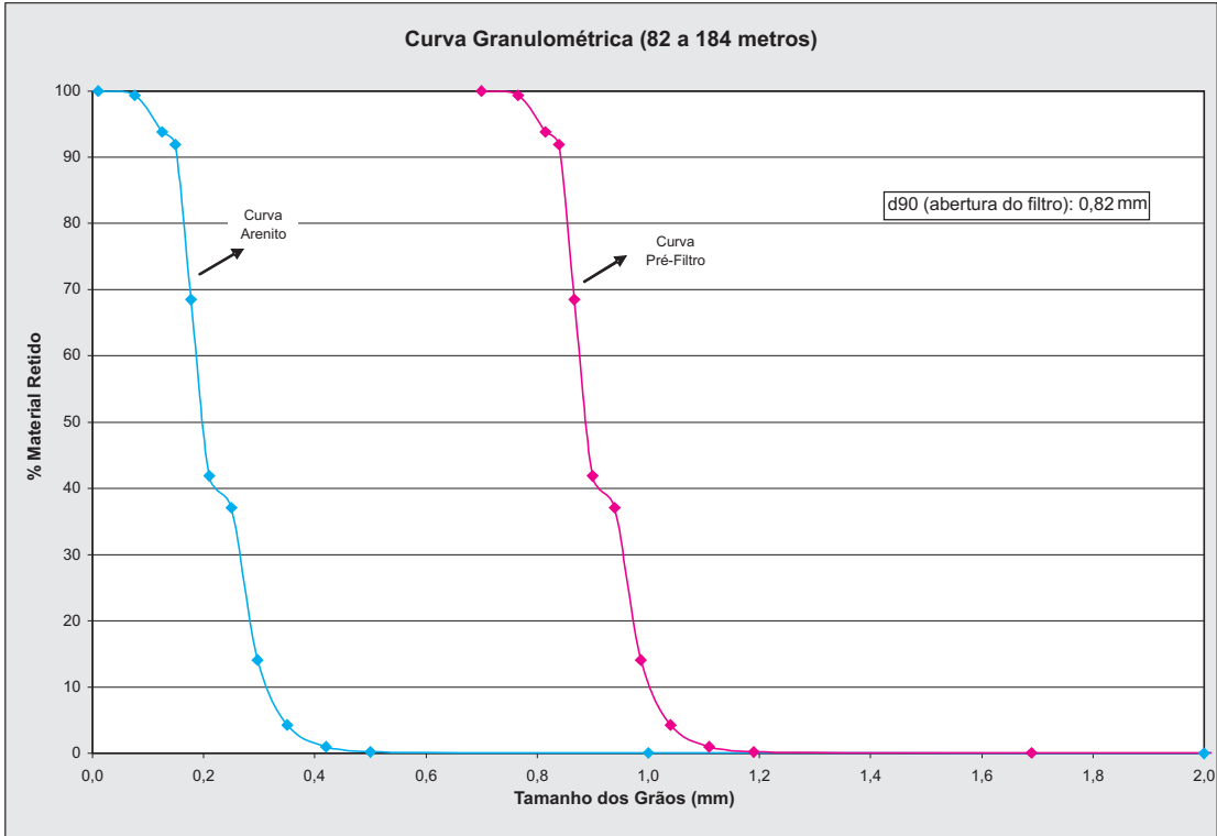
Figura 15.- Curva granulométrica de um poço no Aquífero Guarani com a curva de seleção de pré-filtro.
