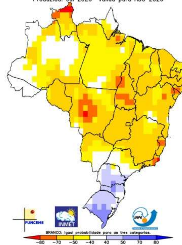
Multi-modelo CPTEC/INMET/FUNCCE Probab. tercil mais provavel: Precip. (%) Produzida: Jul 2026 Valida para ASO 2026
