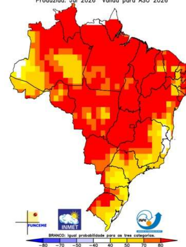
Multi-modelo CPTEC/INMET/FUNCCE Probab. tercil mais provavel: Temp. 2m (%) Produzida: Jul 2026 Valida para ASO 2026
