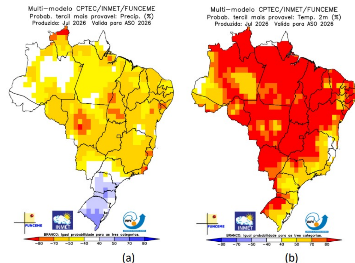
Figura 3: Previsão climática sazonal por tercil (categorias abaixo da faixa normal, dentro da faixa normal e acima da faixa normal), gerada pelo método objetivo (CPTEC/INPE, INMET e FUNCCEME). As áreas em branco indicam igual probabilidade para as três categorias. (a) precipitação; (b) temperatura.
