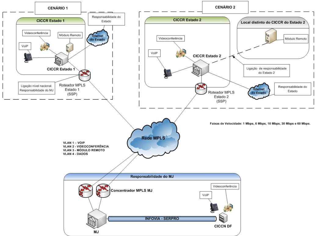
Topologia SENASP
