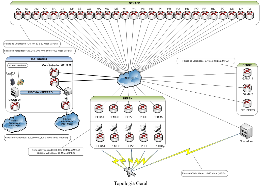
Topologia Geral
