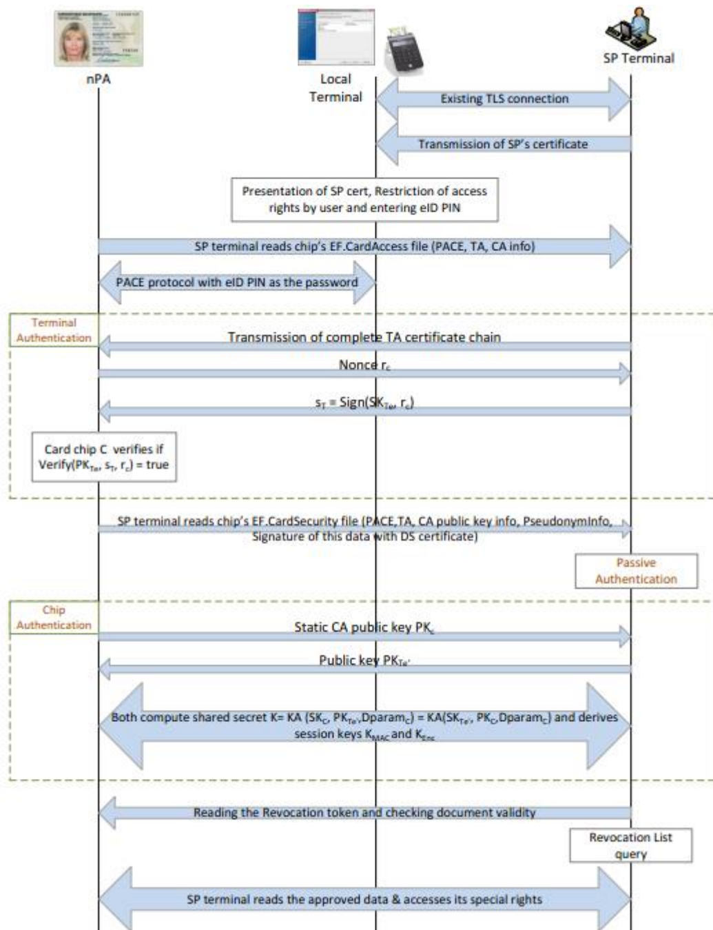
Figura 5.9 (tirada de [19]): Sequência de execução dos protocolos de autenticação para função eID do nPA.
