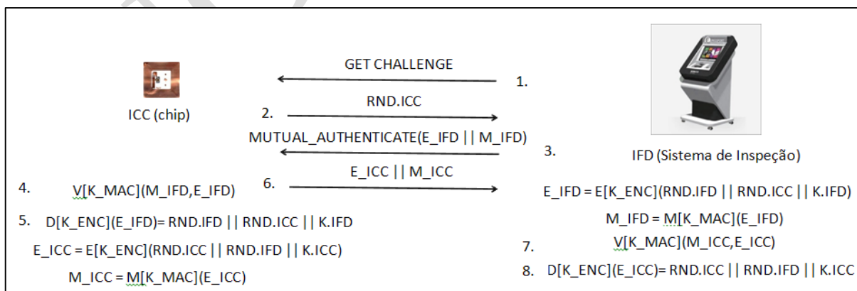
Figura 3.9: Protocolo desafio-resposta do BAC.
