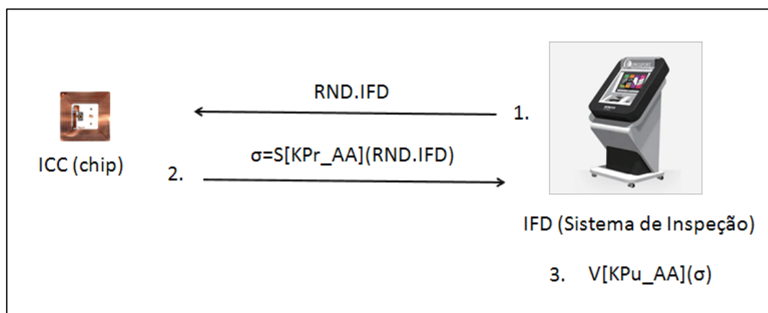
Figura 3.6: Protocolo de autenticação ativa simplificado.
