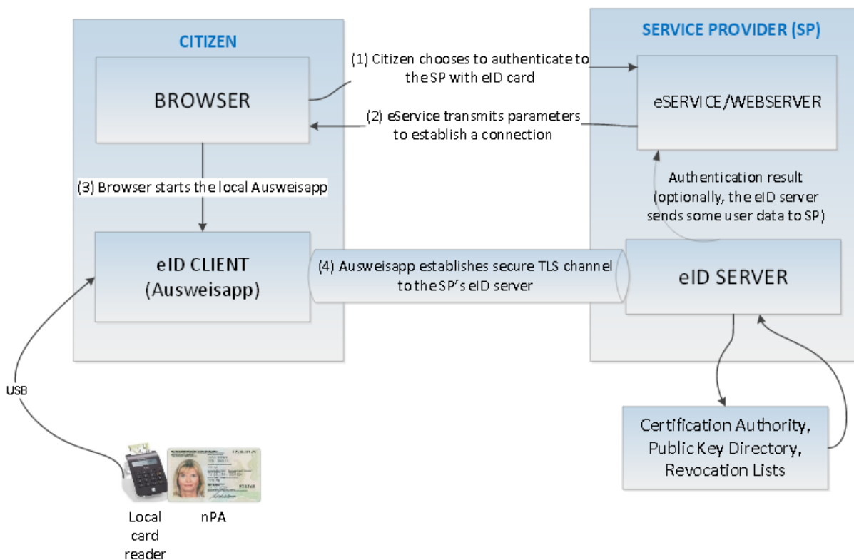
Figura 5.8 [tirada de [19]]: Procedimento de autenticação online do nPA.
