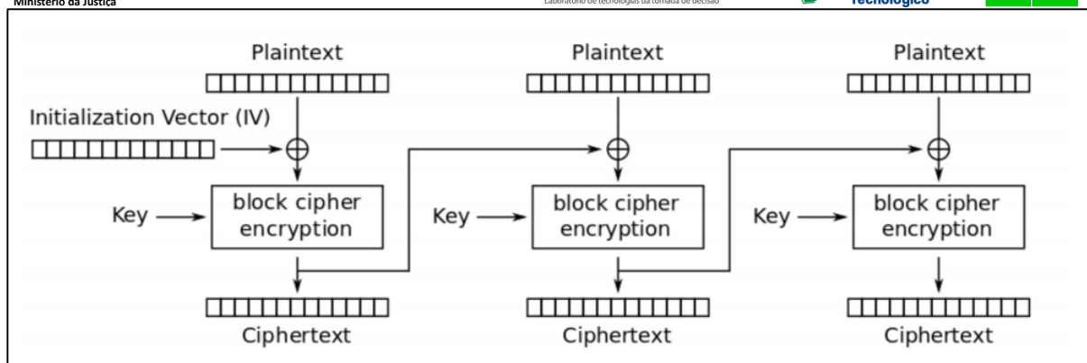
Figura 3.10. Modo de cifragem CBC.
