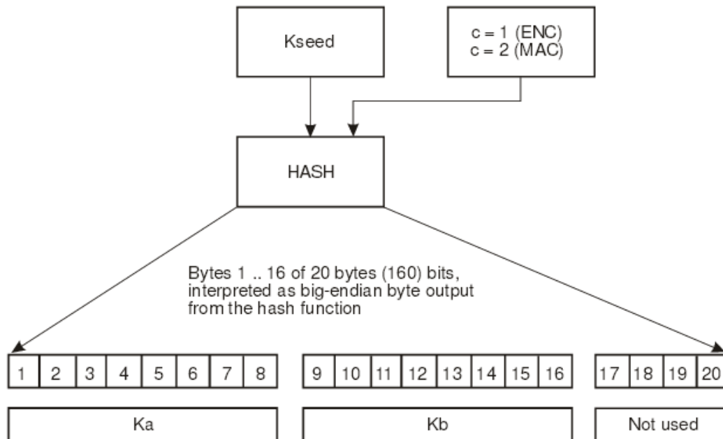
Figura 3.8 (tirada do DOC 9303 da ICAO [2]): Formação de Chaves de Acesso Básico.
