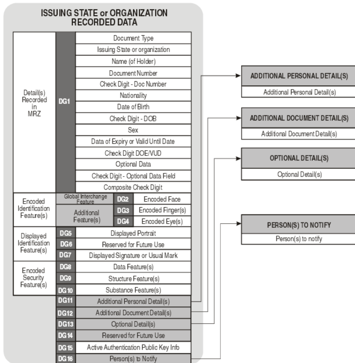
Figura 3.3 (tirada do DOC 9303 da ICAO [2]): LDS.
