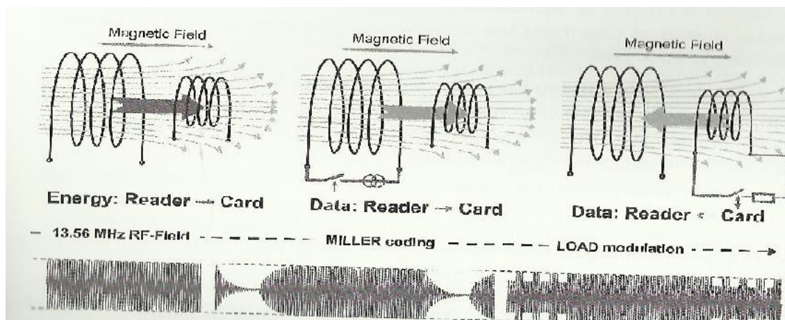
Fig.4 - Transmissão de dados do chip "sem-contato" [1]
