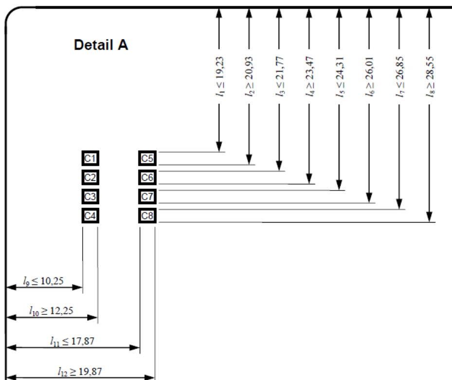
Fig.8 - Localização dos contatos
