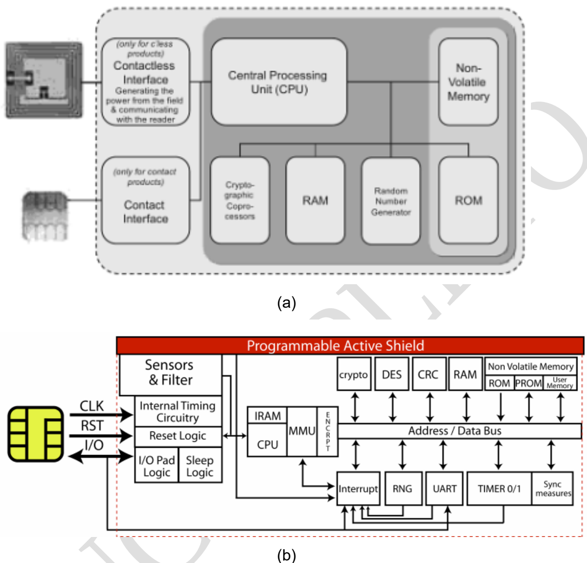
Fig. 2 - Blocos funcionais de um chip de eID (a) [1], e componentes de segurança como sensores e MMU (b) [15]
