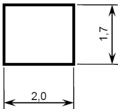
Fig.7 - Mínimas dimensões do contato (em milímetros)
