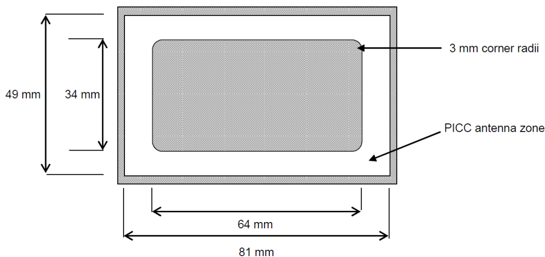
Fig.6 - Dimensões físicas dos cartões PICC
