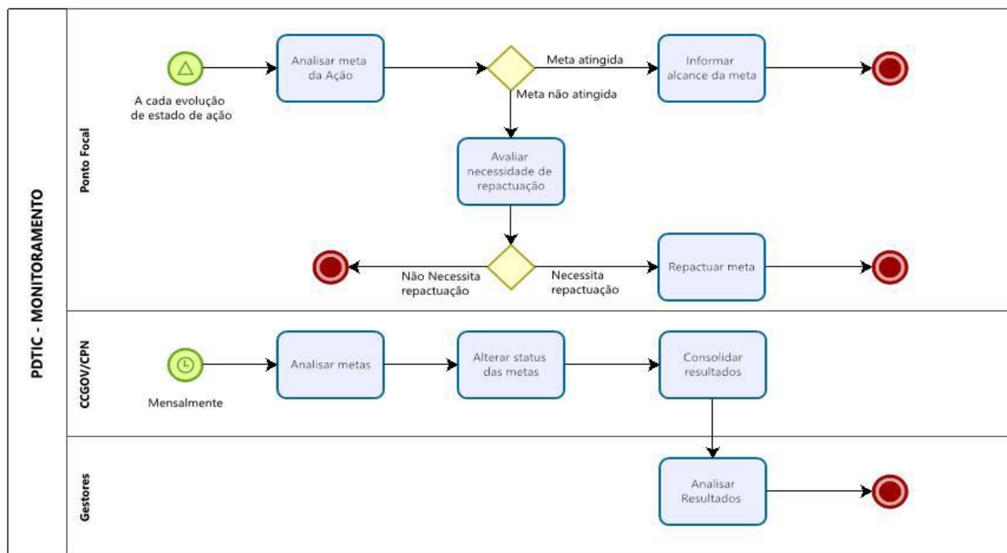
Figura 14 – Fluxo de Monitoramento do PDTIC
