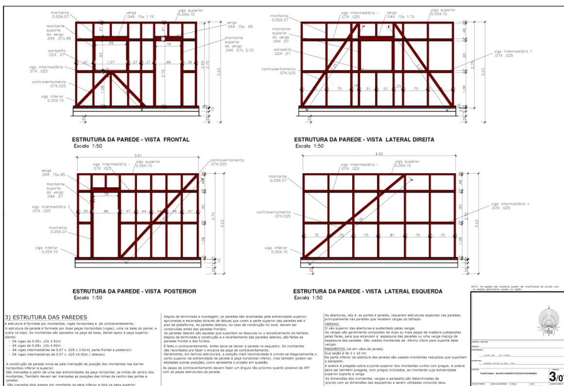
FIGURA 9 – PROCESSO CONSTRUTIVO DOS ABRIGOS MÓVEIS
