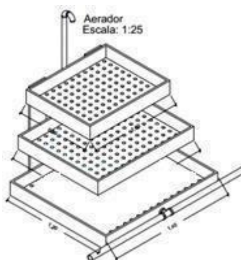
Figura 11: Desenho esquemático do aerador que compõe a unidade de tratamento.
