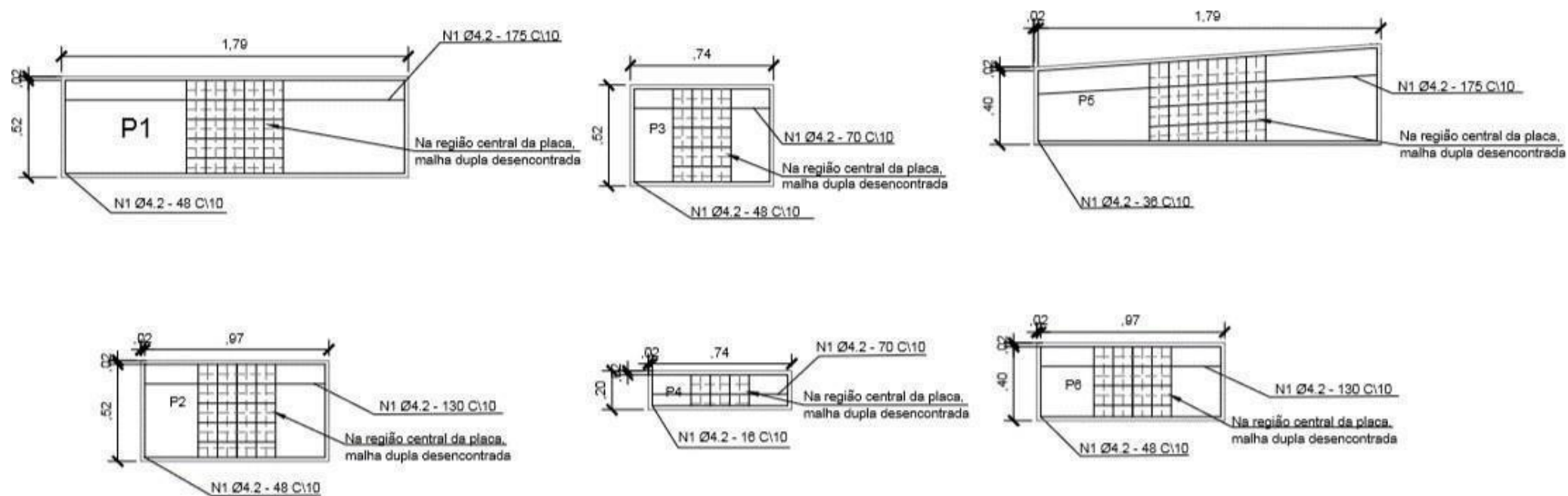
Figura 2: Descrição da malha de ferro
