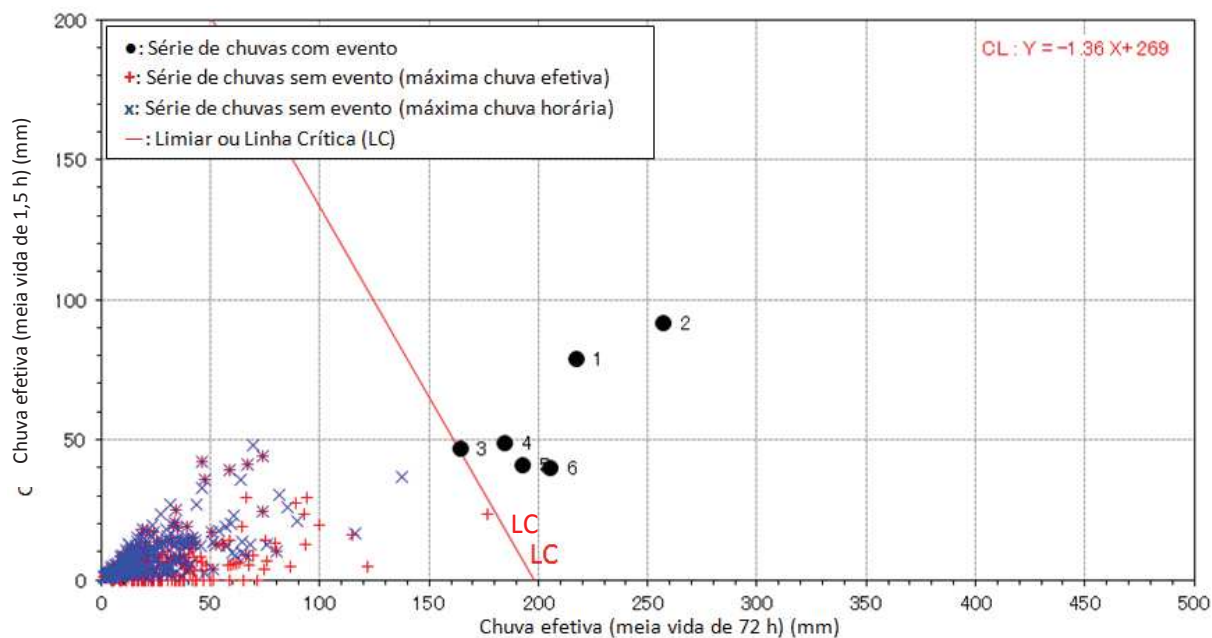
Figura 20: Limiar para o Município de Nova Friburgo (Bloco Noroeste) - Método Compartilhado
