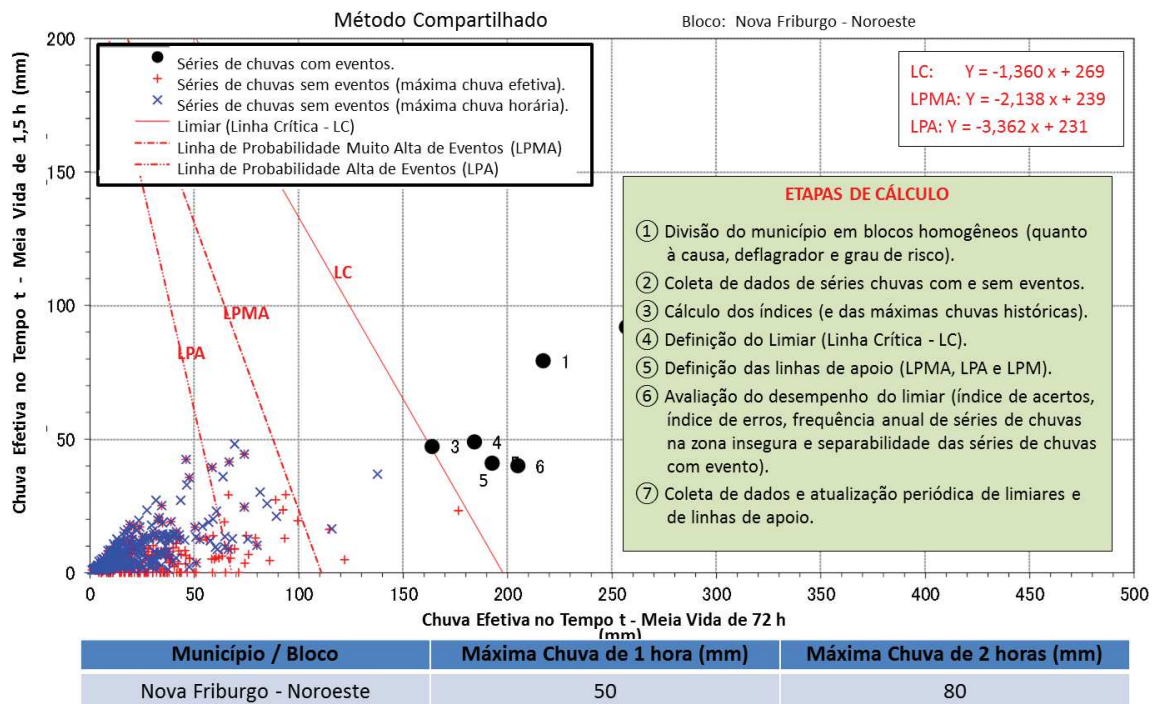
Figura 9: Representação esquemática do Método Compartilhado
