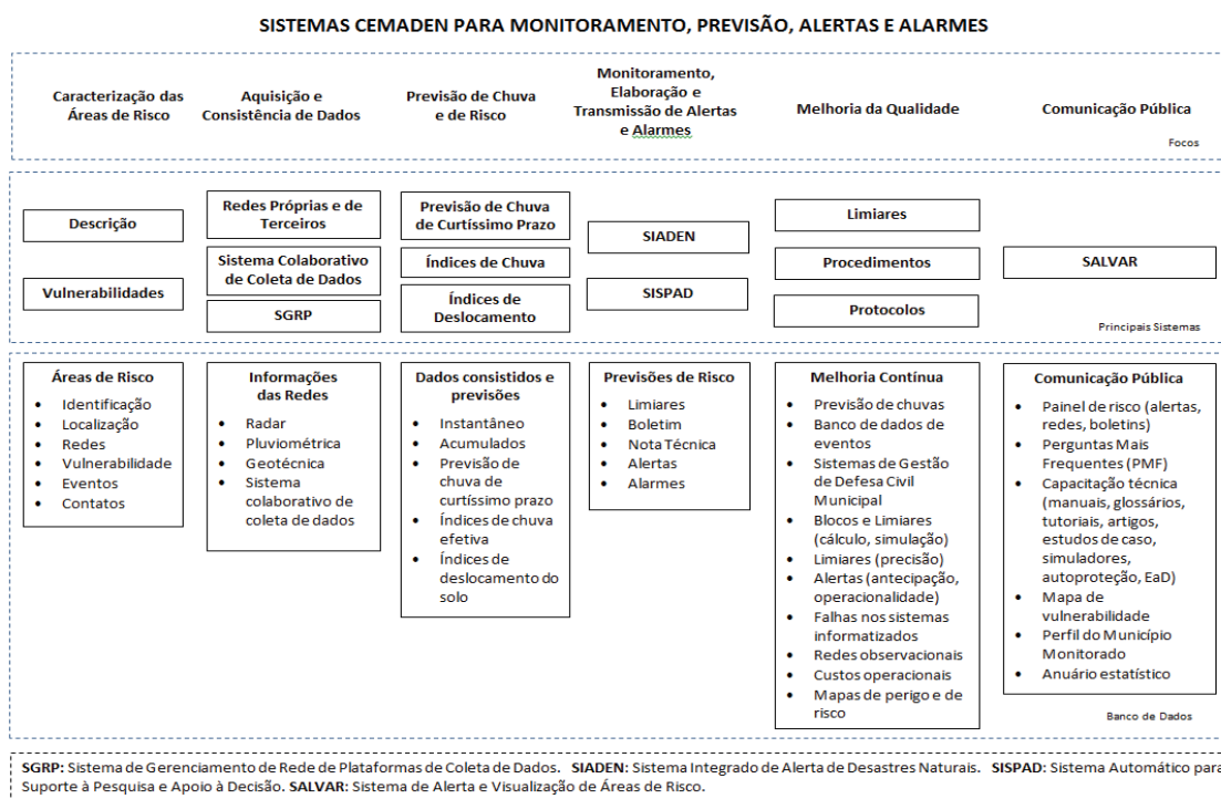
Figura 35: Sistemas informatizados para monitoramento, previsão, alertas e alarmes
