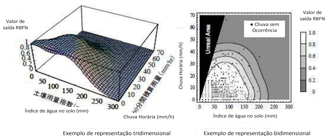
Figura A5: Estabelecimento do limiar pelo Método da Análise RBFN
