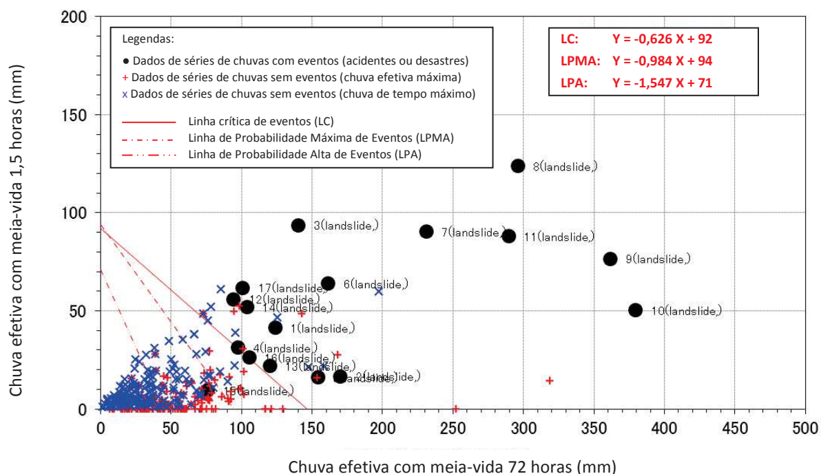
Figura 18: Exemplo de gráfico para cálculo do limiar de movimento de massa (Alto da Independência, Petrópolis - RJ, dados no período 2008 - 2011).
