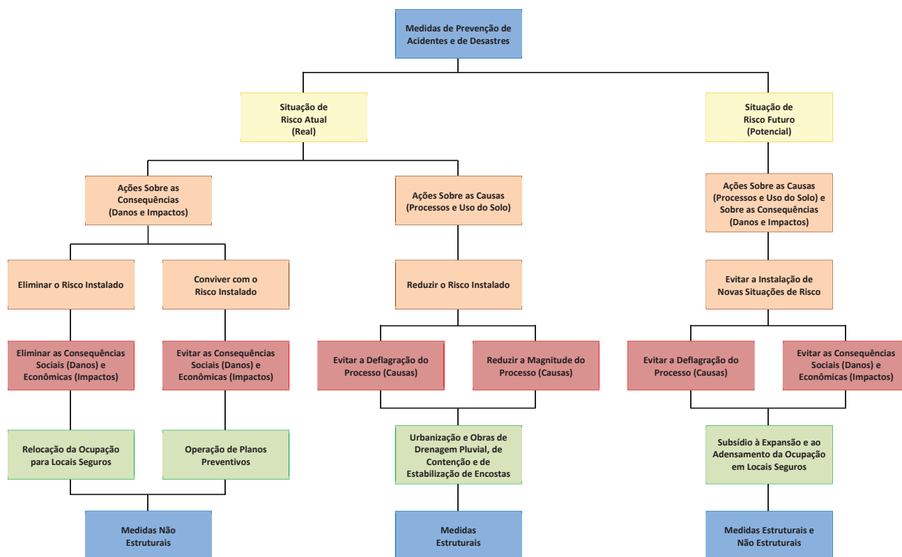
Figura F1: Medidas estruturais e não-estruturais de prevenção de acidentes e desastres naturais
