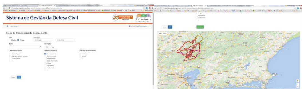
Figura 40: Telas do Sistema de Gestão da Defesa Civil de Petrópolis, RJ
