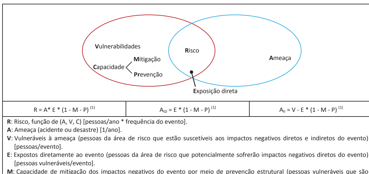
Figura 2: Representação esquemática da equação de risco
