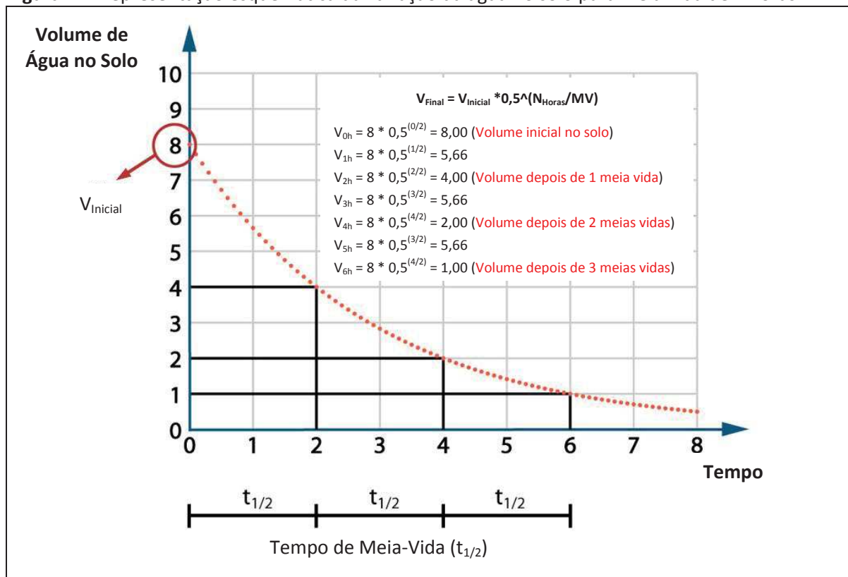
Figura A4: Representação esquemática da variação da água no solo para meia-vida de 2 horas
