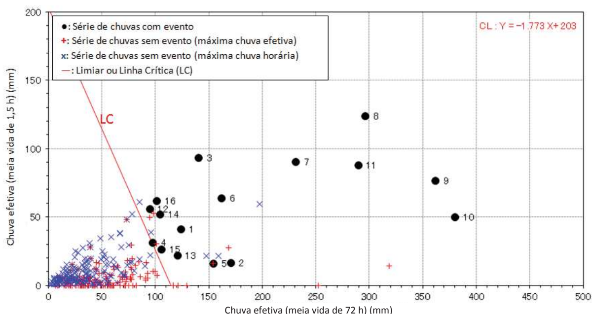
Figura 21: Limiar para o Município de Petrópolis - Método Compartilhado
