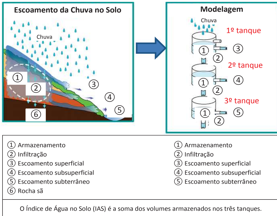
Figura 8: Representação esquemática do Modelo Tanque.
