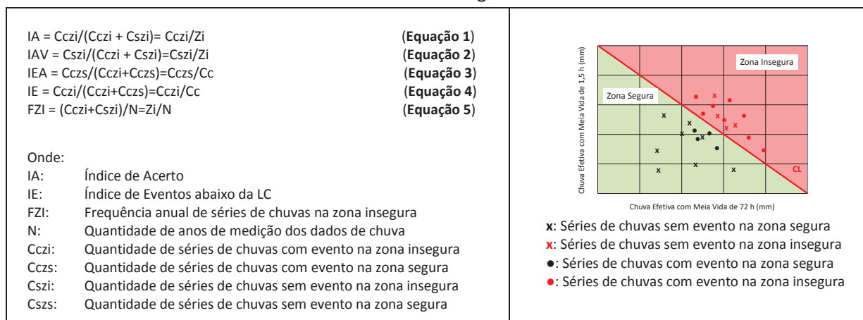
Figura 22: Índice de Acerto, Índice de Eventos abaixo da LC e Frequência Anual de chuvas na Zona Insegura
