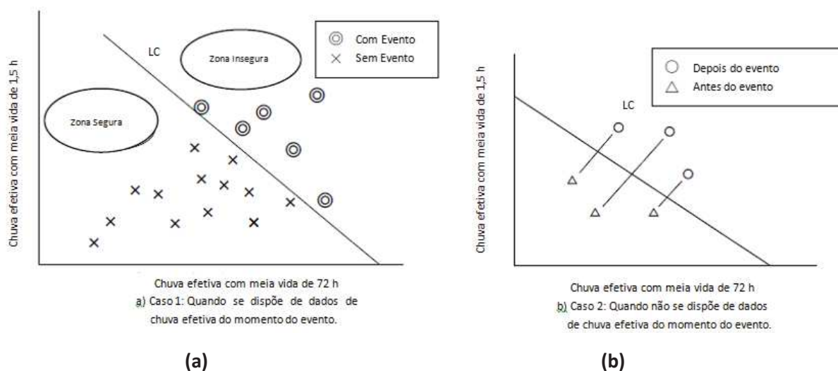
Figura 26: Critérios para o traçado do limiar (Linha Crítica - LC)
