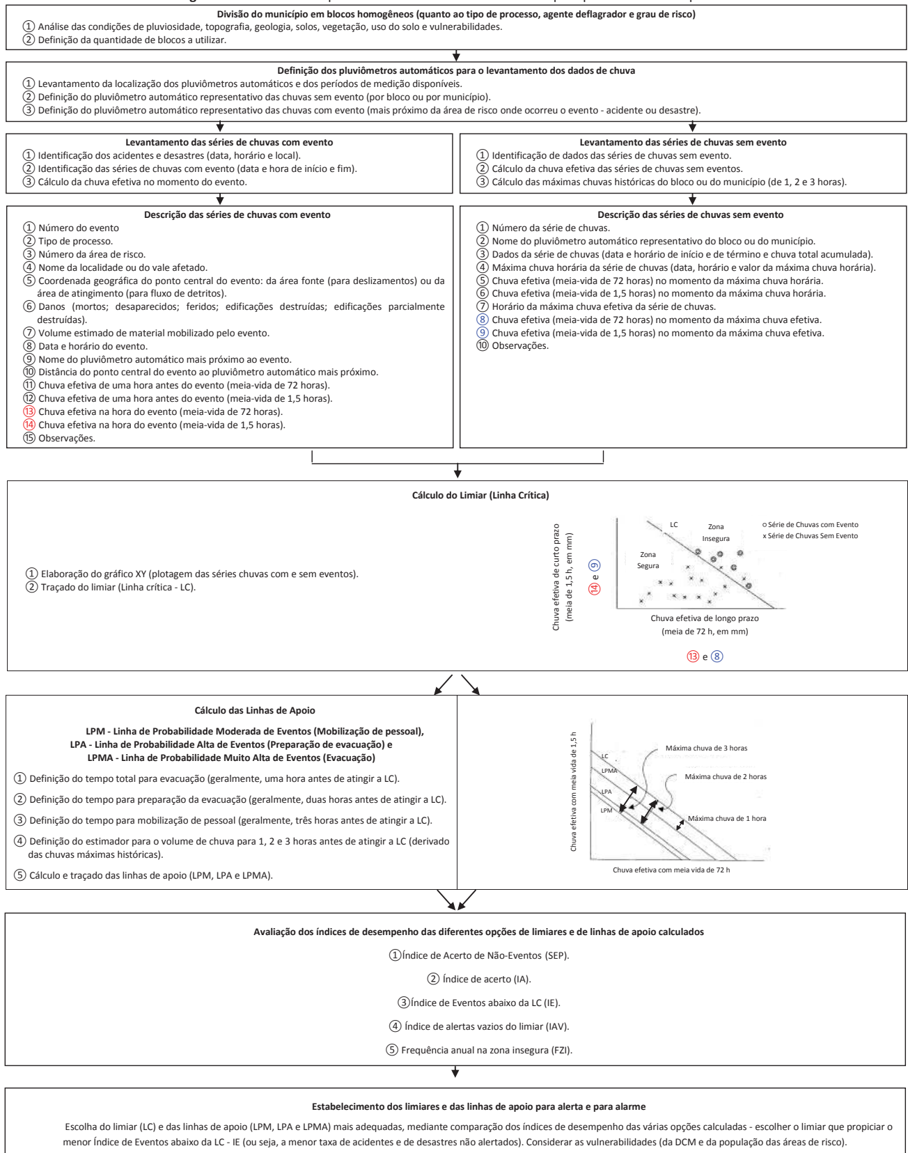
Figura 23: Procedimento para cálculo do limiar e das linhas de apoio pelo Método Compartilhado
