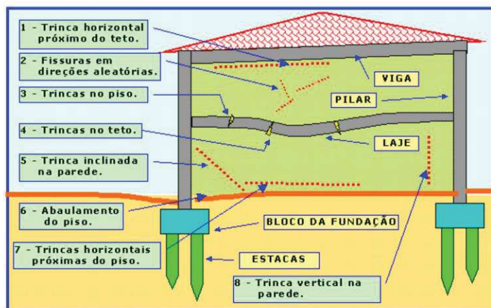
Figura F11: Alguns tipos de trincas e suas causas mais comuns
