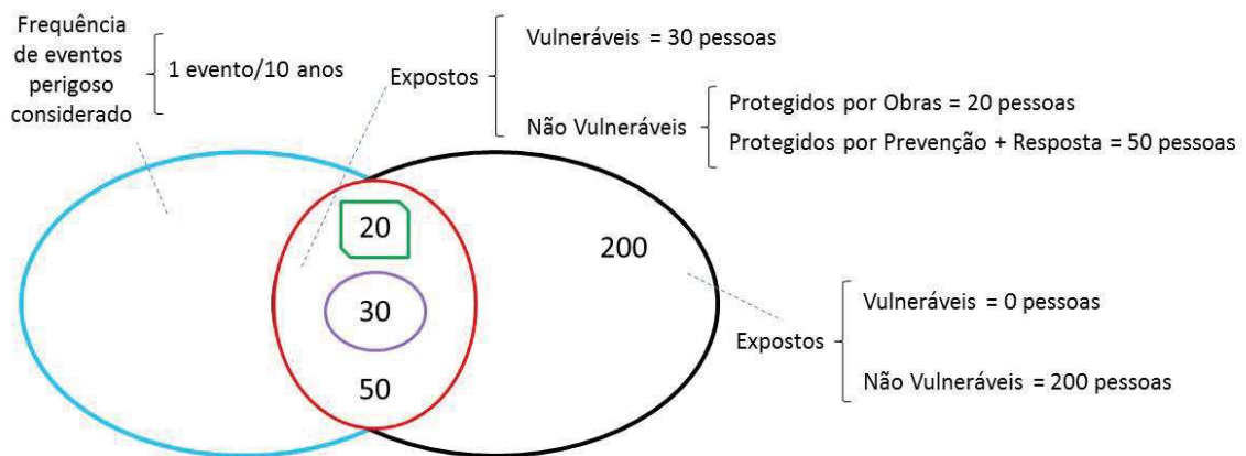
Figura 3: Ilustração de cálculo do risco para um evento hipotético (deslizamento planar, deslizamento rotacional, fluxo de detrito etc.)
