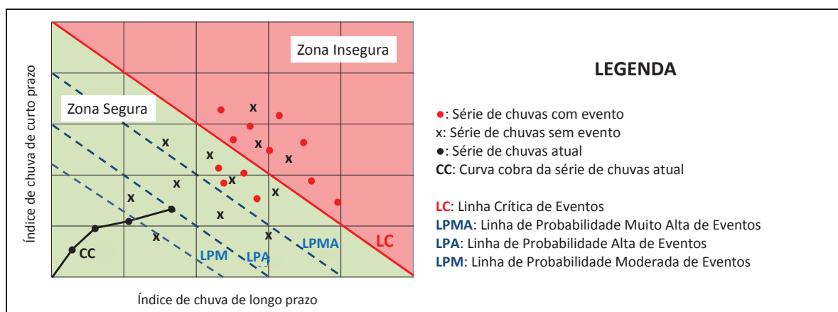
Figura 16: Representação esquemática das séries de chuvas, linhas de referência e curva cobra
