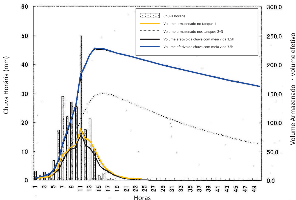
Figura 15: Relação entre o modelo tanque e a chuva efetiva
