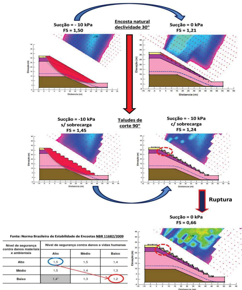
Figura 7: Representação esquemática da análise do Fator de Segurança de uma encosta
