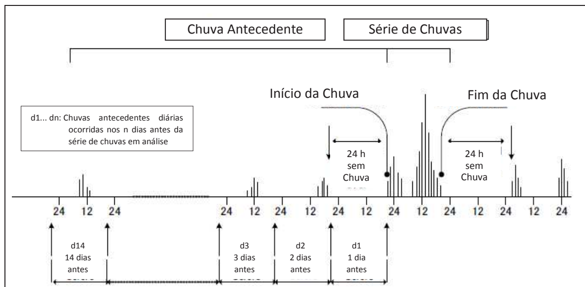
Figura A3: Representação esquemática dos conceitos de série de chuvas e de chuva antecedente
