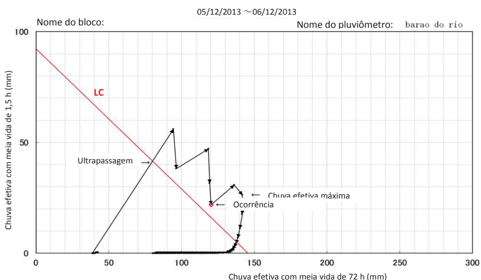
Figura 29: Curva cobra referente aos dados da Tabela 8
