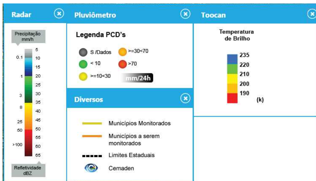
Figura E9: Camadas da aba Legenda
