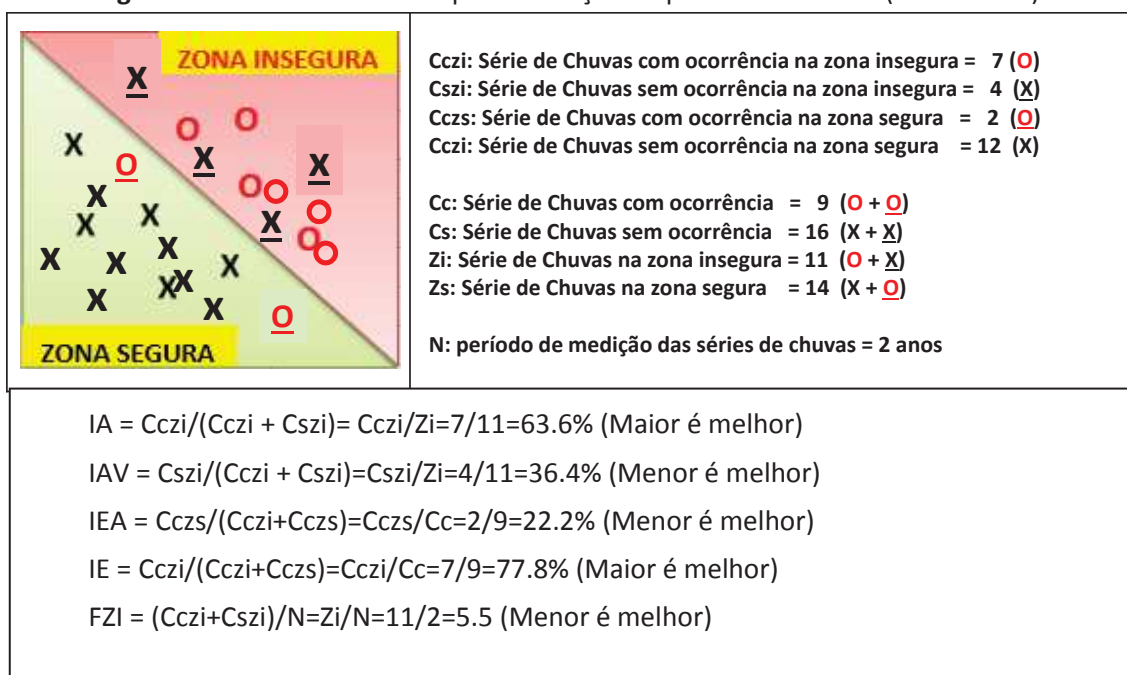
Figura 36: Modelo conceitual para avaliação da precisão do limiar (linha crítica)
