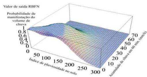
Figura 12: Ilustração de limiar tridimensional - representação em bloco Método RBFN + Método IAS
