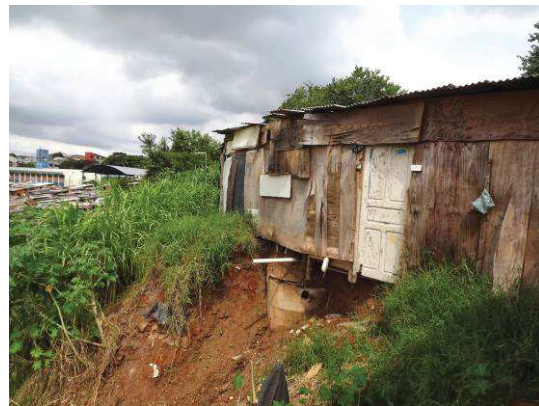
Figura F7: Vazamento de fossa em talude
