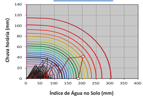
Figura 13: Ilustração de limiar tridimensional - representação em planta Método RBFN + Método IAS
