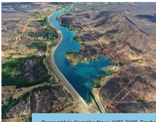
Reservatório Cacimba Nova, WBS 2109, Trecho V, Eixo Leste do PISF, Custódia/PE (nov/2024).
