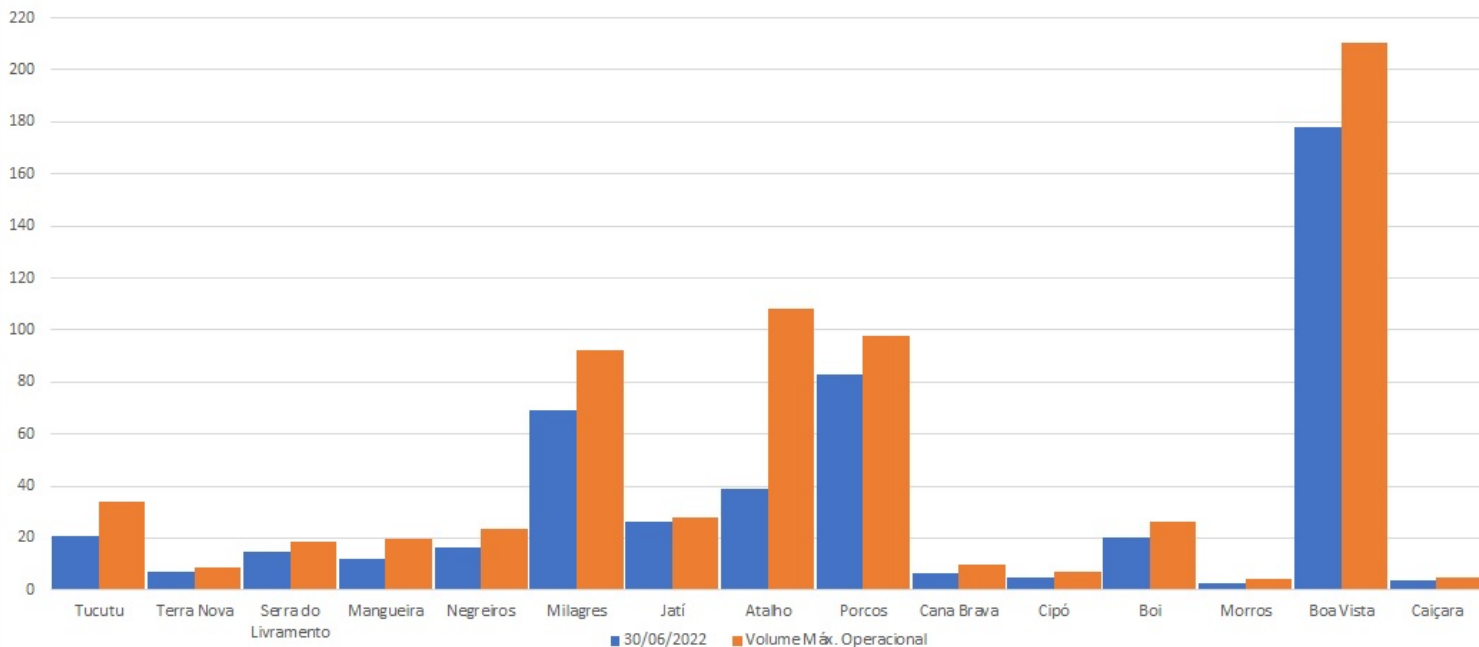
Volume dos Reservatórios Eixo Norte - milhões m 3
