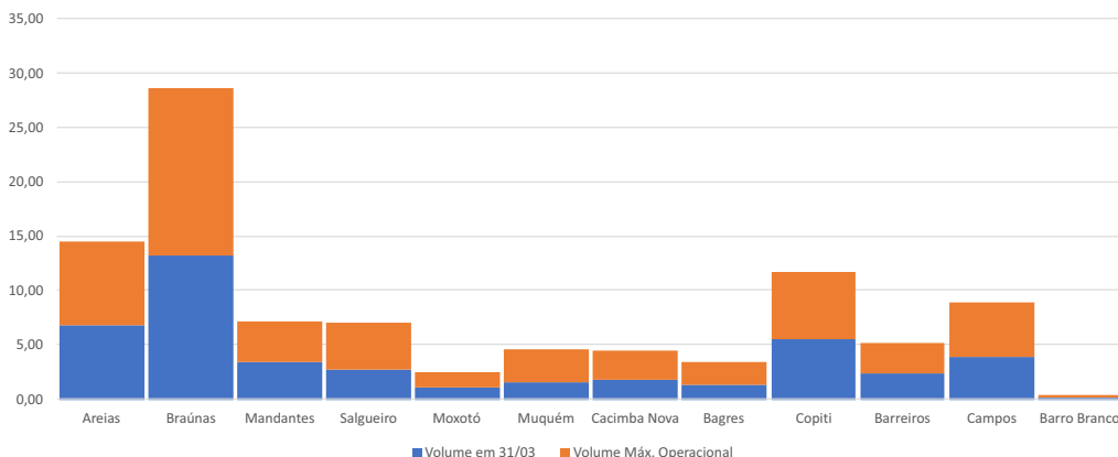
Volume dos Reservatórios Eixo Leste - milhões m 3
