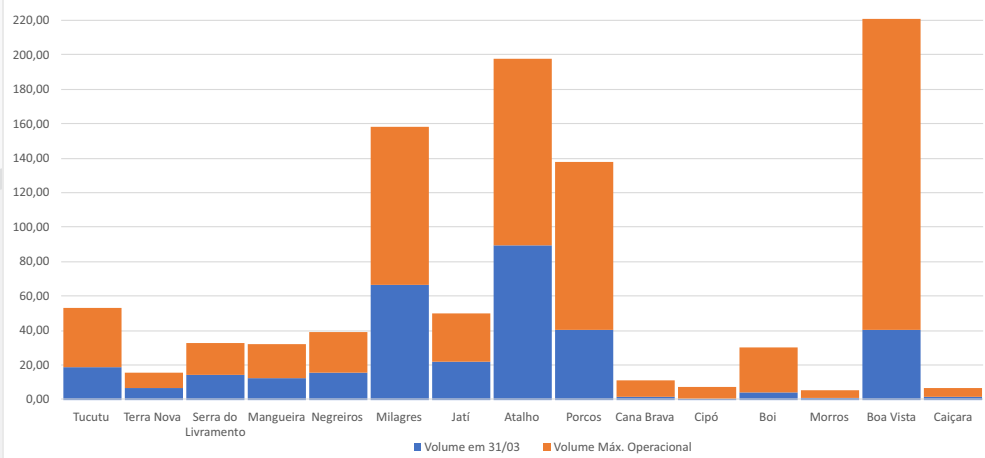
Volume dos Reservatórios Eixo Norte- milhões m³
